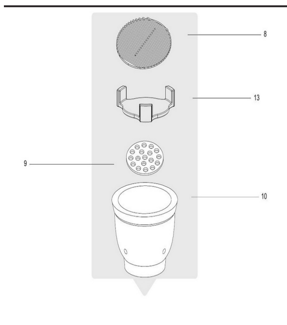
הרכבת הרכיבים הפנימיים בתוך הגוף
