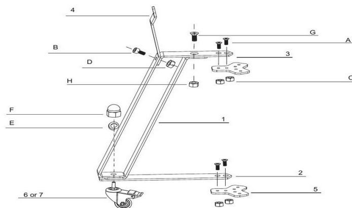
הרכבת מסגרת המעמד והגלגלים
