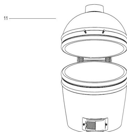
הרכבת הרכיבים הפנימיים בתוך הגוף
