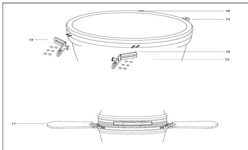
חיבור תושבות ומדפי הצד
