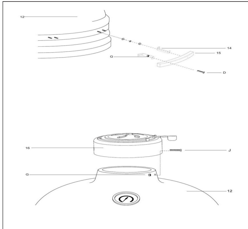
חיבור תושבת מדף הצד והתקנת המדחום
