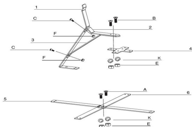
הרכבת מסגרת העגלה
