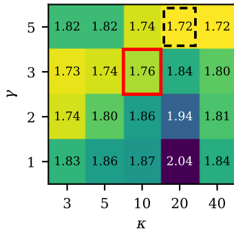
EuroSAT
