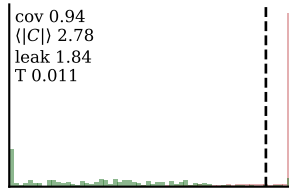
EuroSAT
