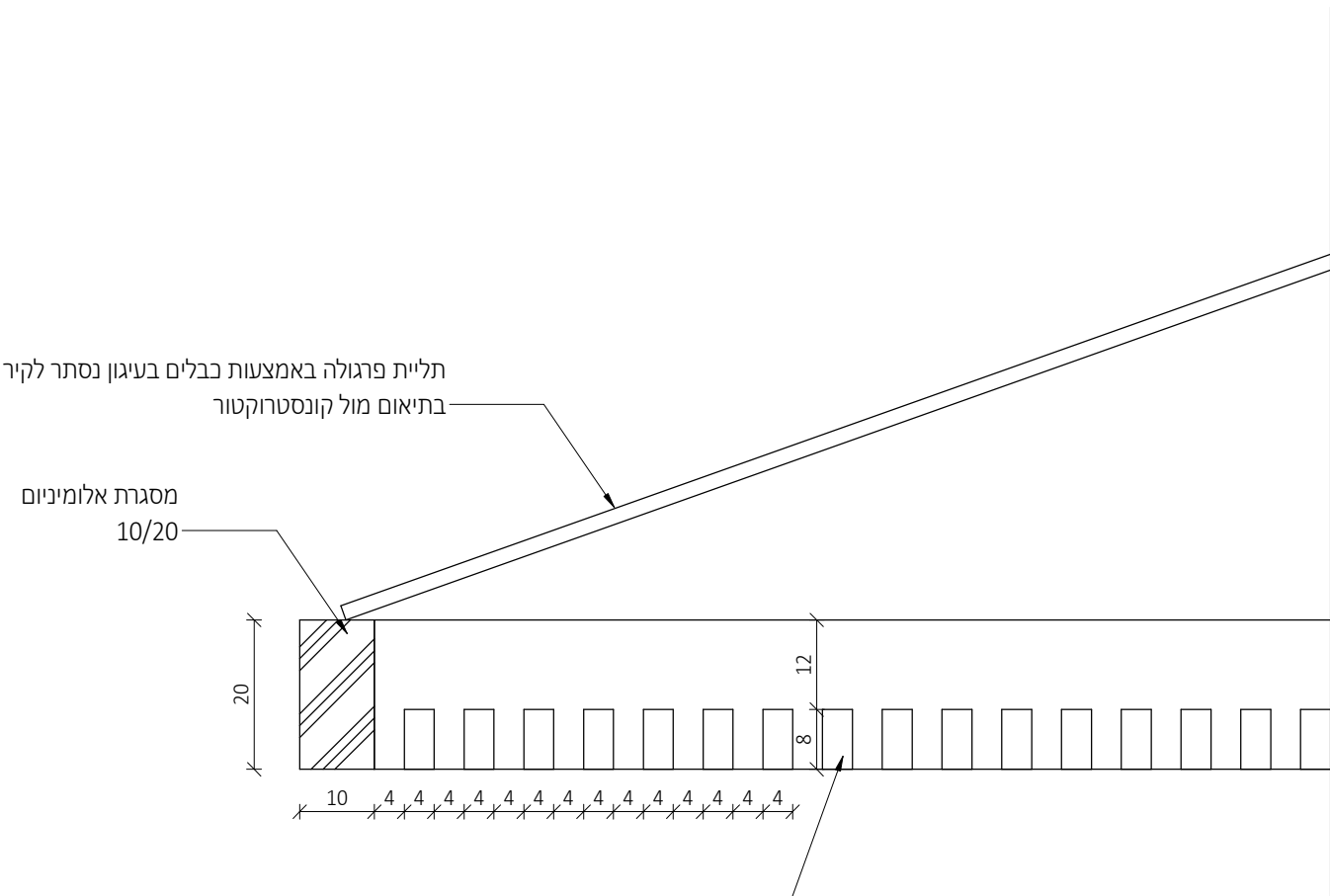
פרגולה - חתך רוחב
