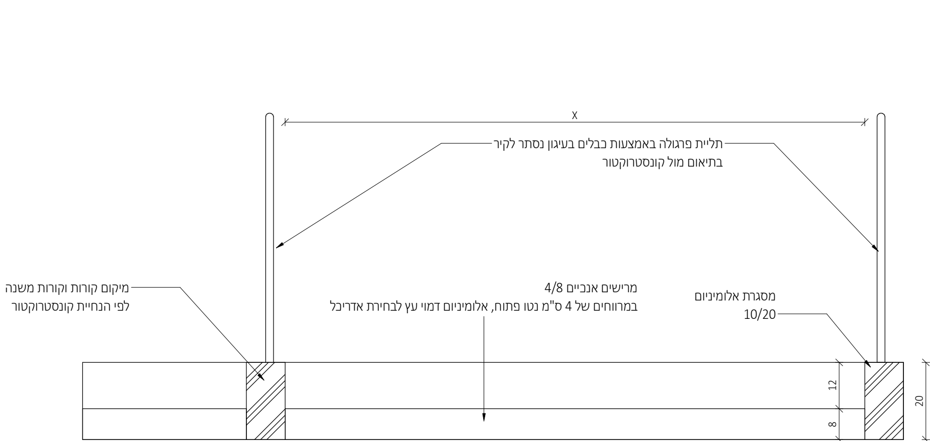
פרגולה - חתך אורך
