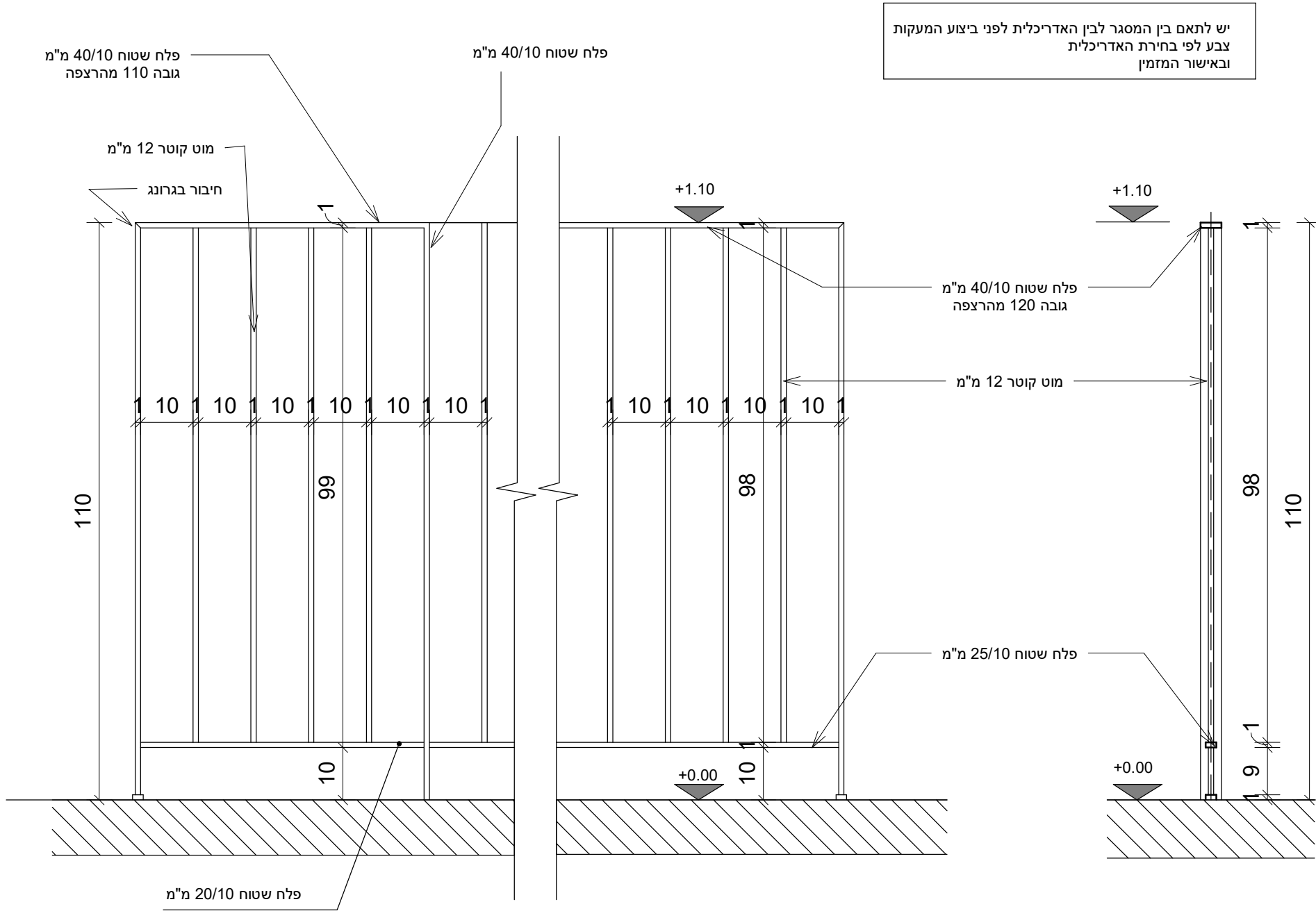
מעקה אנכי
