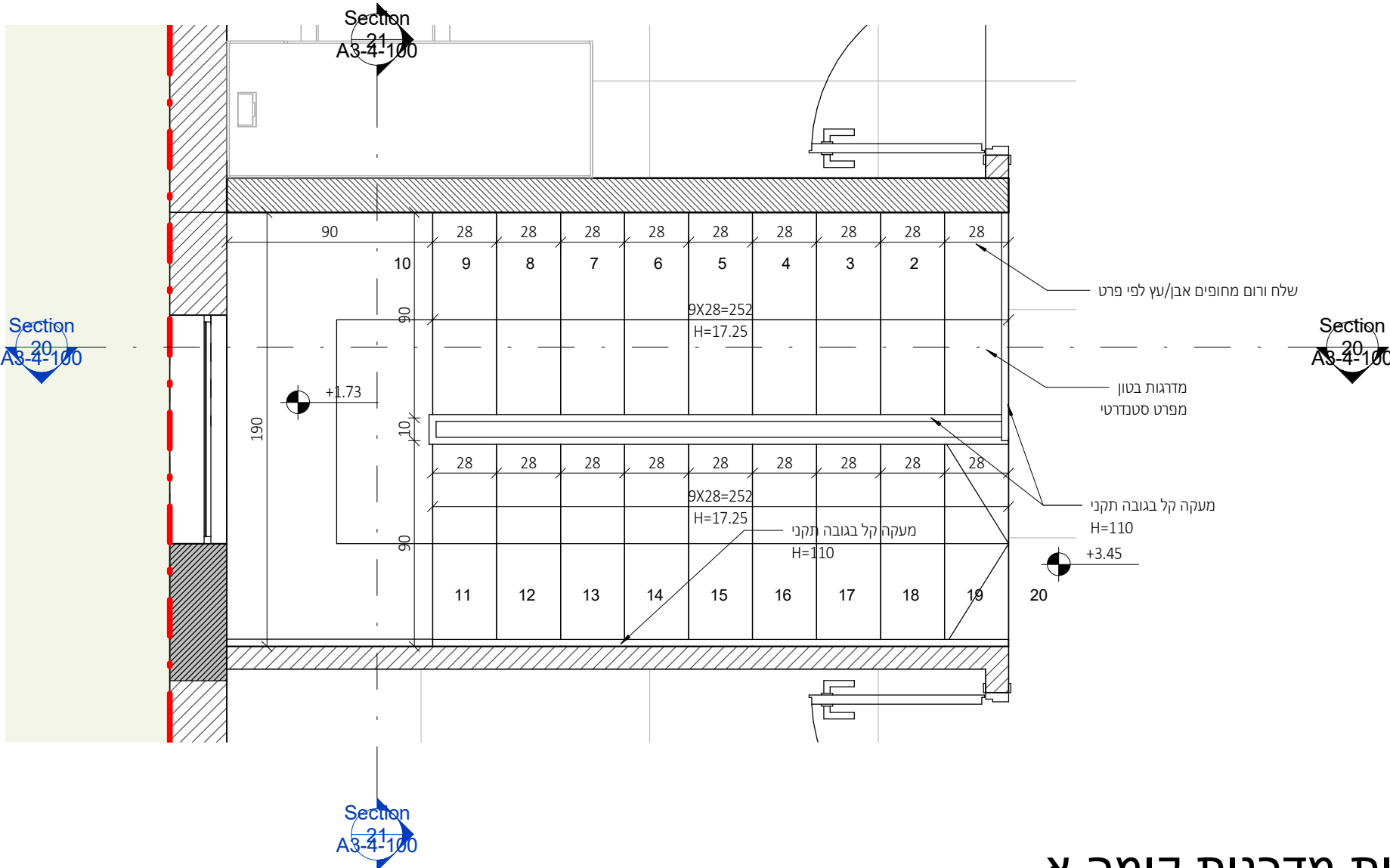
תכנית מדרגות קומה א
