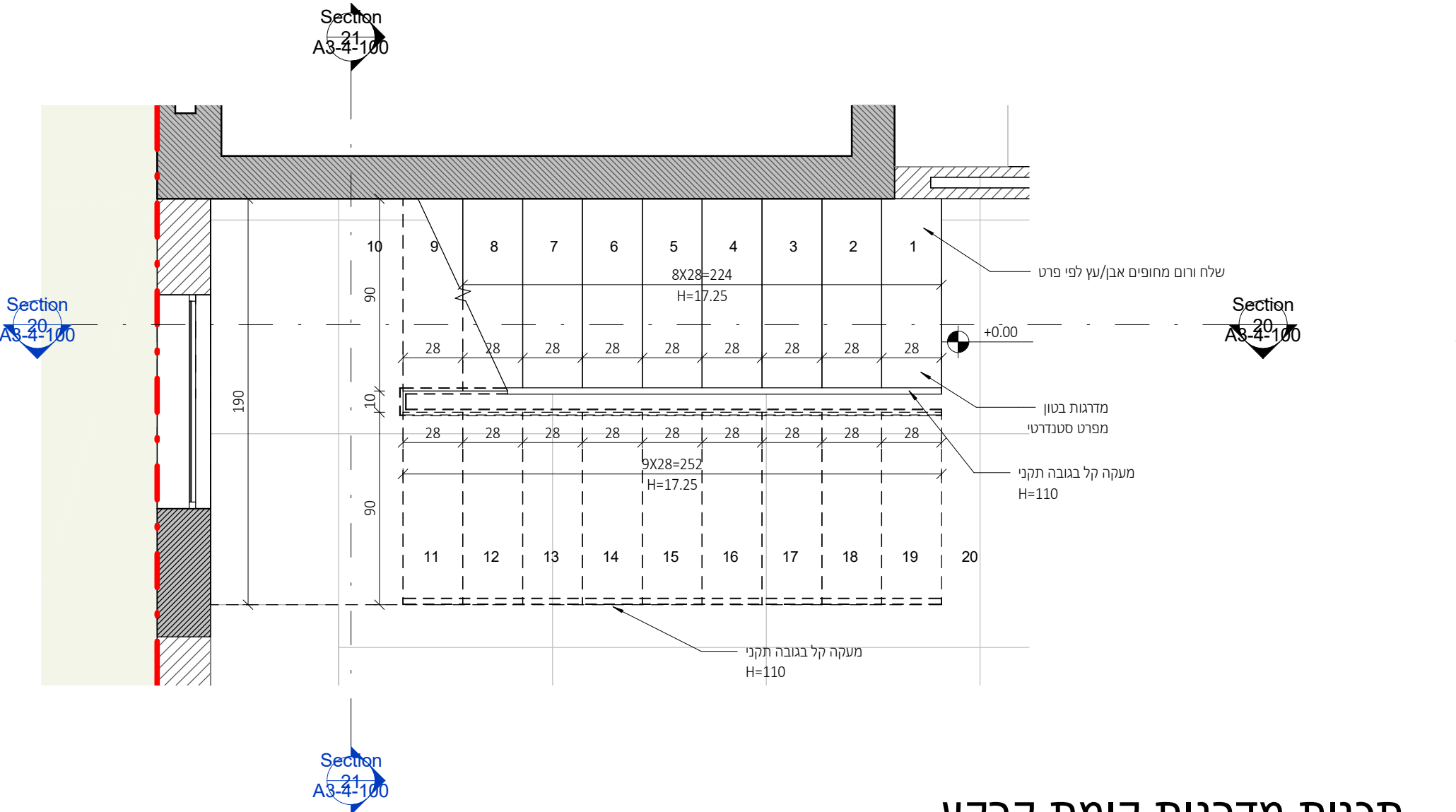
תכנית מדרגות קומת קרקע
