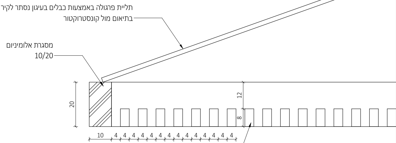
פרגולה - חתך רוחב
