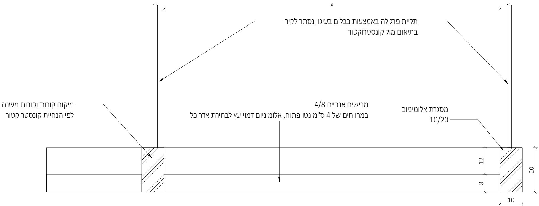
פרגולה - חתך אורך
