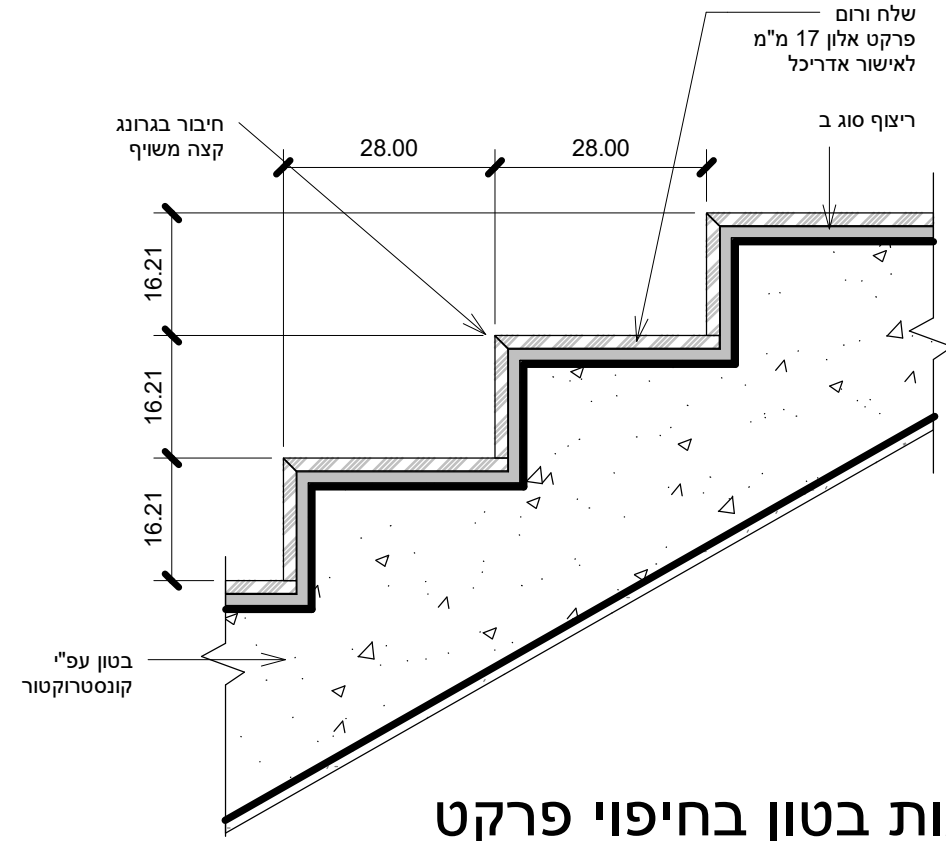
פרט מדרגות בטון בחיפוי פרקט
