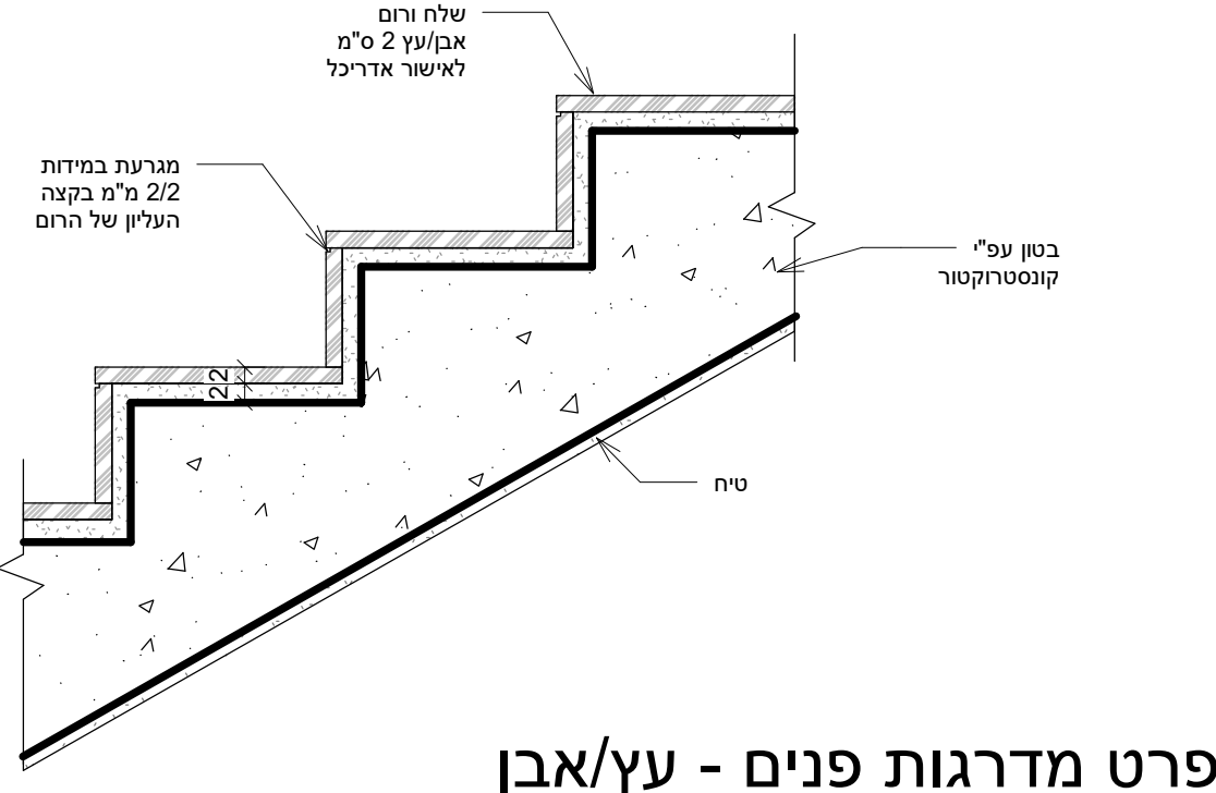
פרט מדרגות פנים - עץ/אבן
