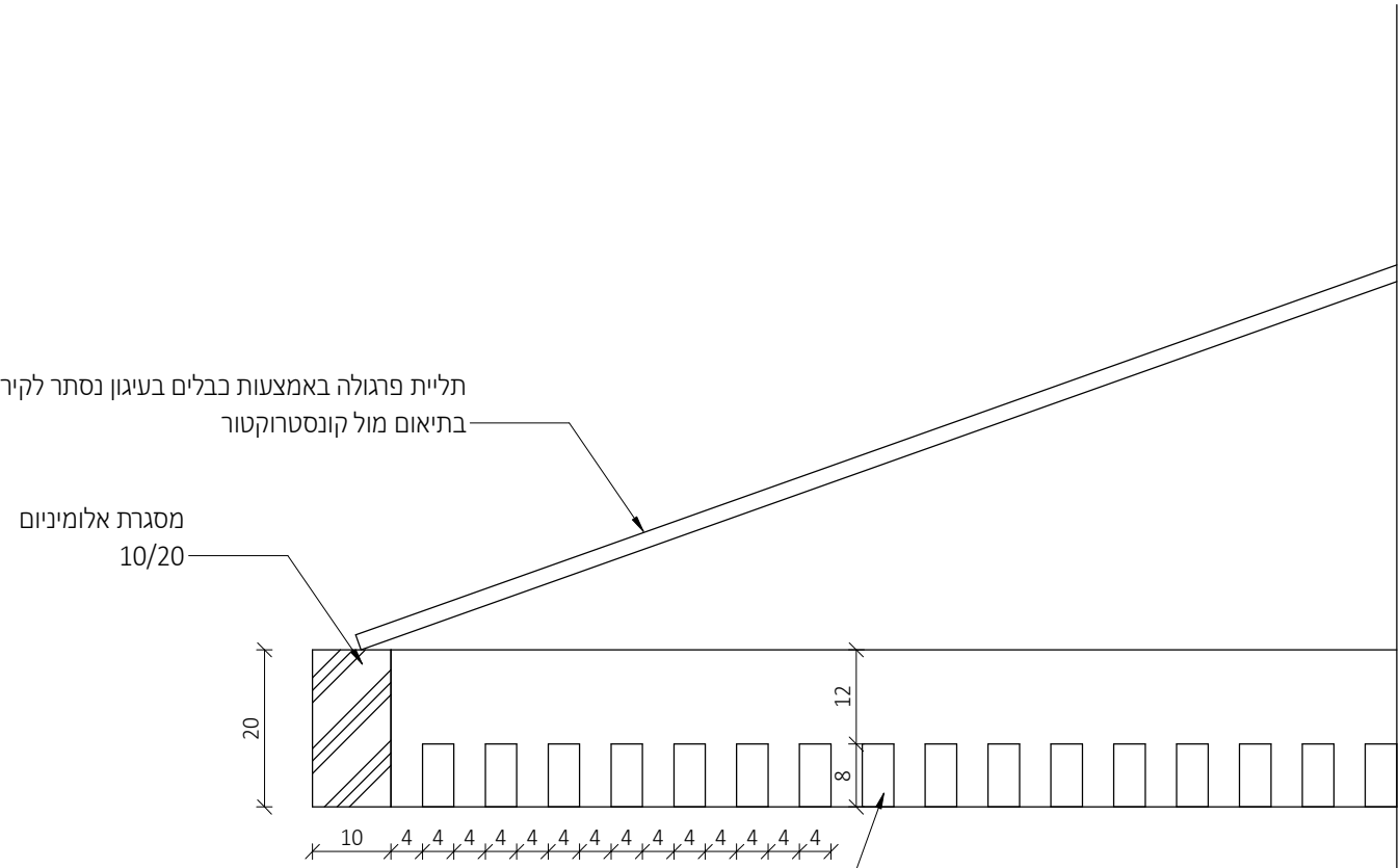
פרגולה - חתך רוחב
