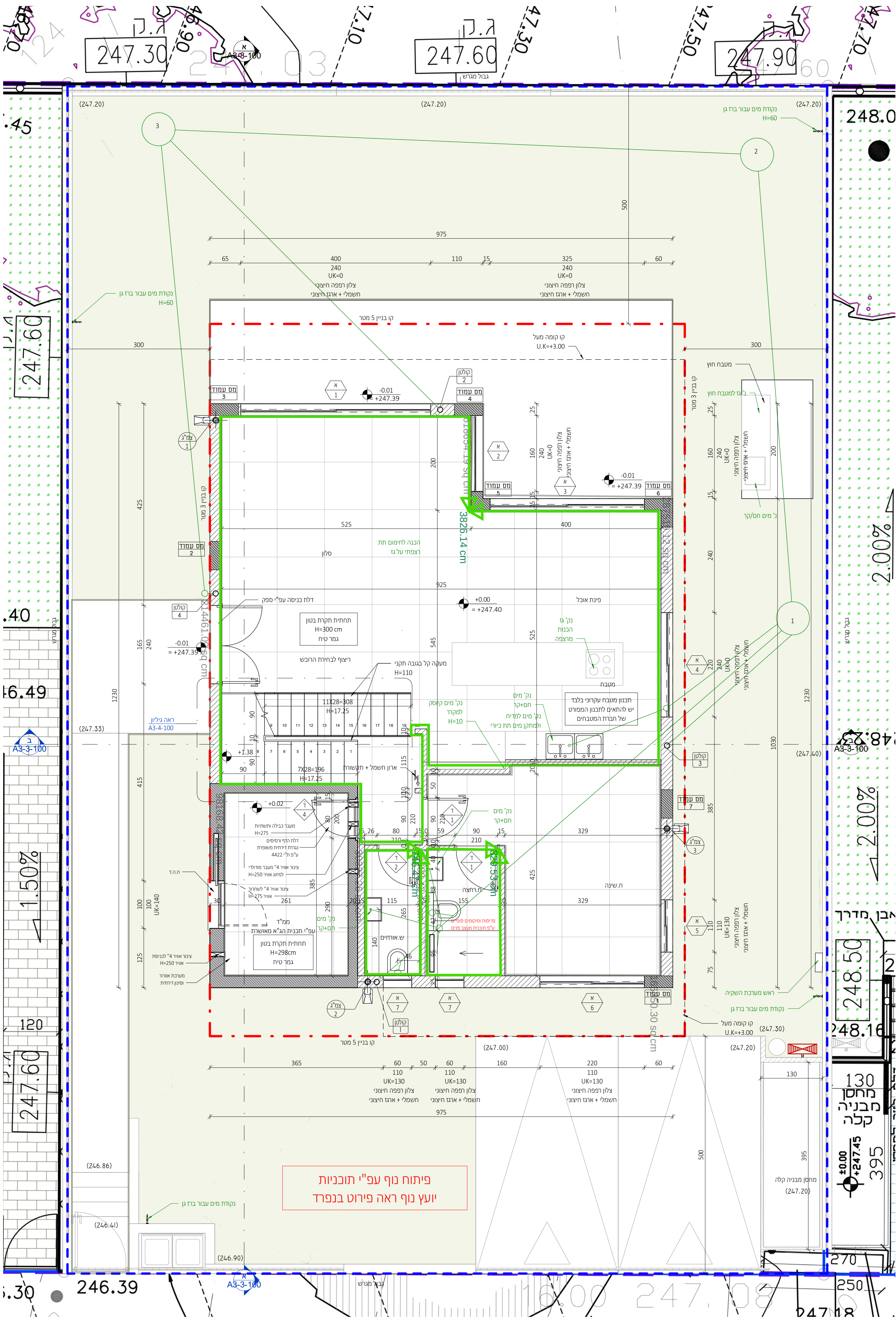
תכנית קומת קרקע
