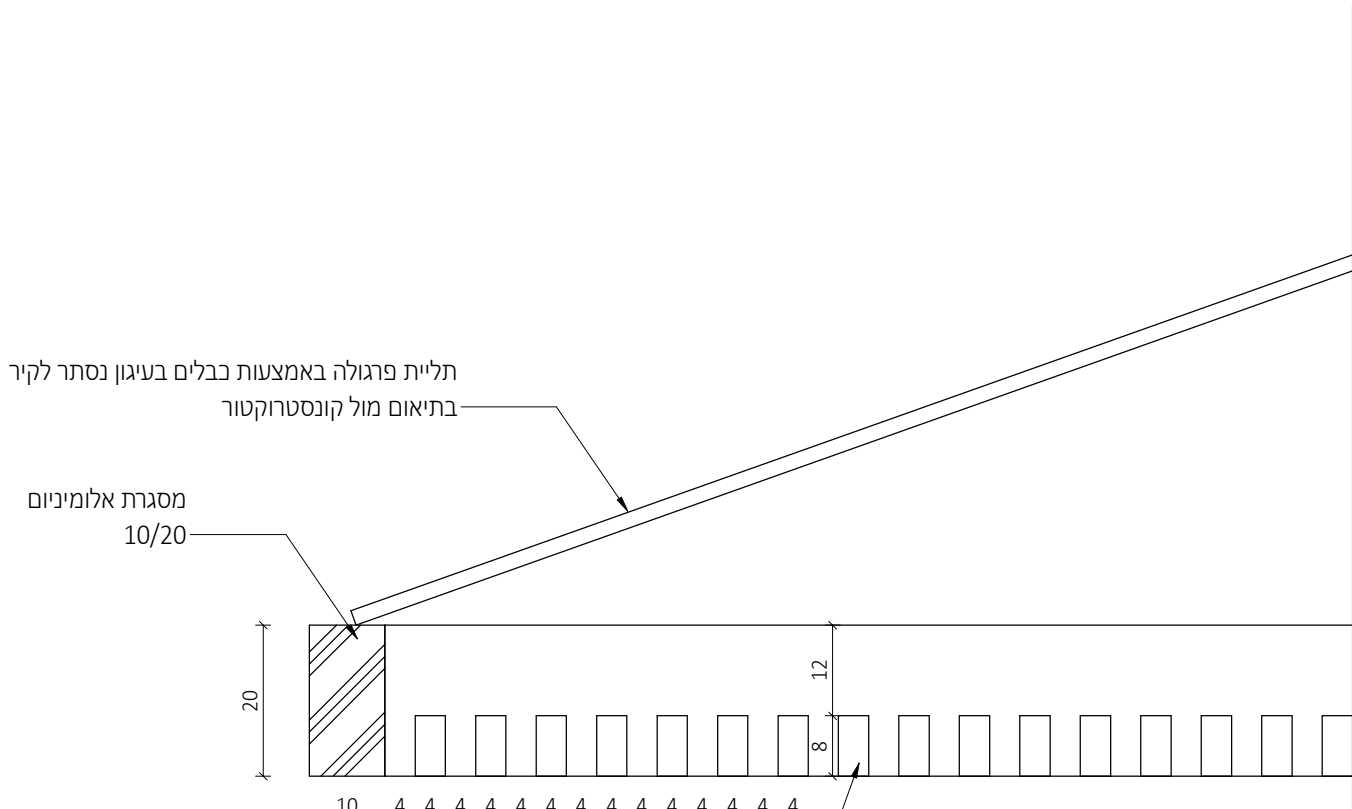
פרגולה - חתך רוחב
