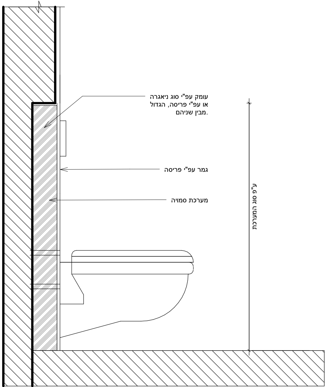
פרט 5 - אסלה תלויה בקיר 20 1 : 10
