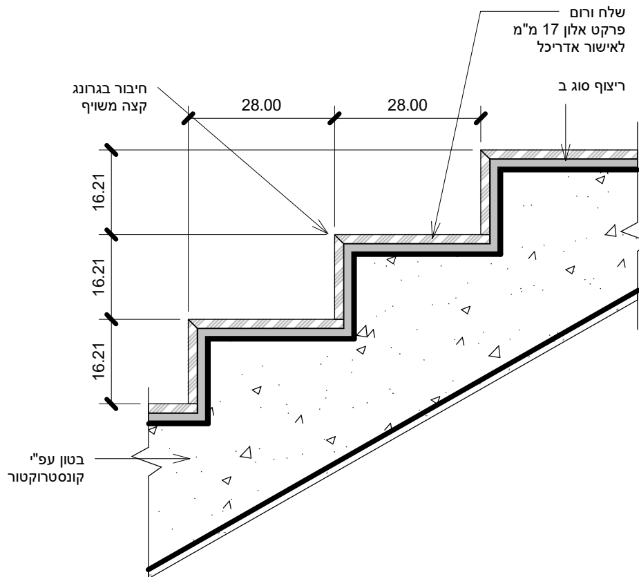
פרט מדרגות בטון בחיפוי פרקט
