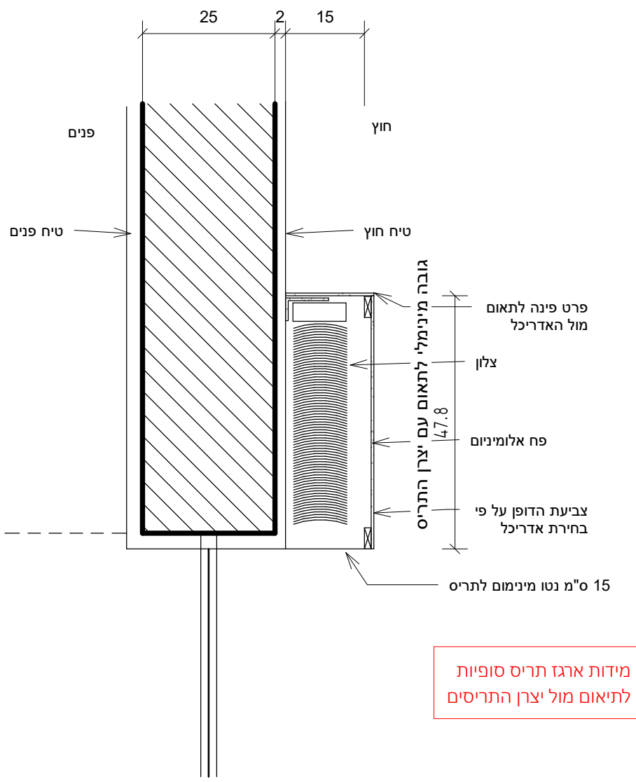
פרט 1 - כיס צלון חיצוני
