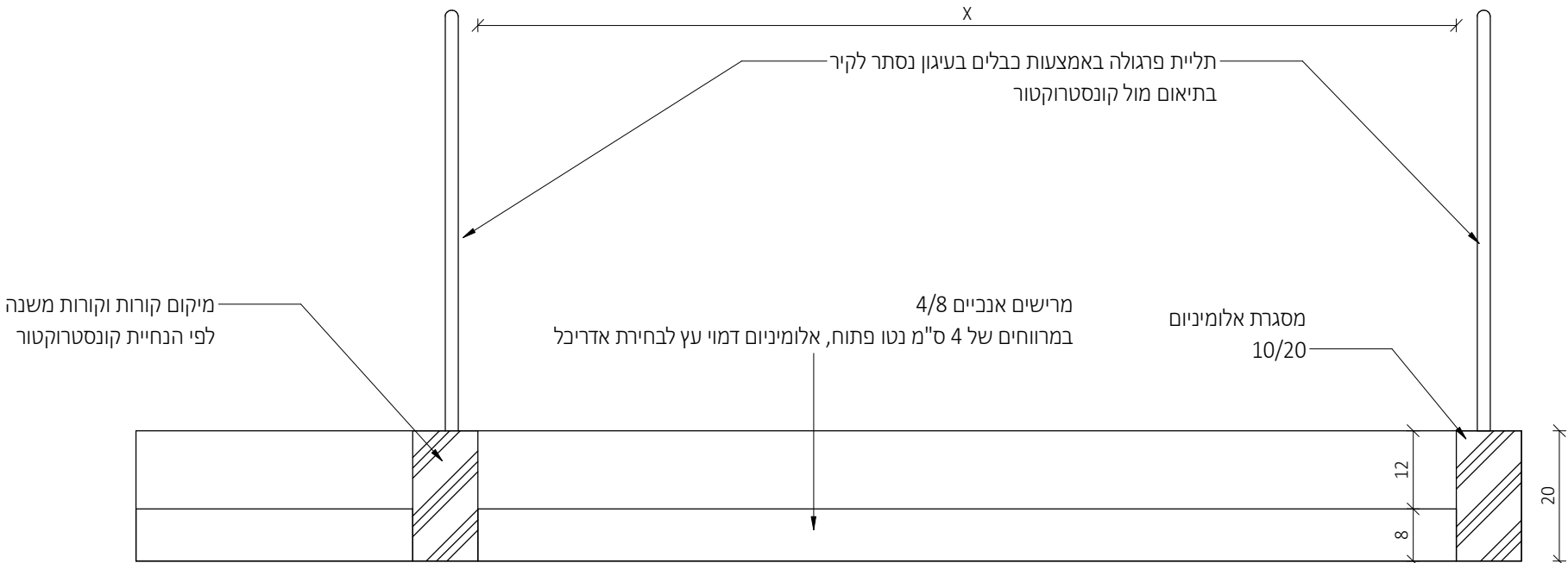
פרגולה - חתך אורך
