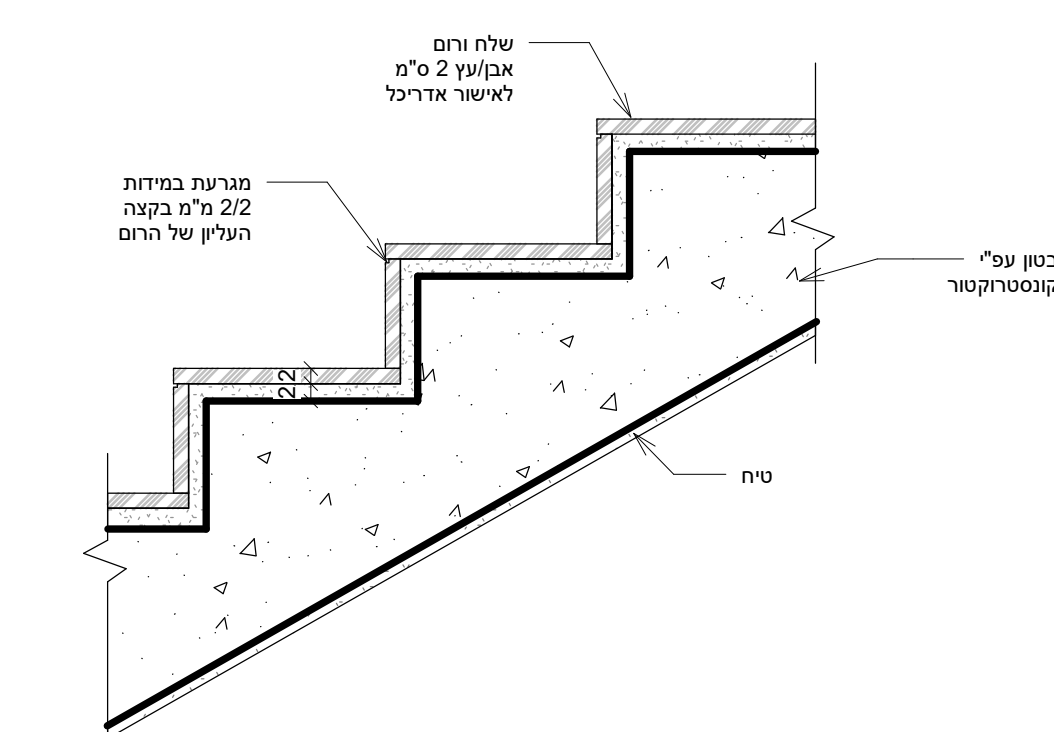
פרט מדרגות פנים - עץ/אבן
