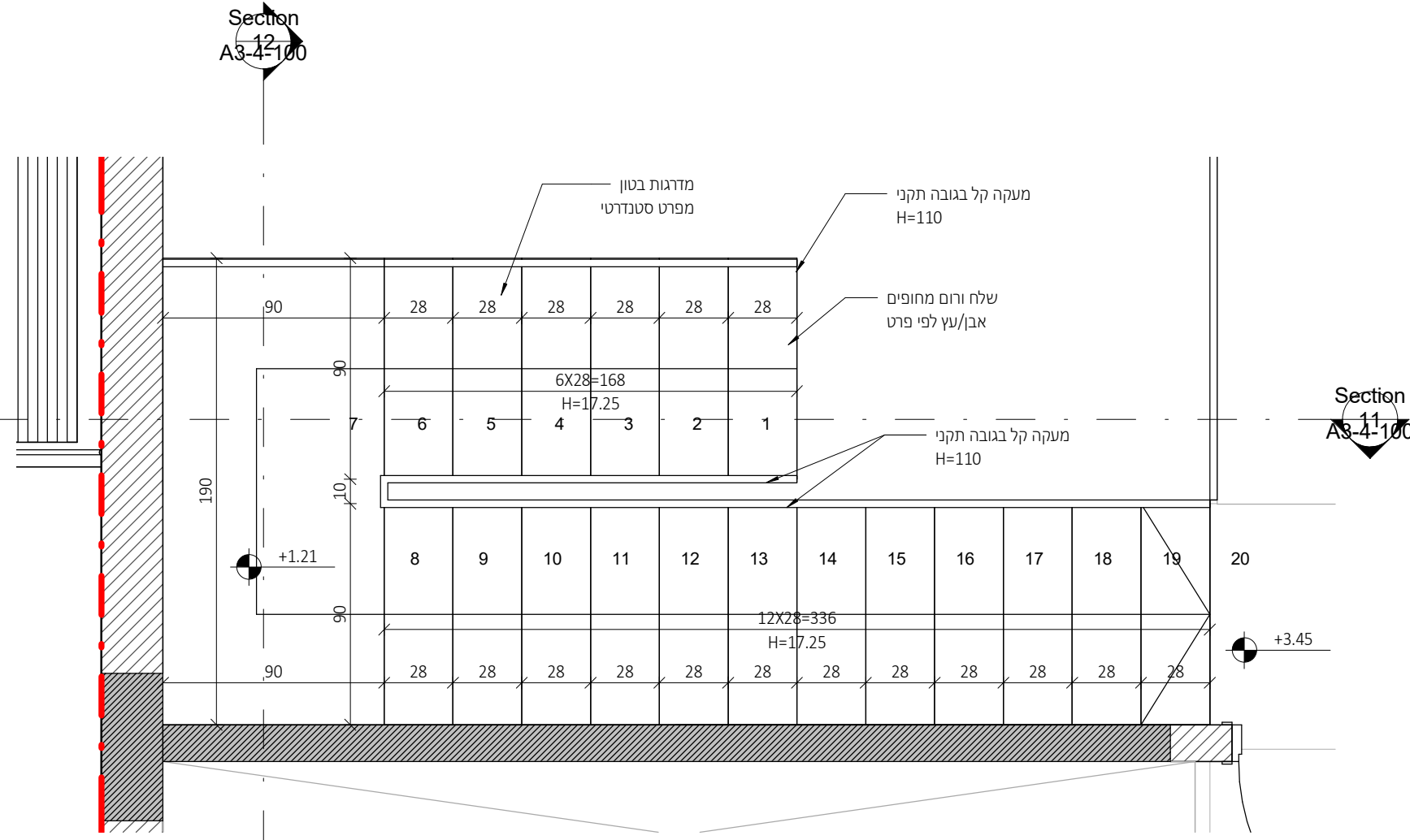
תכנית מדרגות קומה א
