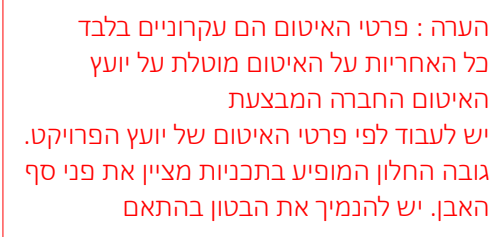
פרט עקרוני בלבד - פרט סופי מספק החלונות
