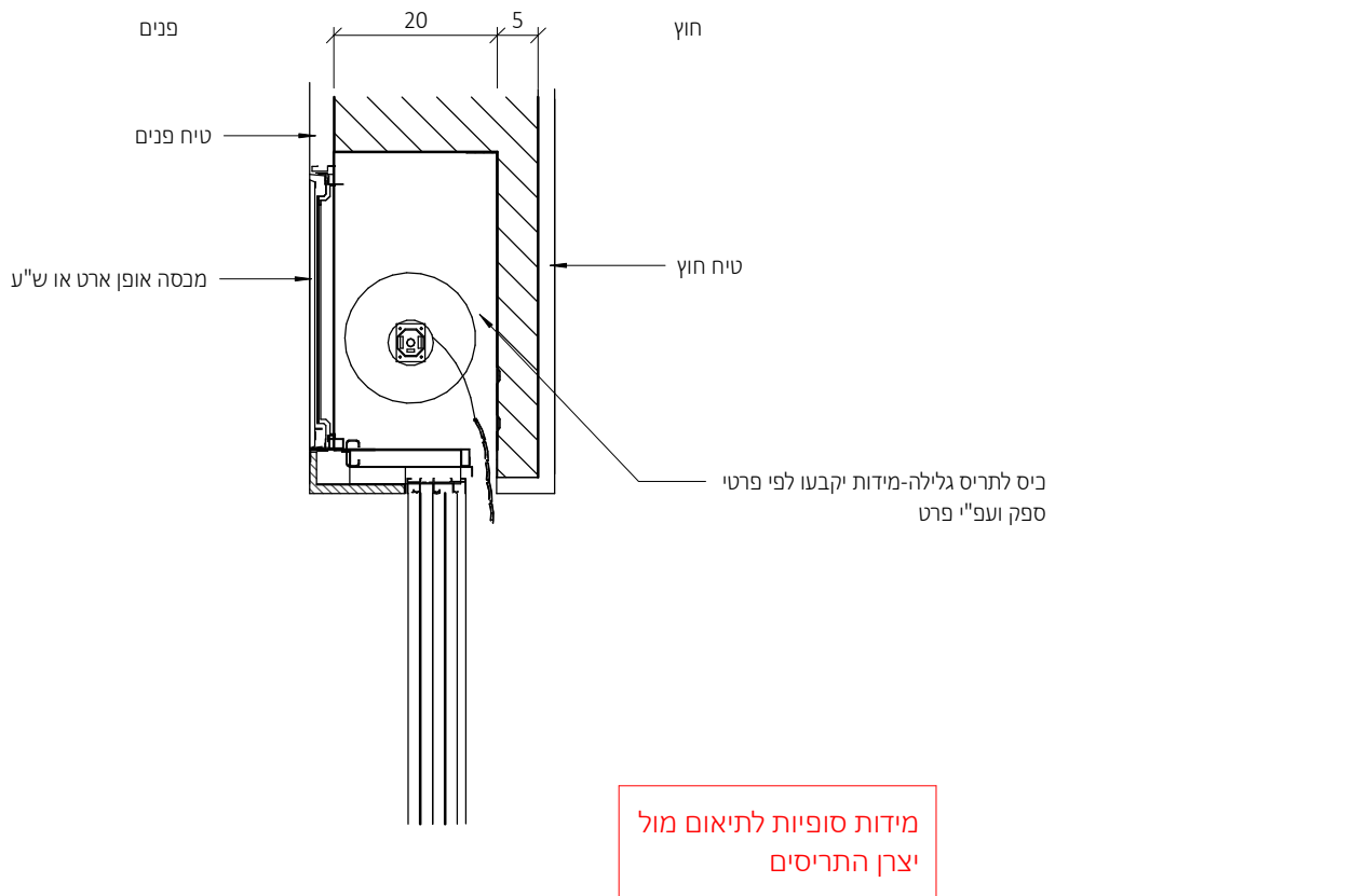
פרט 2 - תריס גלילה 1 : 10
