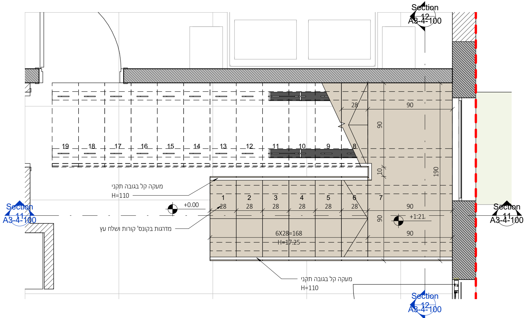
1 : 25
