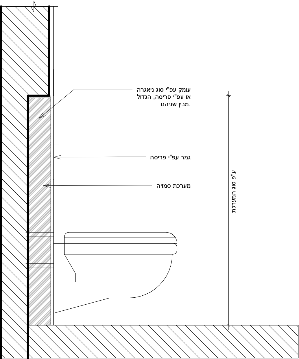
פרט 5 - אסלה תלויה בקיר 20 1 : 10
