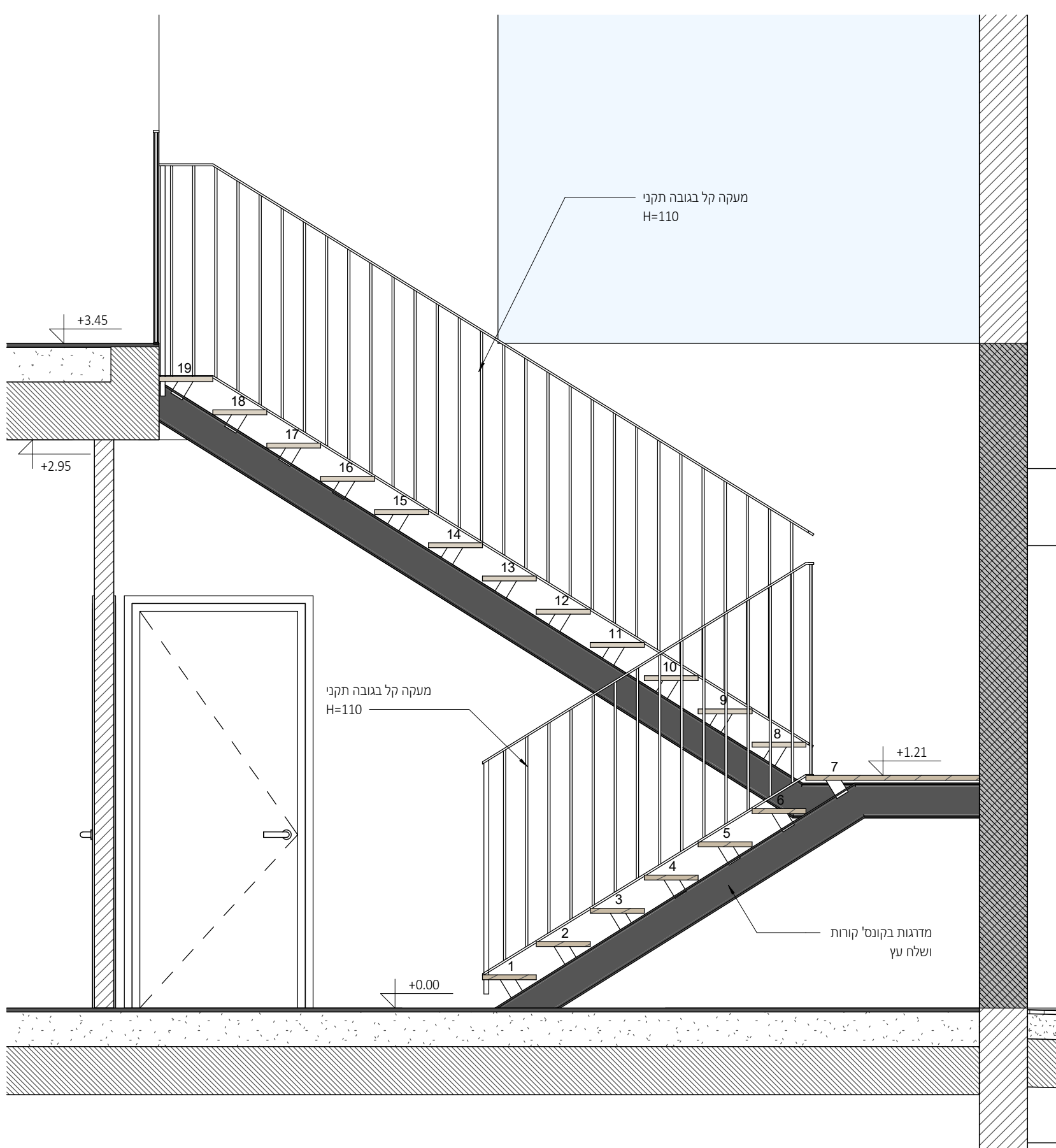
1 : 25
