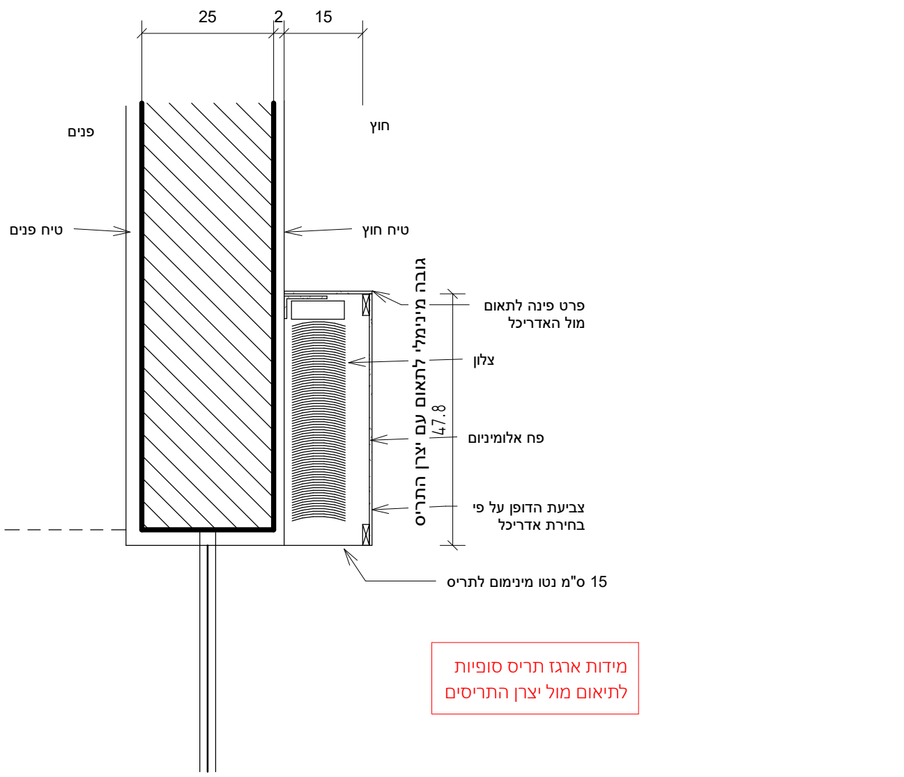
פרט 1 - כיס צלון חיצוני
