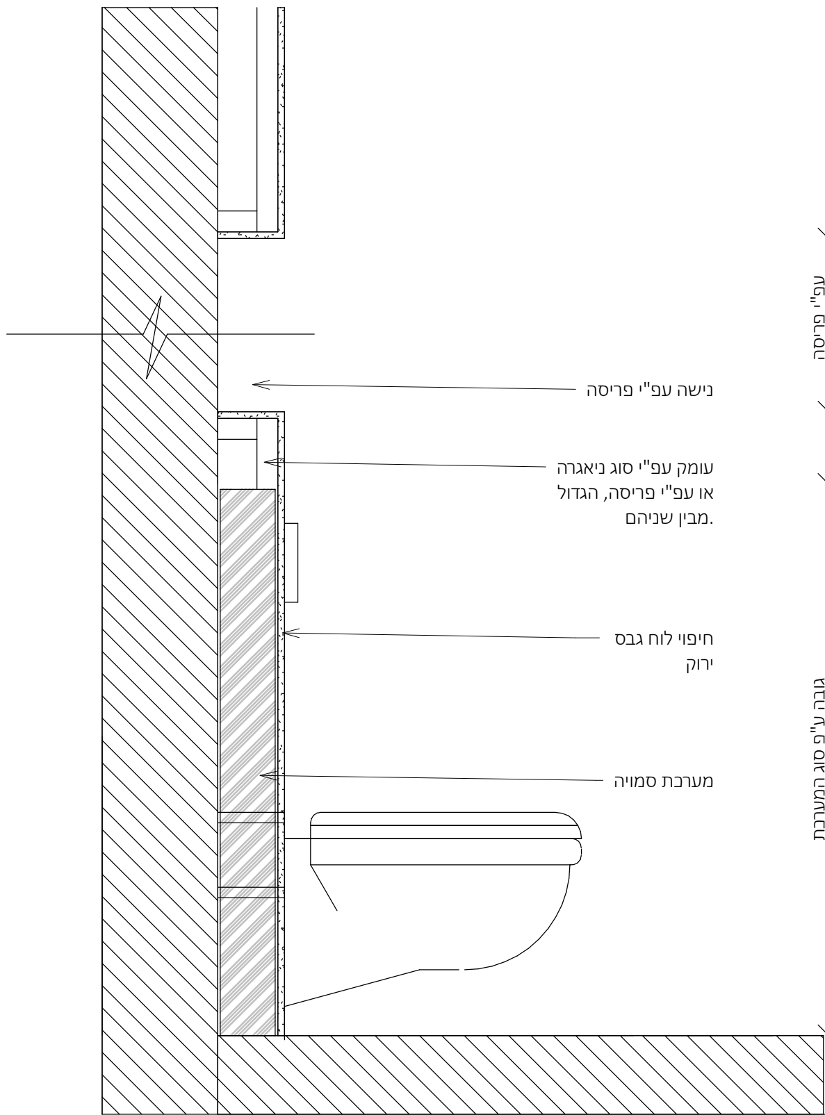
פרט 6 -אסלה תלויה מנגנון סמוי בעיבוי גבס
