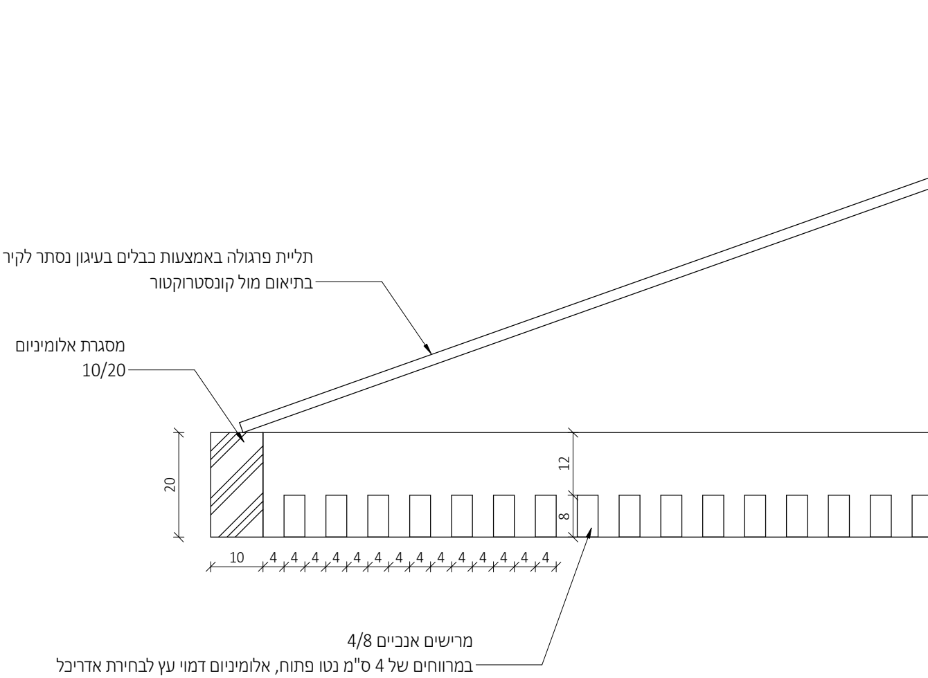
פרגולה - חתך רוחב
