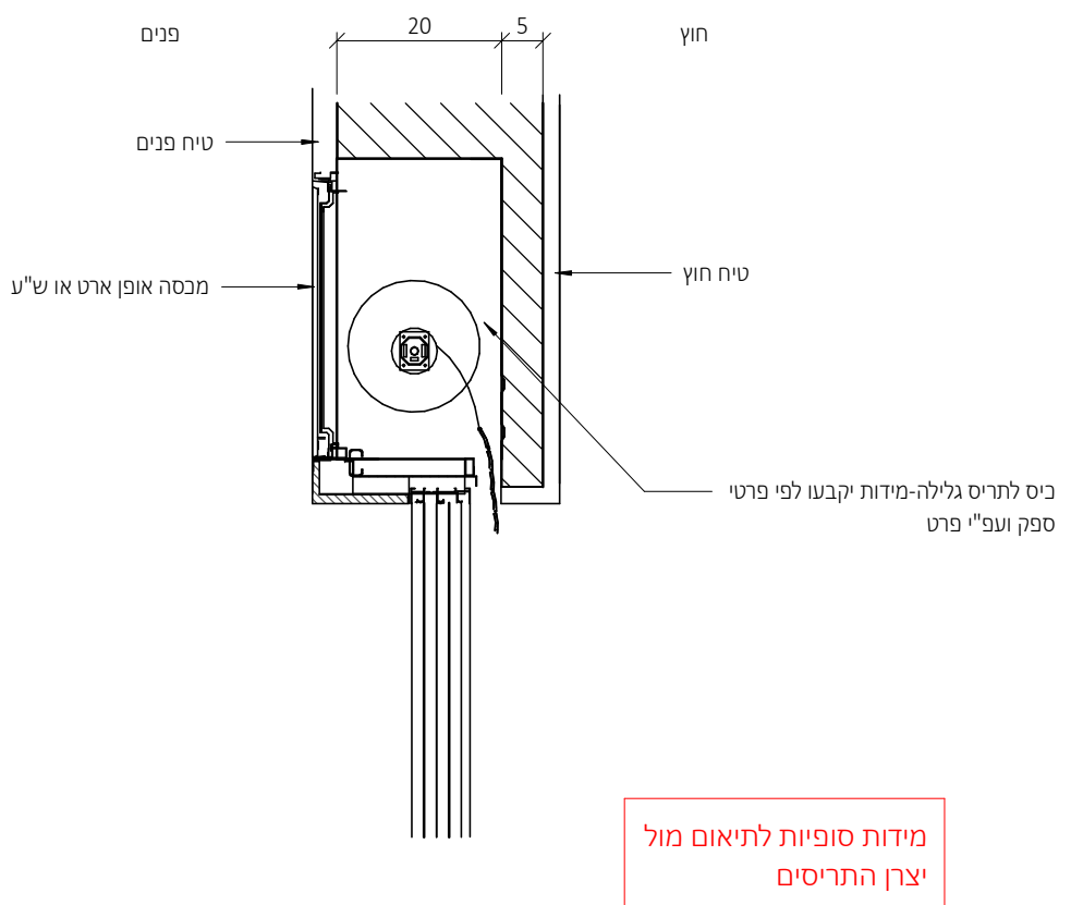
פרט 2 - תריס גלילה 1 : 10
