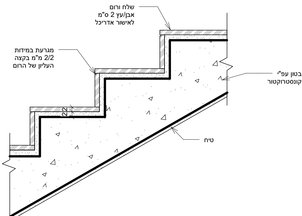
פרט מדרגות פנים - עץ/אבן
