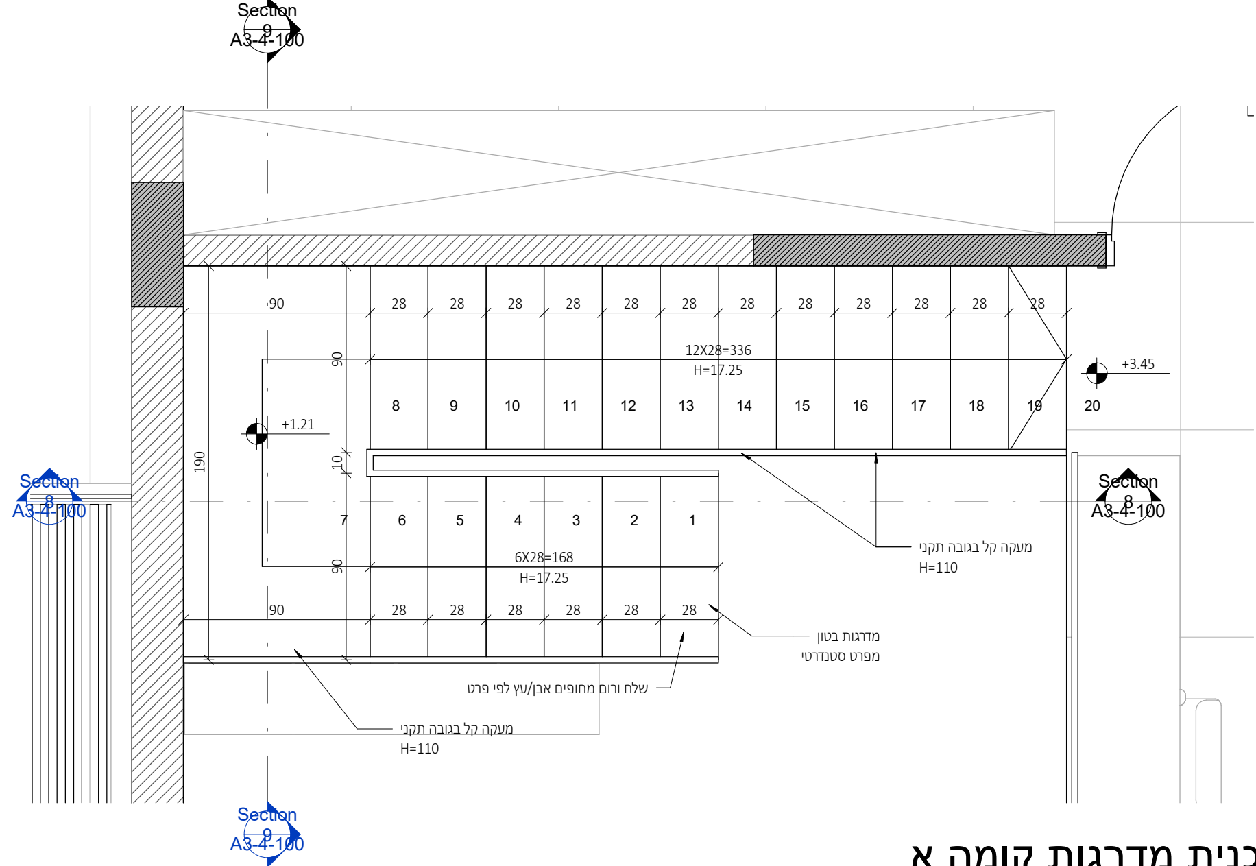
תכנית מדרגות קומה א
