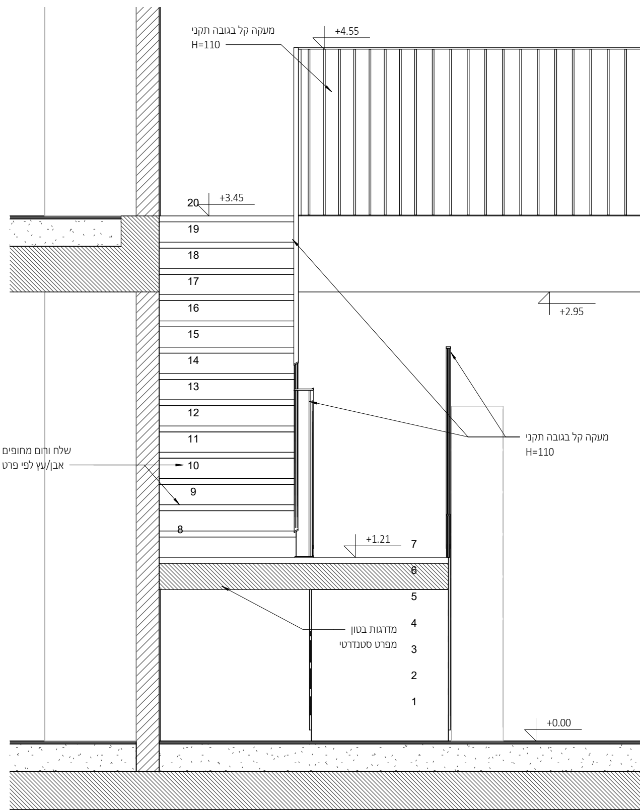
פרט מדרגות בטון בחיפוי פרקט
