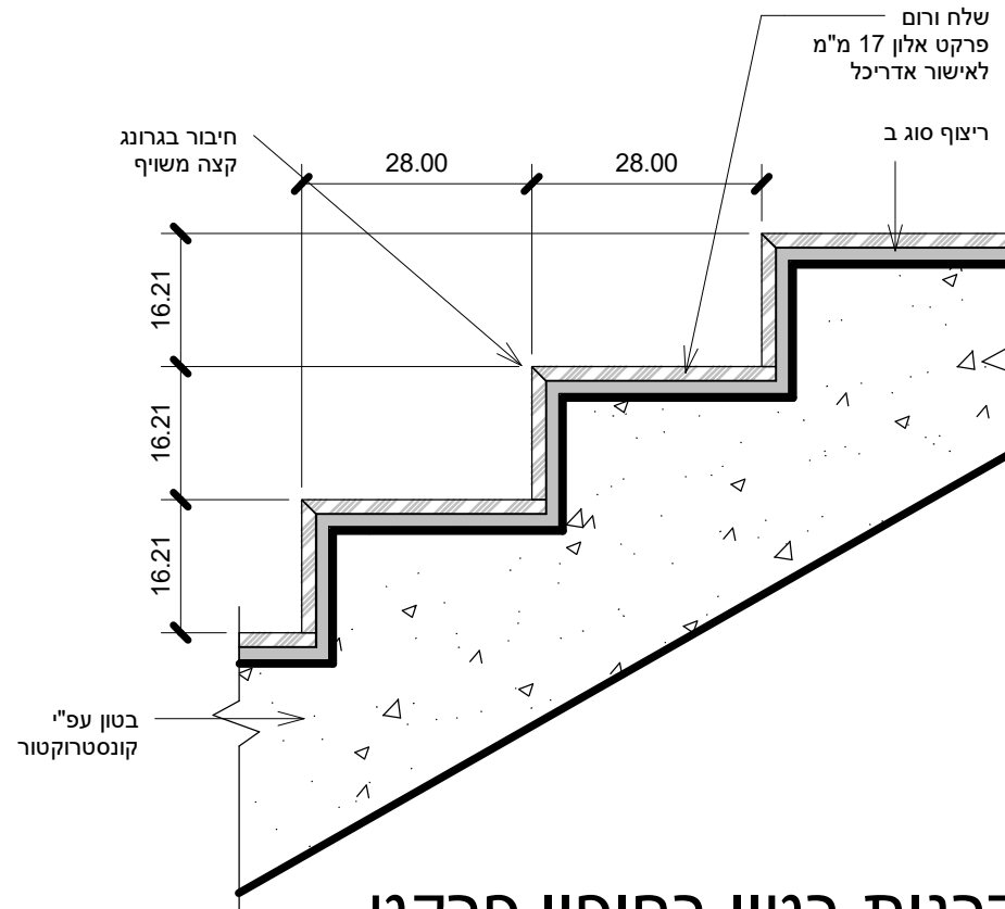
פרט מדרגות בטון בחיפוי פרקט
