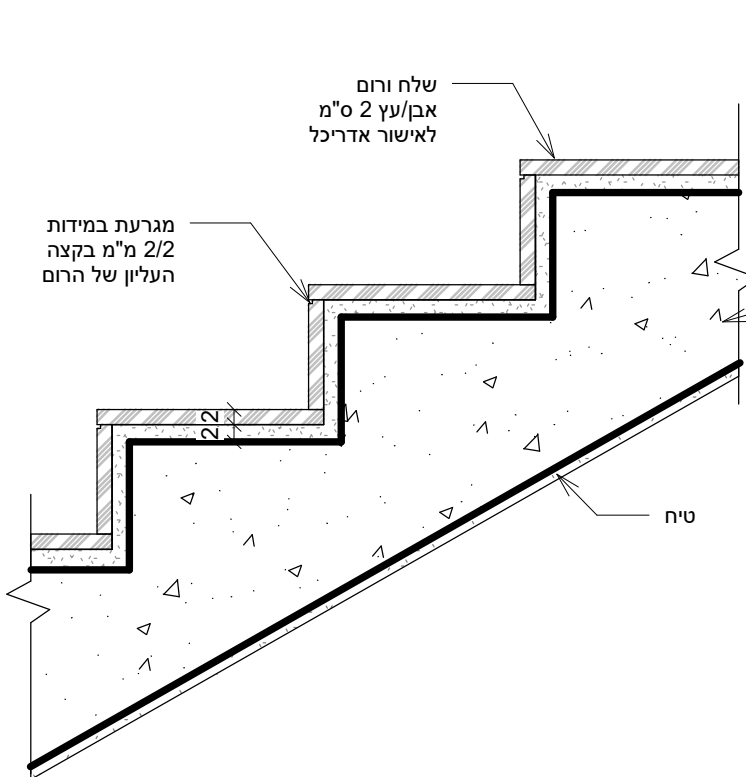
פרט מדרגות פנים - עץ/אבן
