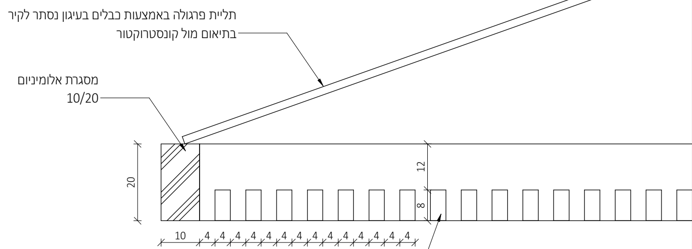
פרגולה - חתך רוחב
