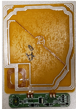
ANT Module(Back)
