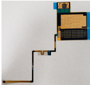
ANT Module(Back)
