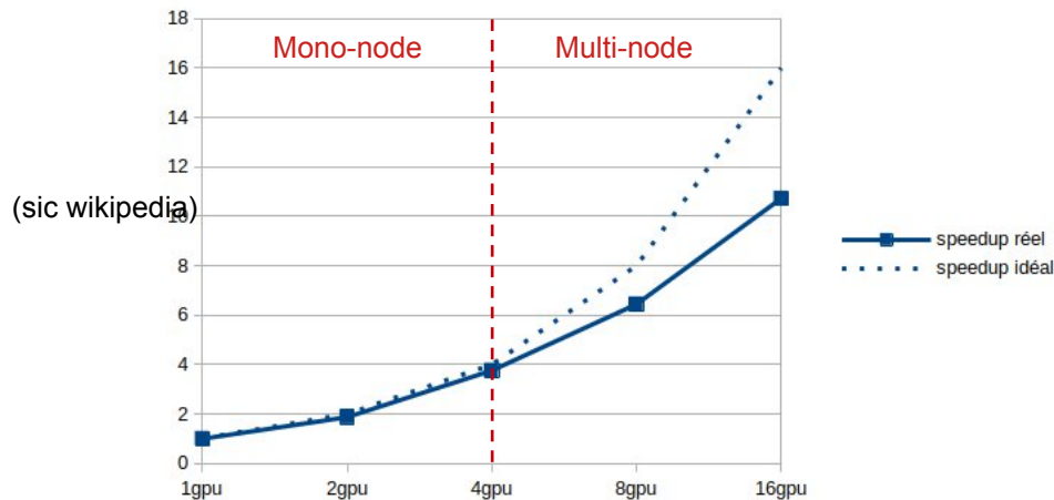
Flaubert benchmark
