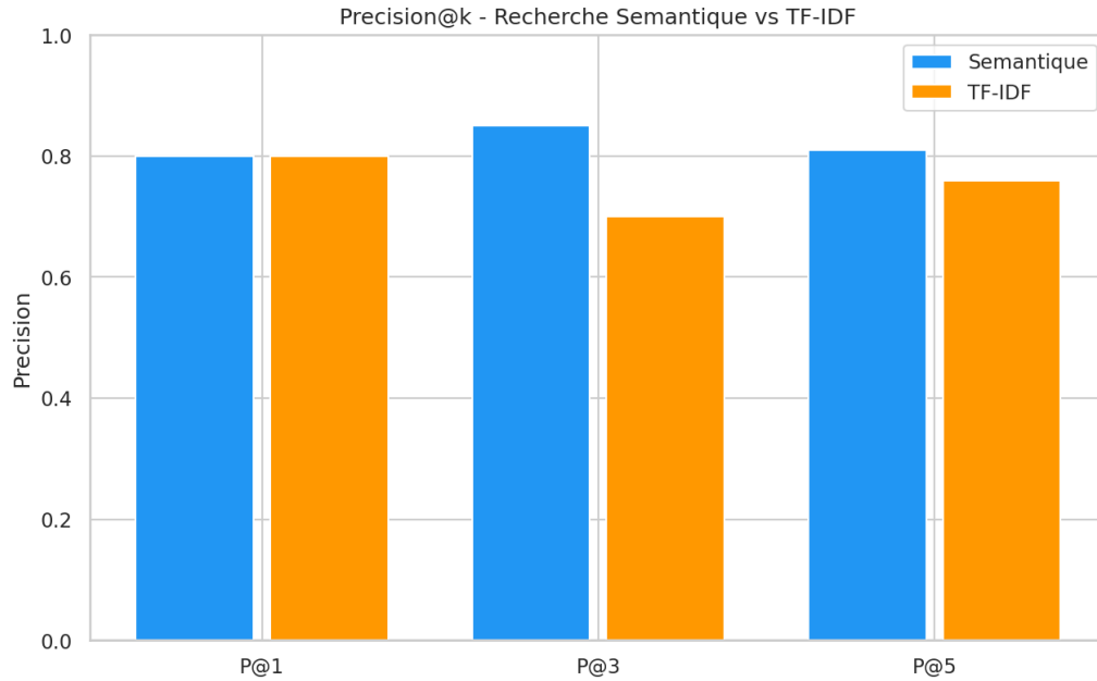
Figure 1: Comparaison de Precision@k entre recherche sémantique et TF-IDF
