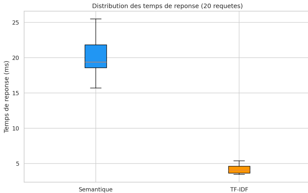
Figure 2: Distribution des temps de réponse
