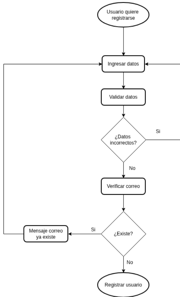
Figura 1: Diagrama de flujo registrar a un usuario
