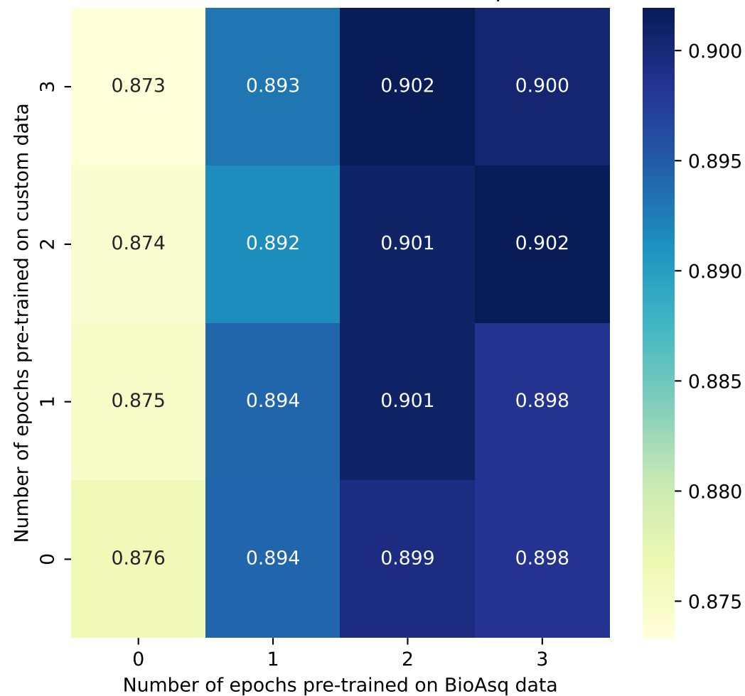
Berstscore F1 Score Heatmap
