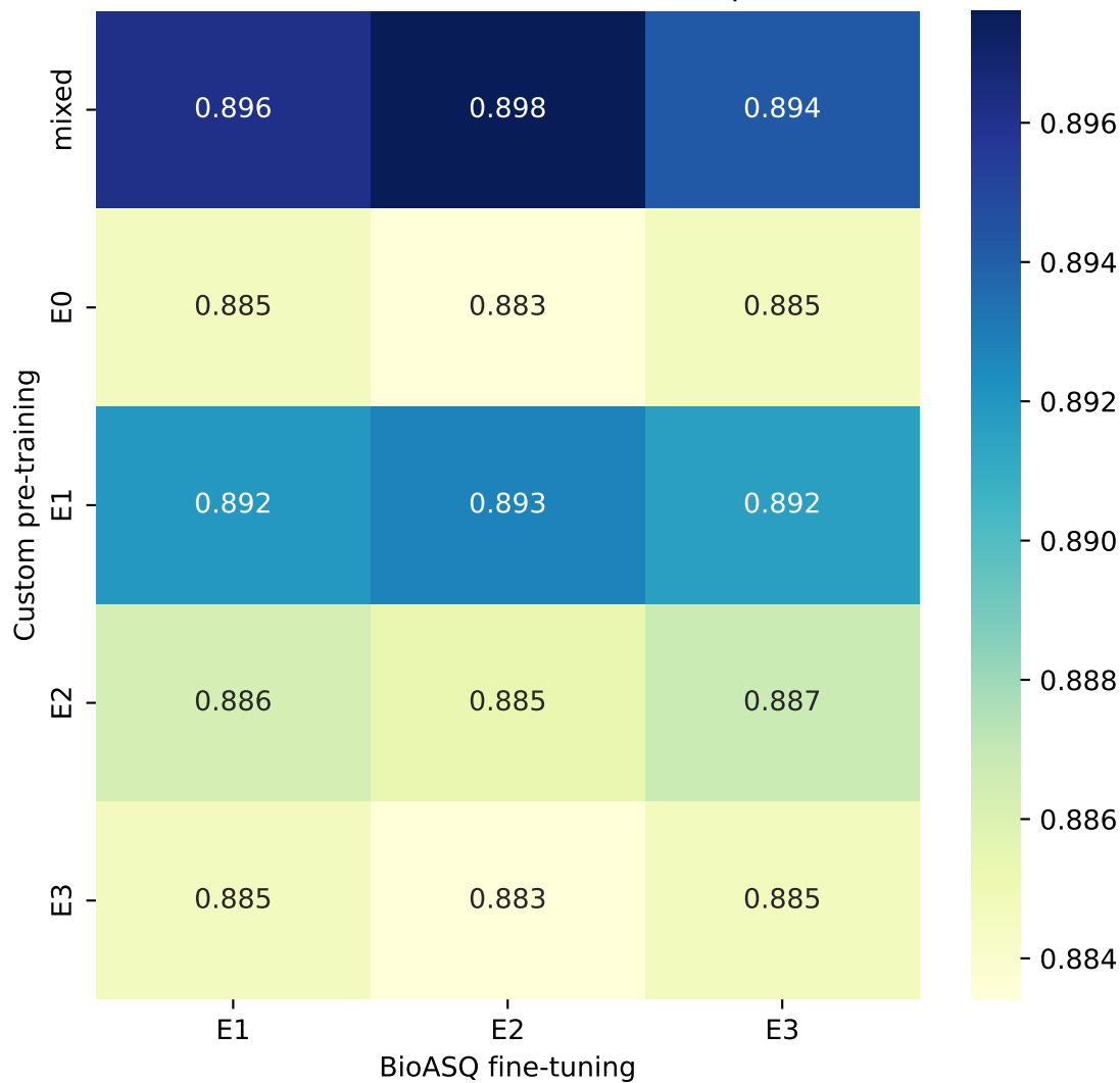
BERTScore F1 Score Heatmap
