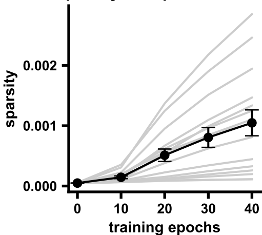
Sparsity vs. Epoch. NO PCA
