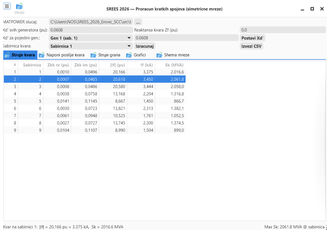
Slika 2: Grafički interfejs: nivoi kvara po sabirnicama (test mreža case9).
