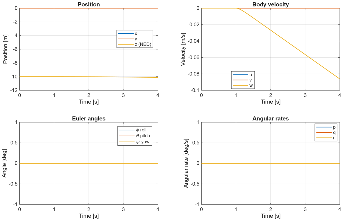
Реакція вертикального каналу
