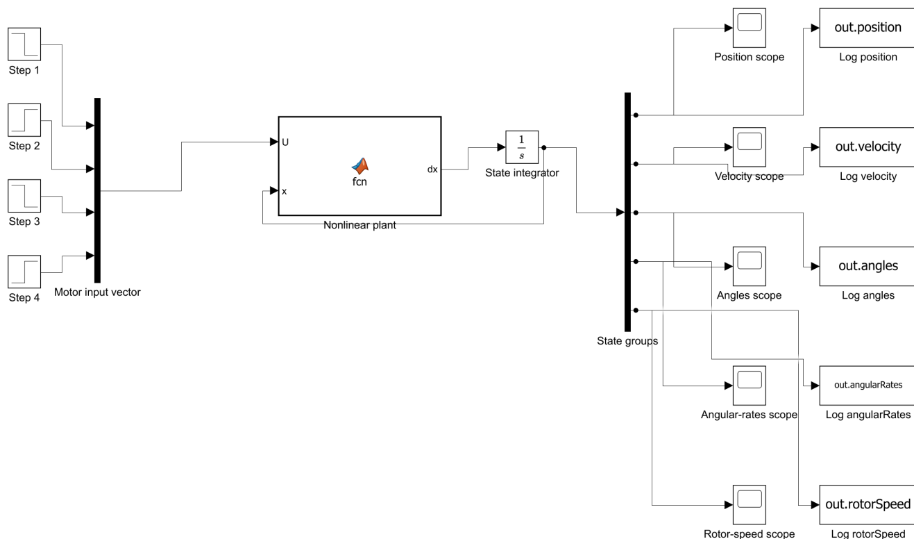
Структура Simulink-моделі
