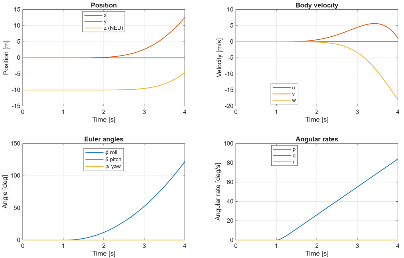
Реакція каналу крену
