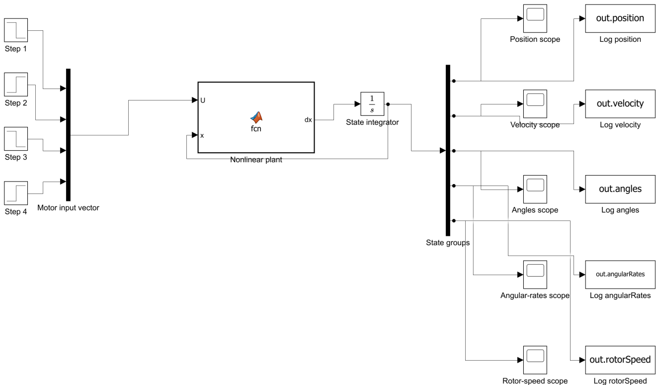
Структура Simulink-моделі
