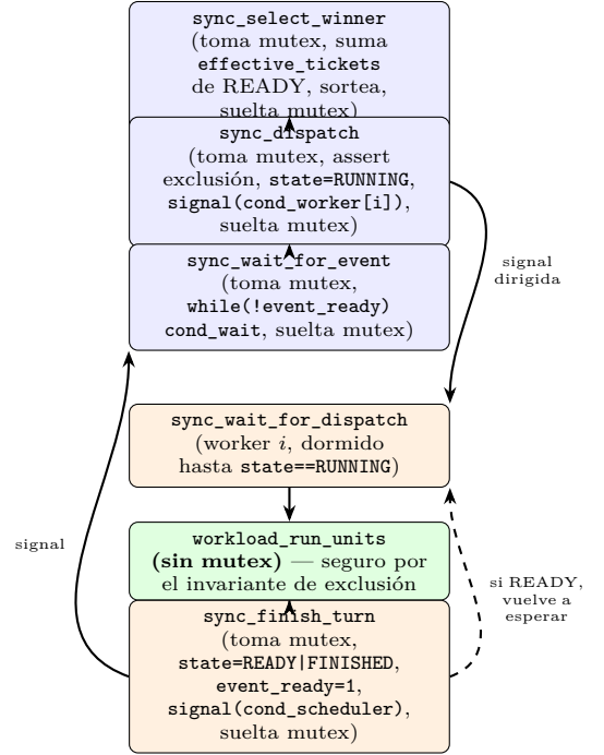
Figura 1: Un ciclo de despacho. Las cajas azules corren en el hilo planificador ( main ); las naranjas y la verde, en el hilo worker de la tarea ganadora. Solo el tramo verde corre sin el mutex tomado.
