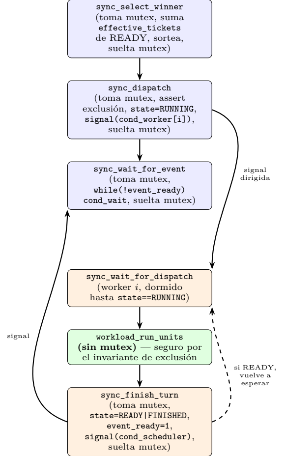
Figura 1: Un ciclo de despacho. Las cajas azules corren en el hilo planificador ( main ); las naranjas y la verde, en el hilo worker de la tarea ganadora. Solo el tramo verde corre sin el mutex tomado.
