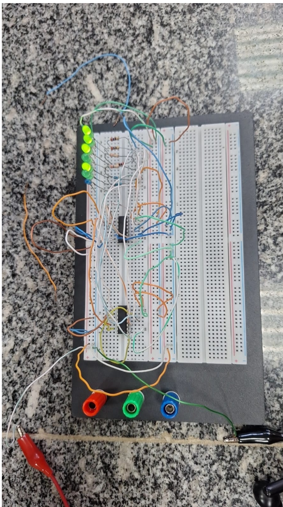
Figure 2: Circuito BCD representação do 23 decimal em binário 0010111
