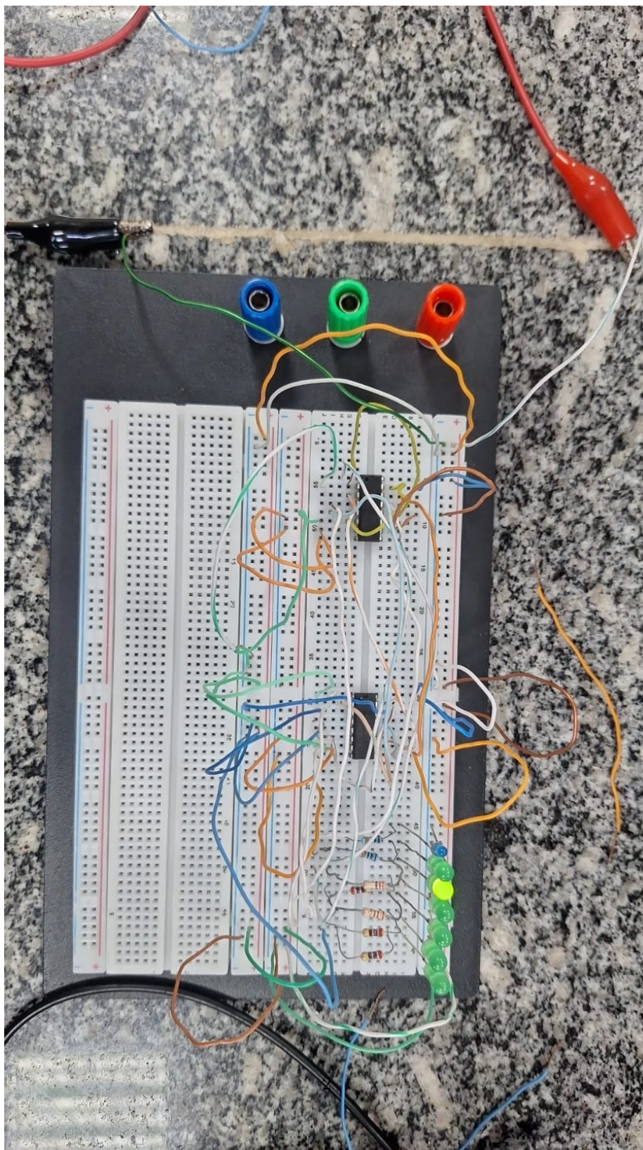
Figure 1: Circuito BCD representação do 16 decimal em binário 0010000
