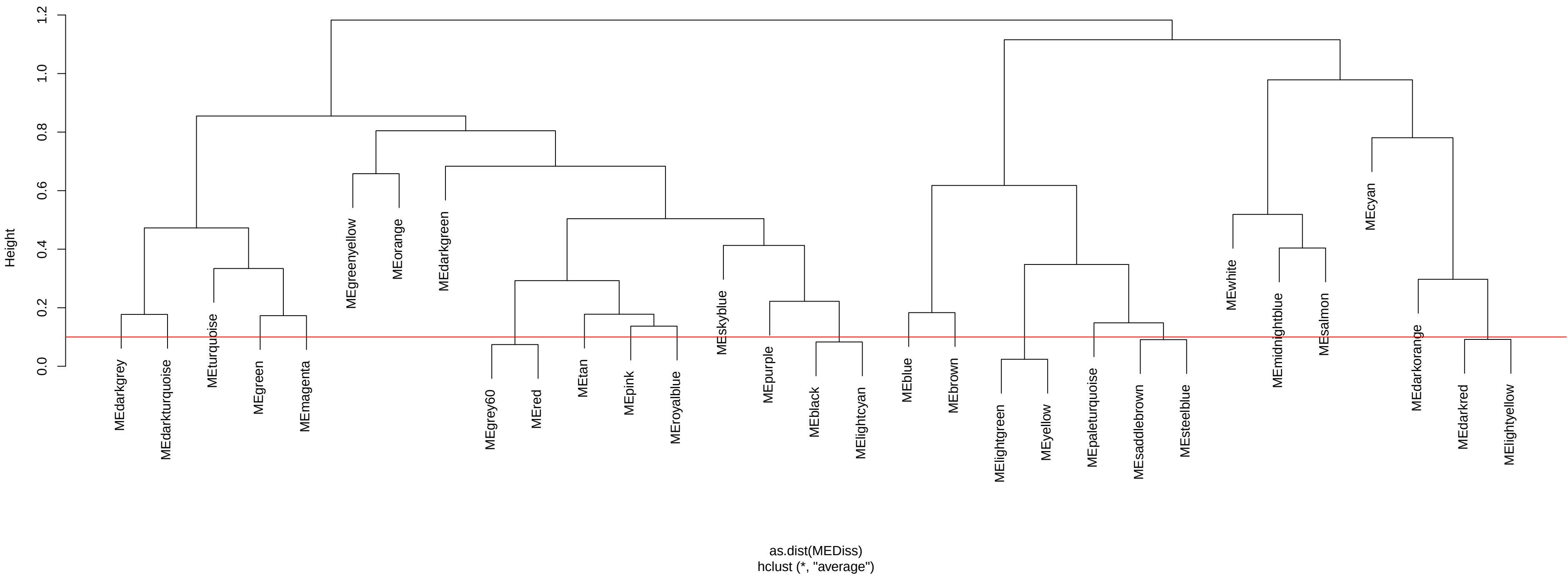
Clustering of Module Eigengenes
