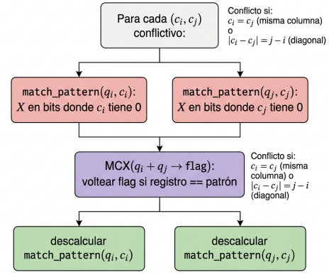
Figura 4. Detección de conflicto (c_i, c_j) con \text{match\_pattern} .
