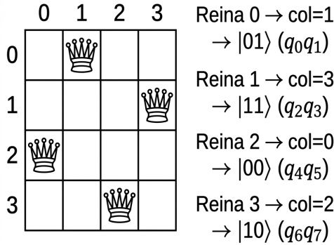
Figura 2. Codificación de [1,3,0,2] para N=4 : 2 qubits por reina.
