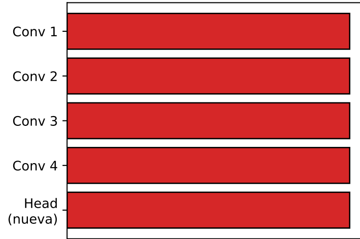
Fine-tuning completo
