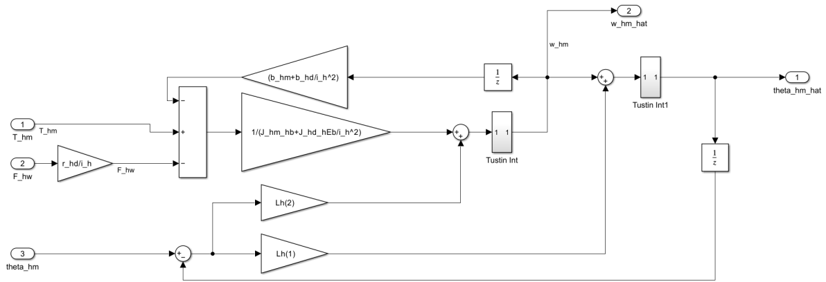
Figura 32: Diagrama de bloques del observador de estados del izaje discretizado (Simulink, T_{s2} = 1 \text{ ms} ).
