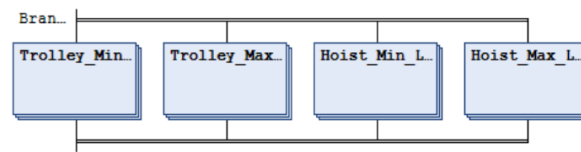
Figura 79: Macropaso Limit_Switch: rama AND con los macropasos Trolley_Min_LS, Trolley_Max_LS, Hoist_Min_LS y Hoist_Max_LS, uno por cada fin de carrera supervisado.
