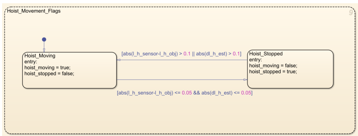
Figura 50: Subestado Hoist_Movement_Flags: detección de izaje detenido.
