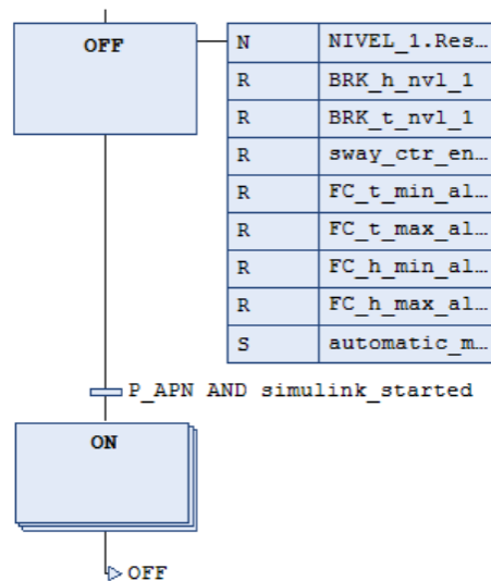
Figura 73: Macropaso Supervisory_Control del programa NIVEL_1. El step OFF inicializa las variables de control y alarma mediante acciones Reset/Set, y permanece activo hasta que se cumple P_APN AND simulink_started . El macropaso ON encapsula la lógica de operación normal y retorna incondicionalmente a OFF al finalizar.
