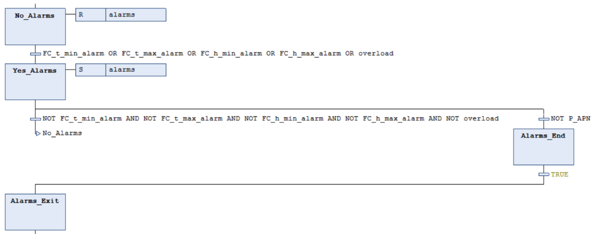
Figura 87: Macropaso Any_Alarms en CODESYS SFC.
