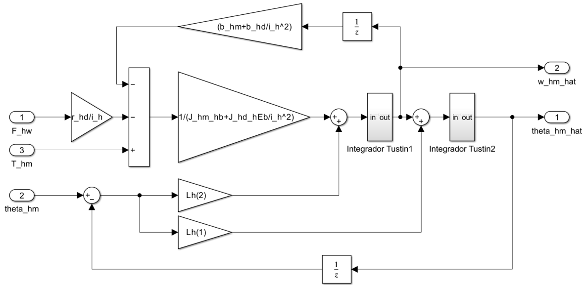
Figura 31: Observador de estados del izaje implementado por bloques en Simulink ( T_{s2} = 1 ms), con las ganancias de retroalimentación L_h .
