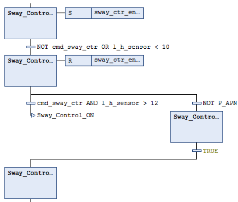
Figura 81: Macropaso Sway_Control1_Mode en CODESYS.
