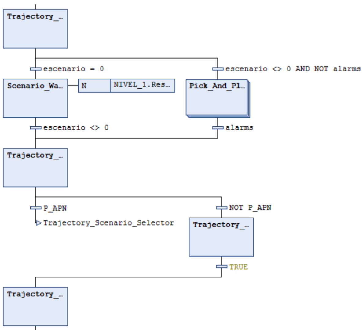
Figura 90: Lógica de selección de escenario y vía de escape del planificador de trayectorias en CODESYS (comportamiento descrito en la sección 3.3.12).
