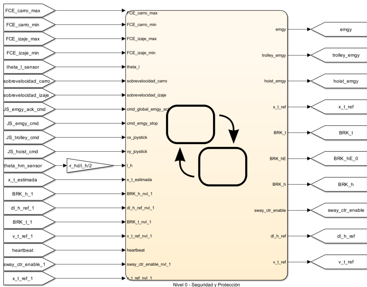
Figura 59: Nivel 0 visto desde el exterior: entradas y salidas del autómata de seguridad y protección (Stateflow).
