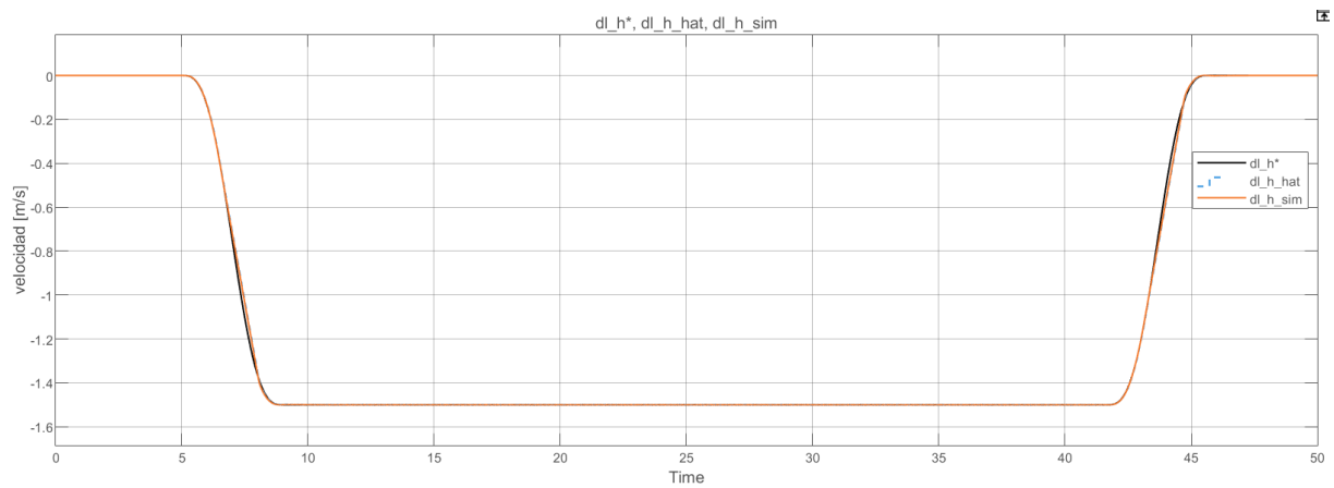
Figura 33: Izaje de carga — velocidad de cable: consigna \dot{l}_h^*(t) , estimada \hat{\dot{l}}_h(t) y simulada \dot{l}_h(t) (carga máxima, perfil trapezoidal).
