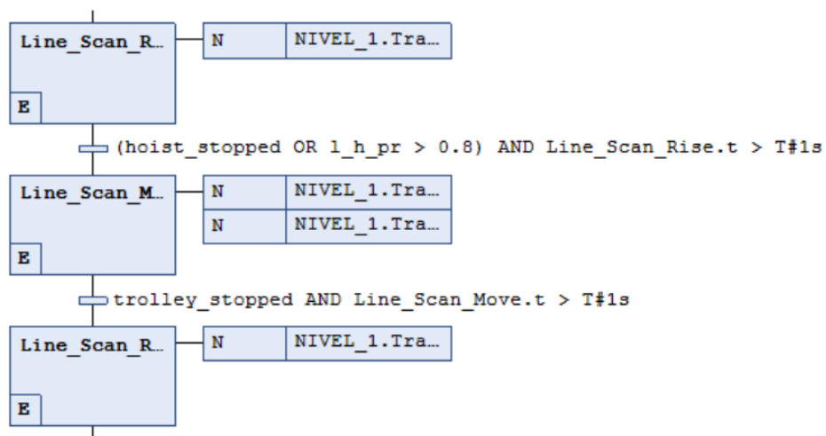
Figura 89: Pasos de inicialización del scan en el planificador de trayectorias de CODESYS: elevación, barrido derecha y barrido izquierda.
