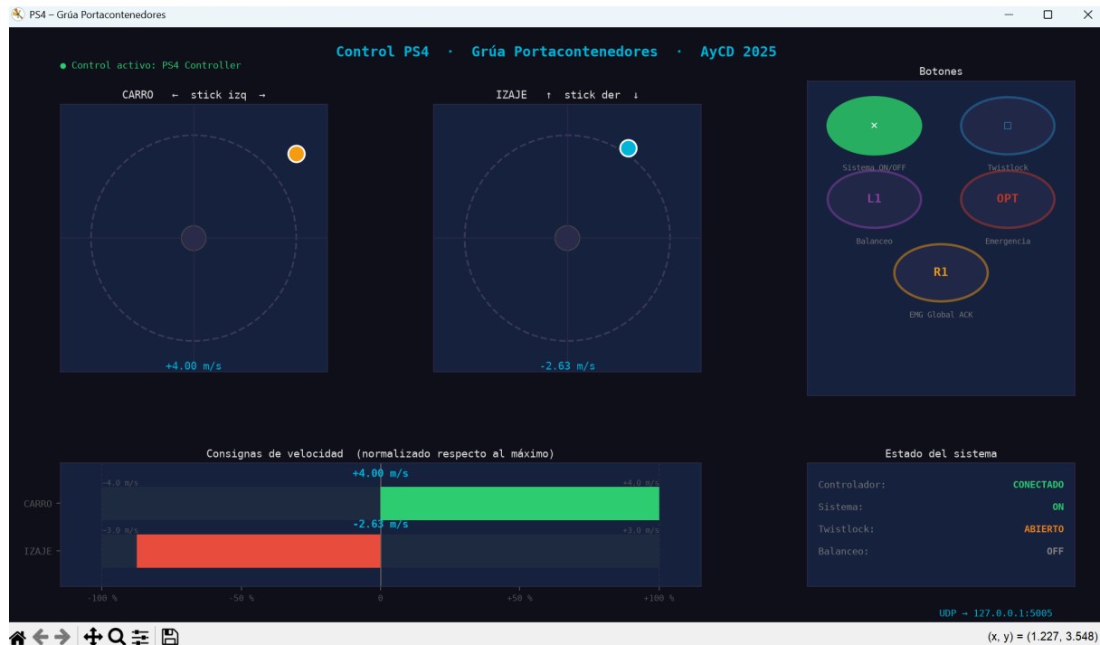
Figura 96: Visualización en tiempo real del script controller_reader.py : sticks analógicos, botones, barras de velocidad y panel de estado del control PS4 durante la operación de la grúa (Python/pygame/matplotlib).
