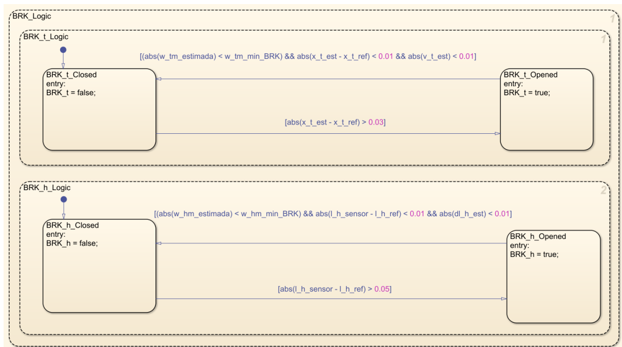
Figura 42: Lógica de frenos en función de la demanda de movimiento: subestados paralelos BRK_t_Logic y BRK_h_Logic.
