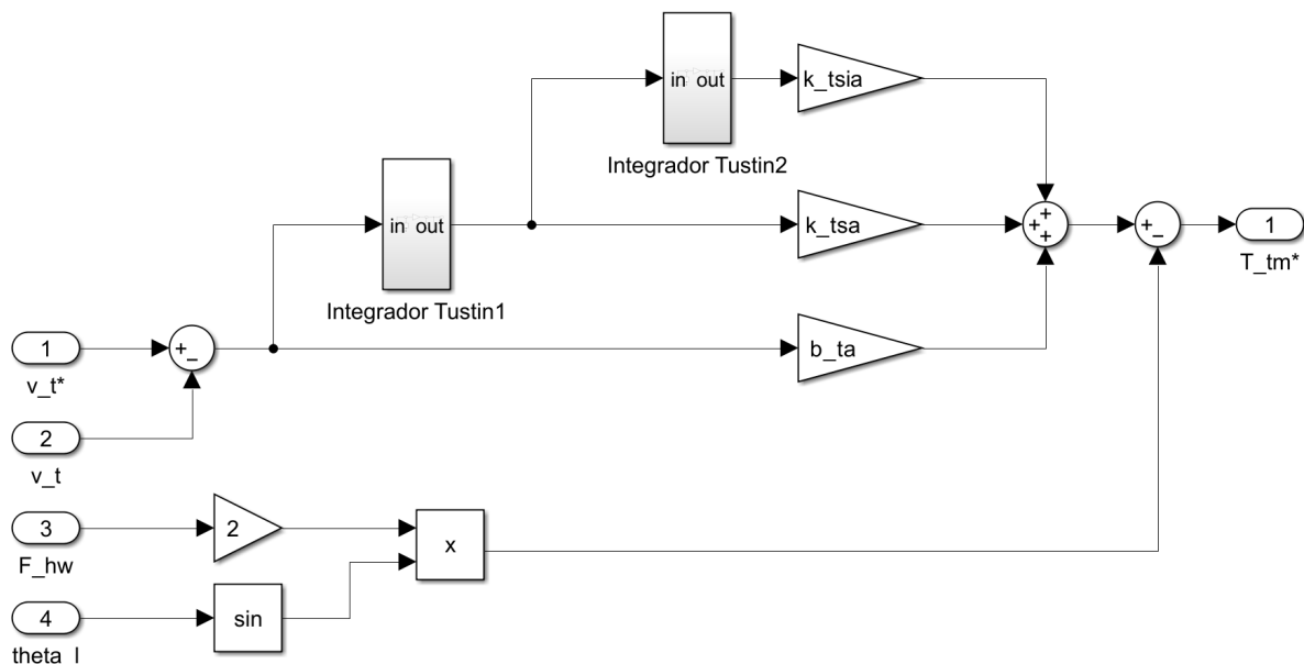
Figura 27: Diagrama de bloques del controlador de traslación del carro discretizado (Simulink, T_{s2} = 1 ms).
