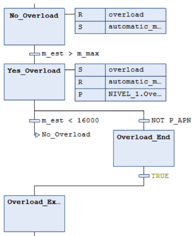
Figura 86: Macropaso Overload_Logic en CODESYS SFC.
