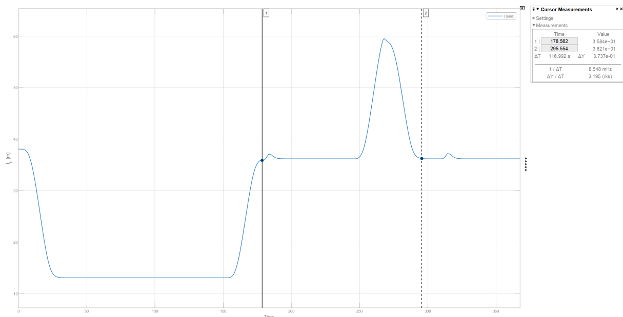
Figura 103: Ciclo simple — evolución de la longitud de cable de izaje l_h(t) .
