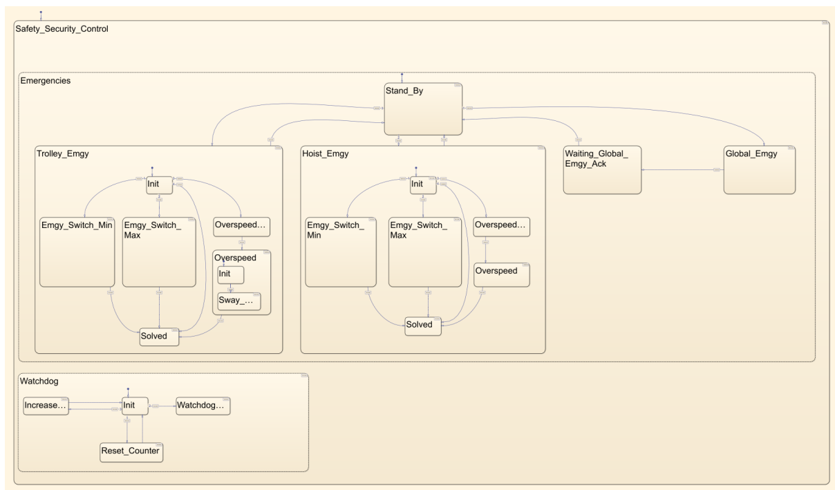
Figura 60: Diagrama de bloques del Nivel 0 completo: estados paralelos Emergencies y Watchdog (Stateflow, T_{s0} = 20 ms).
