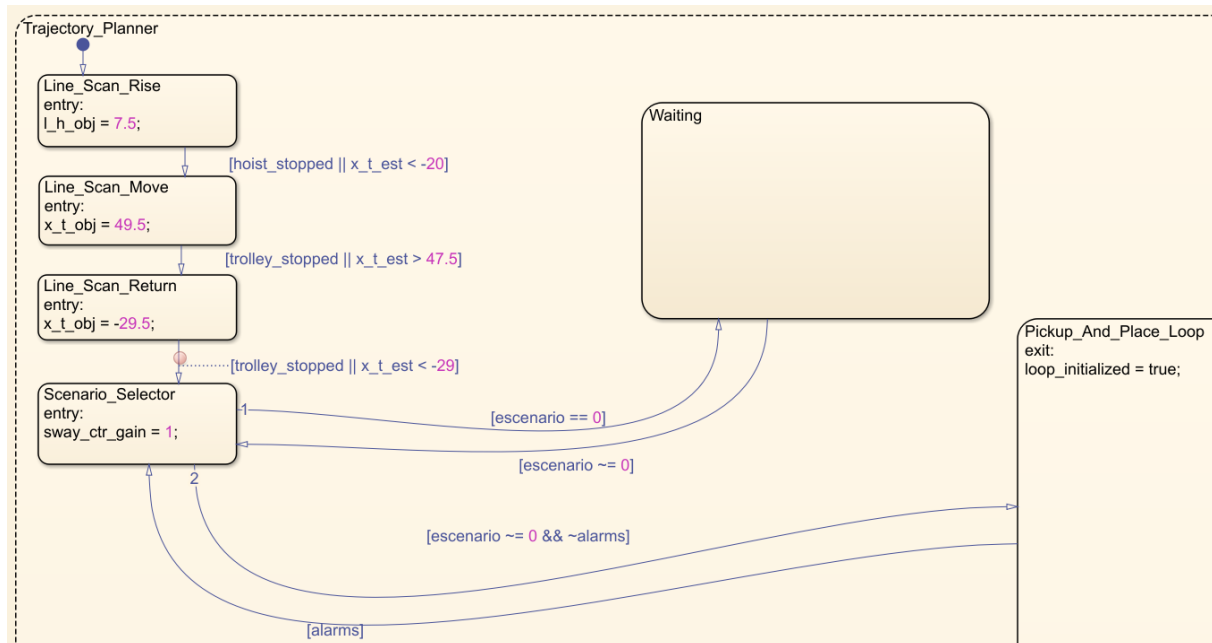
Figura 53: Estructura general del Trajectory_Planner: selección de escenario, escaneo LIDAR y retorno a homing .
