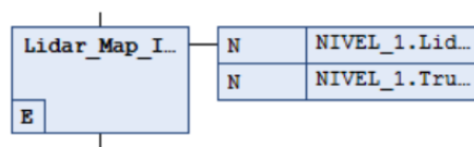
Figura 76: Macropaso Lidar_Map del programa NIVEL_1. Ejecuta las acciones LidarMapEntry (calificador N en el step de entrada E) y LidarMapDuring (calificador N en el step principal), análogas a las acciones entry y during del estado homónimo en Stateflow (sección 3.3.7), ambas implementadas en ST dentro de esta POU.
