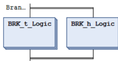
Figura 77: Macropaso BRK_Logic: rama AND que ejecuta en paralelo los macropasos BRK_t_Logic y BRK_h_Logic, uno por cada accionamiento.
