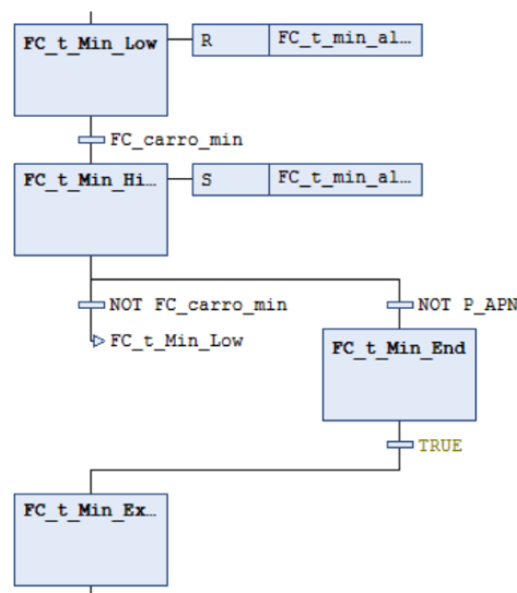
Figura 80: Interior del macropaso Trolley_Min_LS, representativo de los cuatro. Monitorea FC_carro_min para activar o limpiar la alarma FC_t_min_alarm (análogo a la lógica descrita en la sección 2.4). Los demás macropasos (Trolley_Max_LS, Hoist_Min_LS, Hoist_Max_LS) son enteramente análogos sobre sus respectivas señales.
