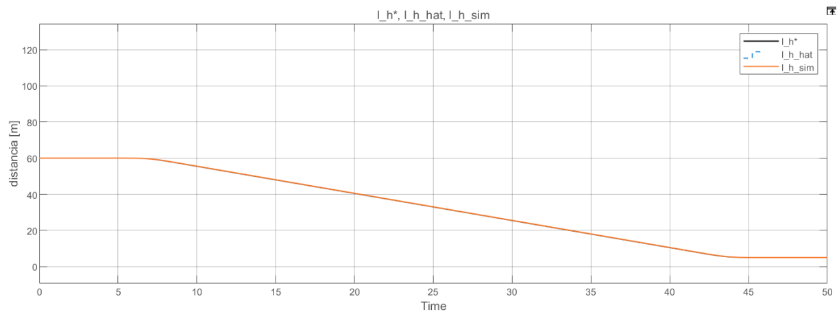
Figura 34: Izaje de carga — posición: consigna l_h^*(t) , estimada \hat{l}_h(t) y simulada l_h(t) (carga máxima, perfil trapezoidal).
