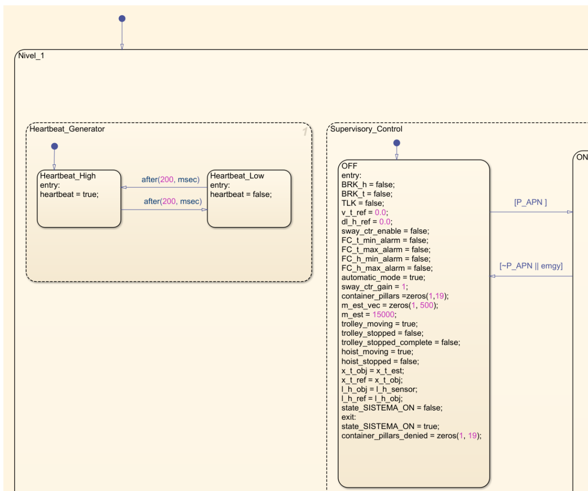
Figura 41: Estructura paralela del Nivel 1: Heartbeat_Generator y estado OFF de Supervisory_Control.
