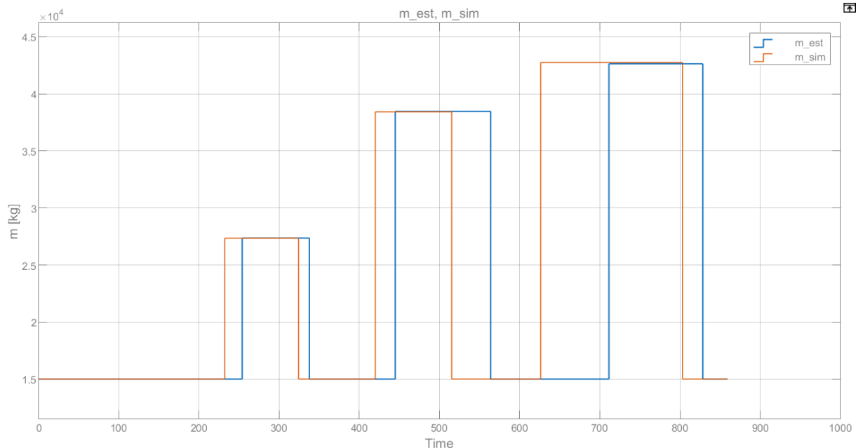
Figura 109: Evolución de la masa estimada \hat{m}(t) a lo largo de múltiples ciclos de carga y descarga para la evaluación del estimador en distintos escenarios de operación.
