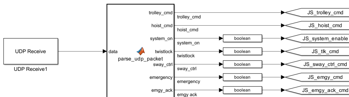
Figura 98: Bloque de lectura UDP completo en Simulink: UDP Receive y MATLAB Function parse_udp_packet con sus siete salidas hacia el sistema de control.
