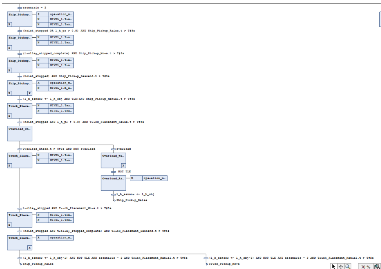
Figura 92: Recorrido de pasos para la operación de descarga (barco → camión) dentro del macropaso Pick_And_Place_Loop.
