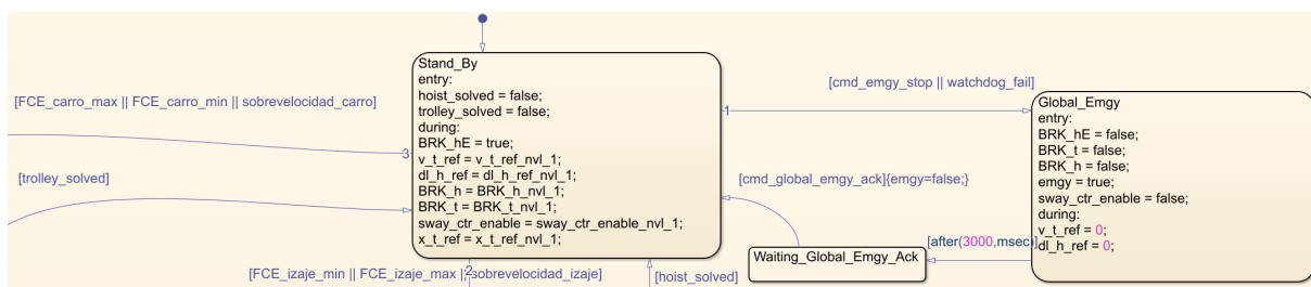
Figura 61: Estado Emergencies: estado de entrada Stand_By (Stateflow).
