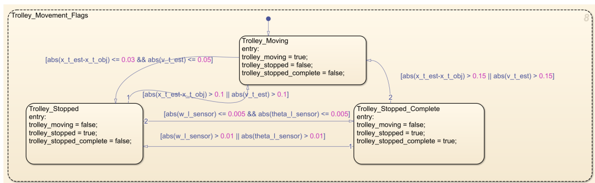
Figura 49: Subestado Trolley_Movement_Flags: detección de carro detenido con condición de balanceo amortiguado.
