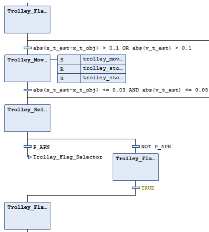
Figura 82: Macropaso Trolley_Movement_Flags en CODESYS: primer elemento de la rama OR (comportamiento descrito en la sección 3.3.9).
