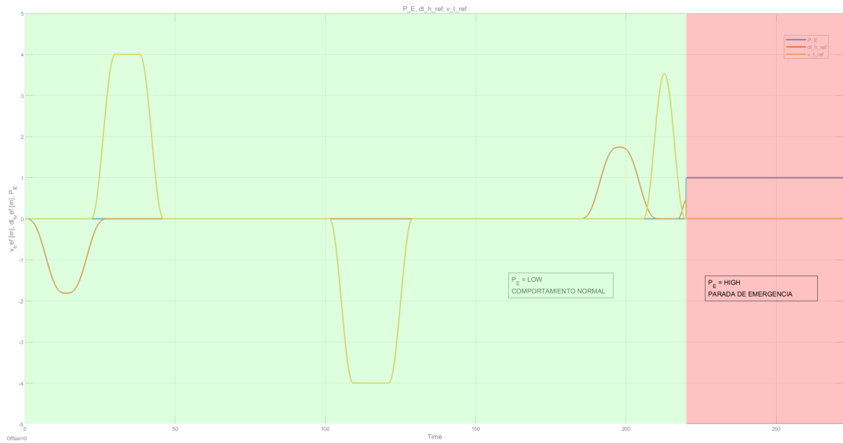
Figura 107: Referencias de velocidad del carro ( v_{t,ref} ) y del izaje ( h_{t,ref} ) ante una parada de emergencia: caída inmediata a cero al activarse P_E .
