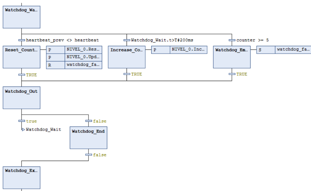
Figura 69: Macropaso Watchdog del programa NIVEL_0. Su funcionamiento es análogo al descrito para el estado homónimo en el Statechart de Stateflow (sección 3.4.1). Las acciones ResetCounter, UpdateHeartbeat e IncreaseCounter están implementadas en ST como acciones asociadas a los pasos de esta POU. Al final del macropaso se incorpora una rama OR con transición false hacia el step Watchdog_Exit, recurso requerido por IEC 61131-3 para que el compilador acepte el diagrama SFC como conforme a la norma.
