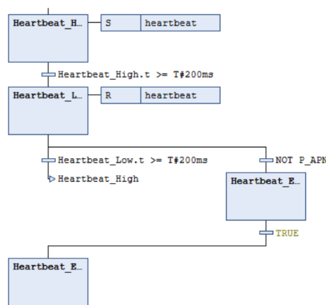
Figura 72: Macropasado Heartbeat_Generator del programa NIVEL_1, análogo al diseño de Stateflow de la sección 3.3.1. Al final se provee el camino de escape mencionado anteriormente, requerido por IEC 61131-3 para conformidad del compilador.
