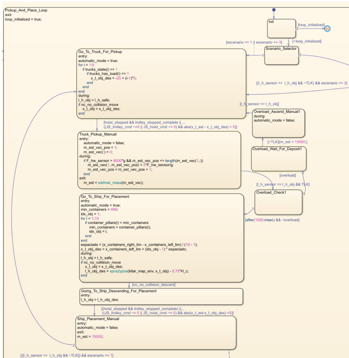
Figura 55: Secuencia de estados del Escenario 1 (descarga tierra → barco) dentro de Pickup_And_Place_Loop.
