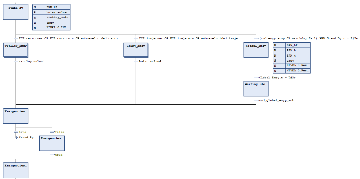
Figura 70: Macropaso Emergencias del programa NIVEL_0, análogo al diseño de Stateflow de la sección 3.4.1. La acción LVL1PASS, con calificador N en el step Stand_By, permite el paso de las consignas provenientes del Nivel 1 (BRK_t, BRK_h, v_t_ref, x_t_ref, dl_h_ref, l_h_ref, sway_ctr_enable) mientras no haya falla activa. Las acciones ResetTrolleyRef y ResetHoistRef, activadas ante emergencia, sustituyen dichas consignas por velocidades nulas y referencias de posición iguales al valor actual del sensor o estimación, de modo que no induzcan movimiento sobre el eje afectado. Las tres acciones están implementadas en ST dentro de esta POU.
