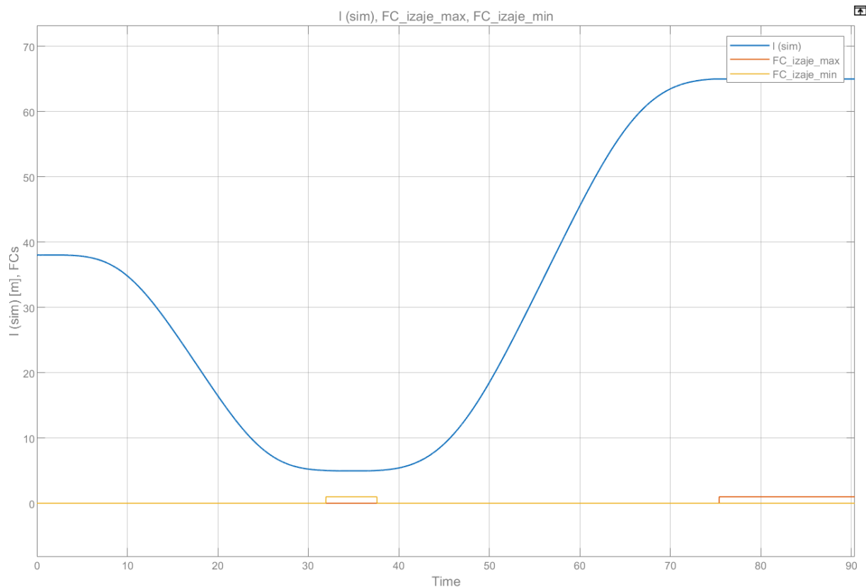
Figura 106: Activación de fines de carrera de operación del izaje: trayectoria desde 5 hasta 65 m de longitud de cable.
