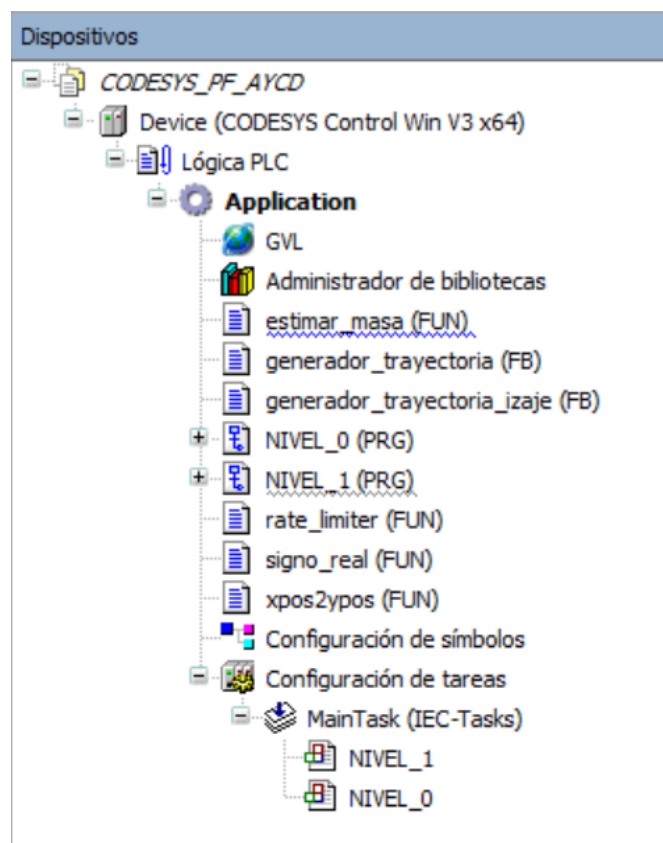
Figura 67: Árbol de proyecto CODESYS_PF_AYCD. Bajo Application se agrupan las variables globales (GVL), las funciones auxiliares ( estimar_masa , rate_limiter , signo_real , xpos2ypos ), los bloques de función de generación de trayectorias ( generador_trayectoria , generador_trayectoria_izaje ), y las POU tipo Programa NIVEL_0 y NIVEL_1 (cada una con acciones internas). La Configuración de símbolos habilita la interfaz OPC UA. En Configuración de tareas , MainTask ejecuta cíclicamente ambos programas.
