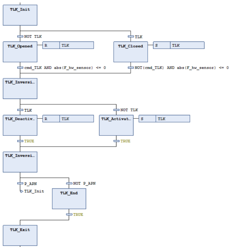
Figura 88: Macropaso TLK_Logic en CODESYS.
