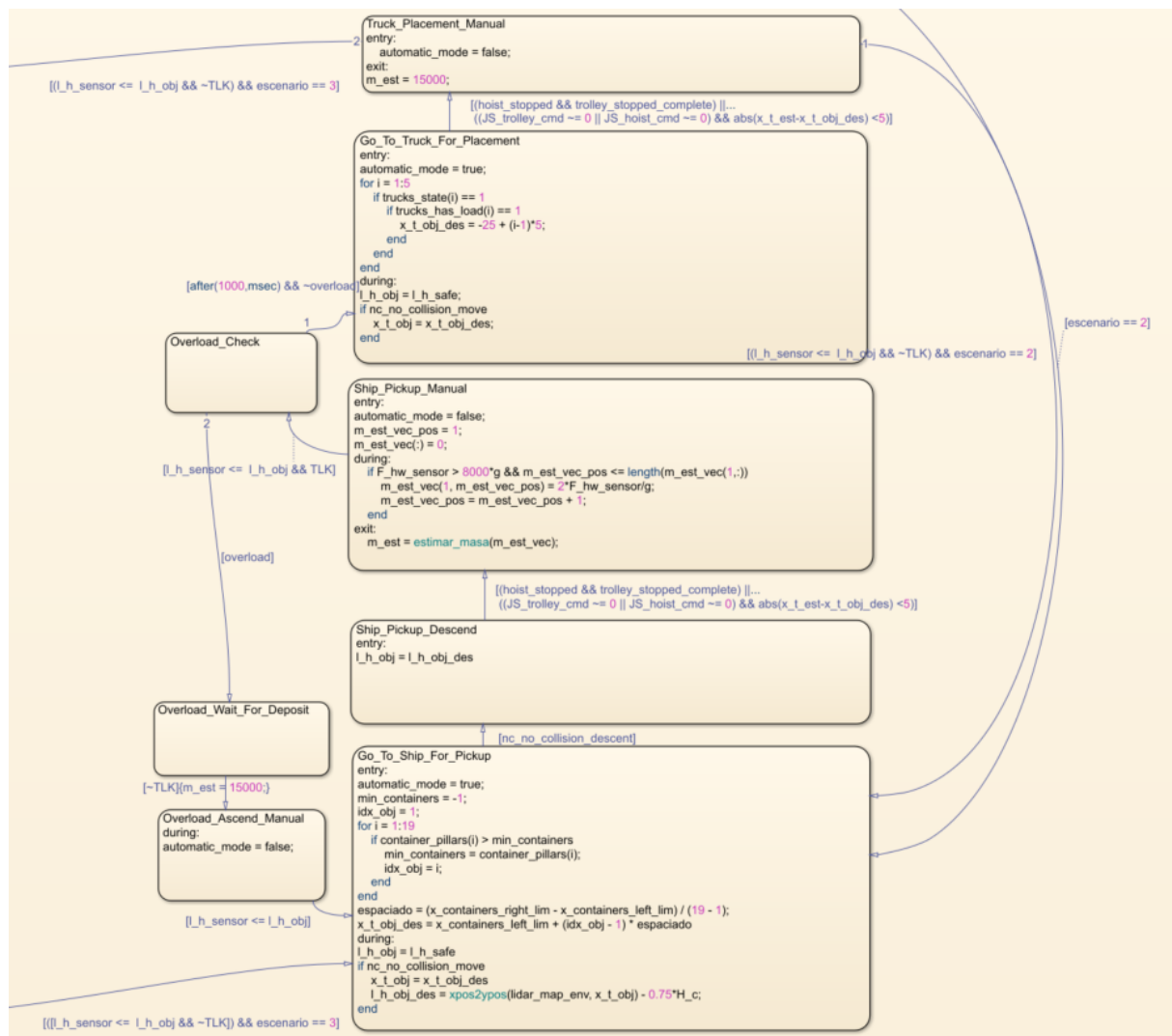
Figura 57: Secuencia de estados del Escenario 2 (carga barco → tierra) dentro de Pickup_And_Place_Loop.
