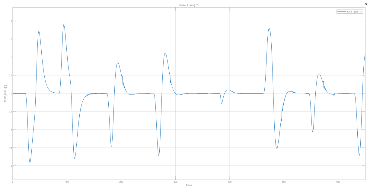
Figura 104: Evolución del ángulo de balanceo \theta_l(t) a lo largo de múltiples ciclos doubles (carga + descarga) con el controlador de oscilación activo.
