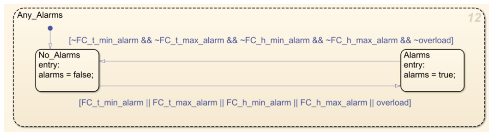
Figura 51: Subestado Any_Alarms : agrupación de alarmas de fines de carrera y sobrecarga en una señal booleana unificada.
