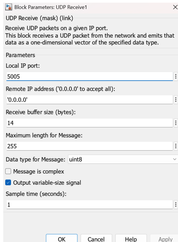
Figura 97: Configuración del bloque UDP Receive en Simulink: puerto 5005, buffer de 14 bytes, salida uint8 (Instrument Control Toolbox).
