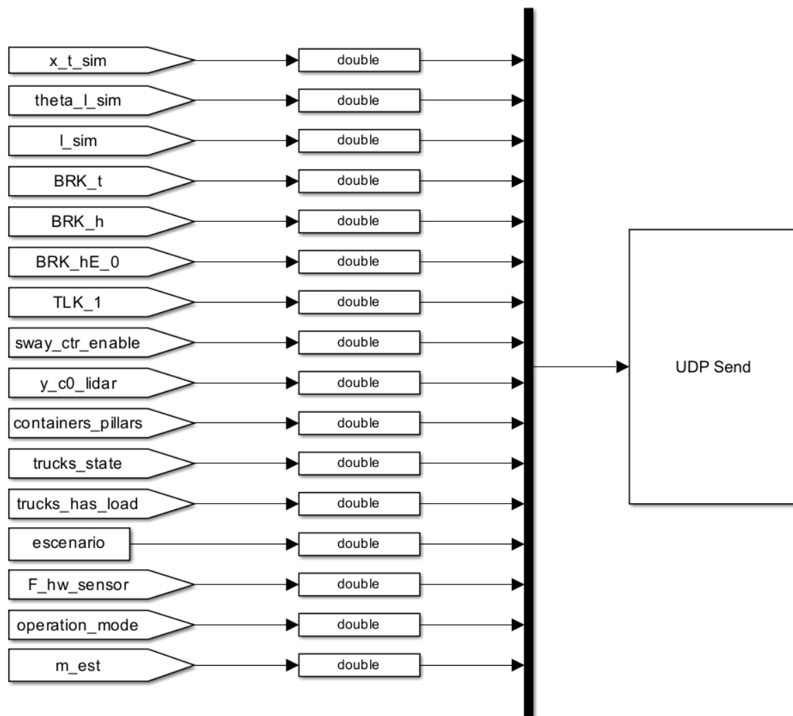
Figura 100: Subsistema transmisor completo en Simulink: multiplexado de señales y bloque UDP Send hacia RT_VIEW.
