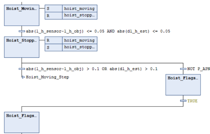
Figura 84: Macropaso Hoist_Movement_Flags en CODESYS (comportamiento descrito en la sección 3.3.9).
