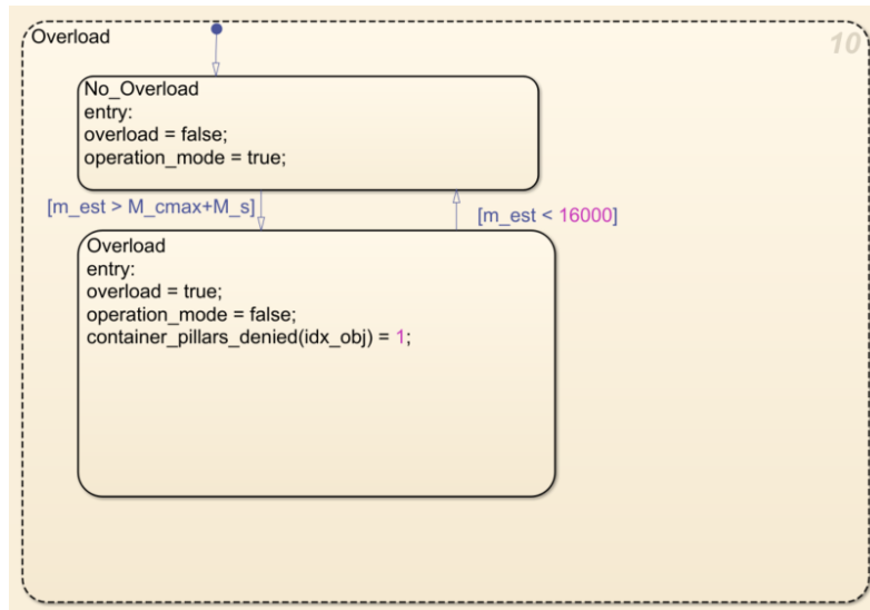
Figura 48: Subestado Overload: detección de sobrecarga con activación de alarma y forzado a modo manual.
