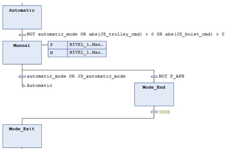
Figura 85: Macropaso Mode en CODESYS.
