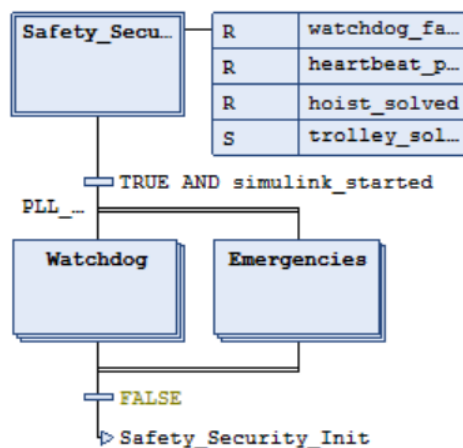
Figura 68: SFC del programa NIVEL_0 en CODESYS. El step inicial Safety_Security inicializa mediante acciones Reset/Set las variables de diagnóstico (watchdog_failed, heartbeat_present, hoist_solved, trolley_solved). La transición TRUE AND simulink_started habilita una rama AND que lanza en paralelo los pasos Watchdog y Emergencies, manteniendo ambas lógicas activas de forma concurrente durante toda la operación. Ante una condición FALSE, se ejecuta la acción Safety_Security_Init que reinicializa el nivel.
