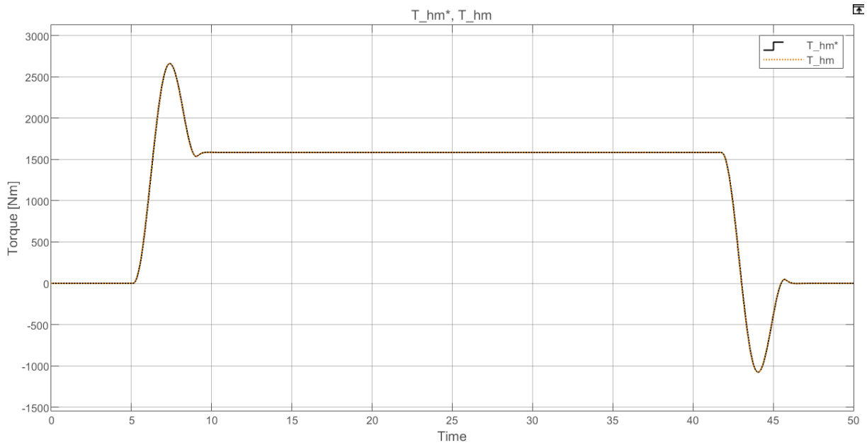
Figura 35: Izaje de carga — comparativa de torque: consigna T_{hm}^*(t) y torque a la salida del modulador T_{hm}(t) (carga máxima, perfil trapezoidal).
