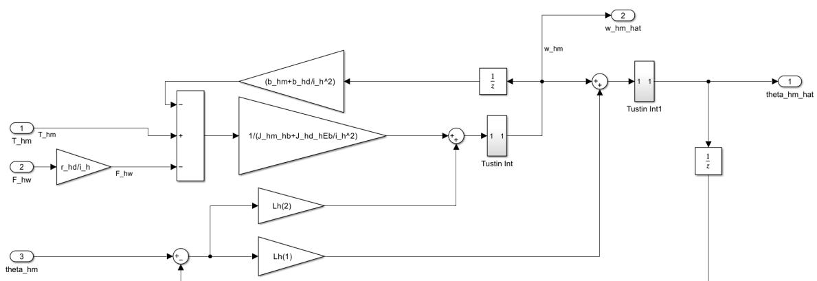
Figura 34: Diagrama de bloques del observador de estados del izaje discretizado (Simulink, T_{s2} = 1 ms).
