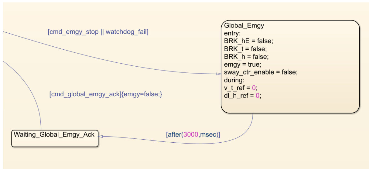
Figura 64: Subestado Global_Emgy completo: acciones de entrada, espera de 3 s y reconocimiento del operador en Waiting_Global_Emgy_Ack (Stateflow).
