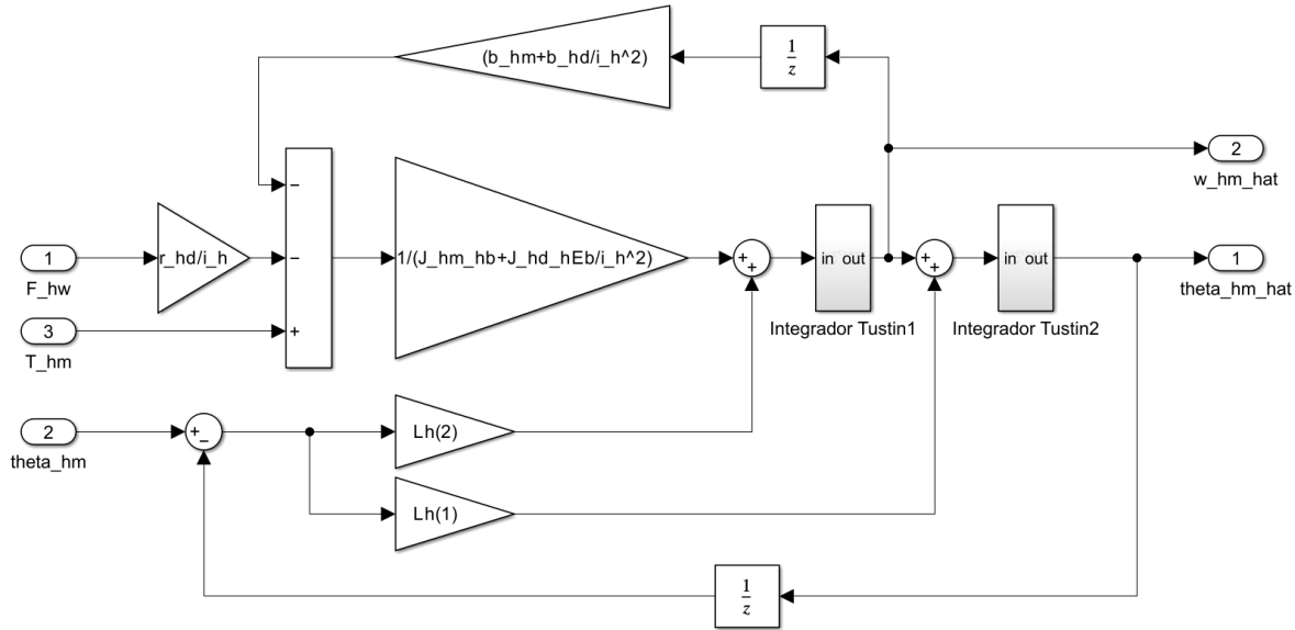
Figura 32: Observador de estados del izaje implementado por bloques en Simulink ( T_{s2} = 1 \text{ ms} ), con las ganancias de retroalimentación \mathbf{L}_h .
