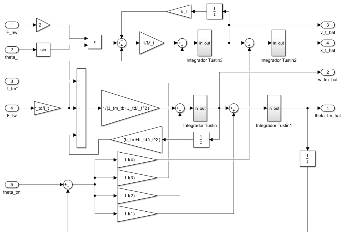
Figura 25: Observador de estados del carro implementado por bloques en Simulink ( T_{s2} = 1 ms), con las ganancias de retroalimentación L_t .
