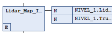
Figura 75: Macropaso Lidar_Map del programa NIVEL_1. Ejecuta las acciones LidarMapEntry (calificador N en el step de entrada E) y LidarMapDuring (calificador N en el step principal), análogas a las acciones entry y during del estado homónimo en Stateflow (sección 3.3.8), ambas implementadas en ST dentro de esta POU.
