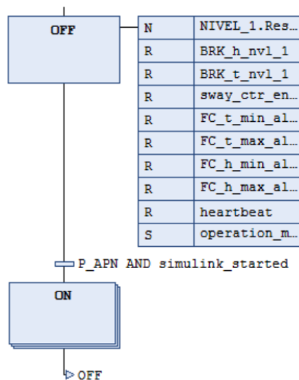
Figura 72: Macropaso Supervisory_Control del programa NIVEL_1. El step OFF inicializa las variables de control y alarma mediante acciones Reset/Set, y permanece activo hasta que se cumple P_APN AND simulink_started. El macropaso ON encapsula la lógica de operación normal y retorna incondicionalmente a OFF al finalizar.
