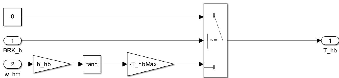
Figura 9: Diagrama de bloques del modelo del freno de operación del izaje (Simulink).
