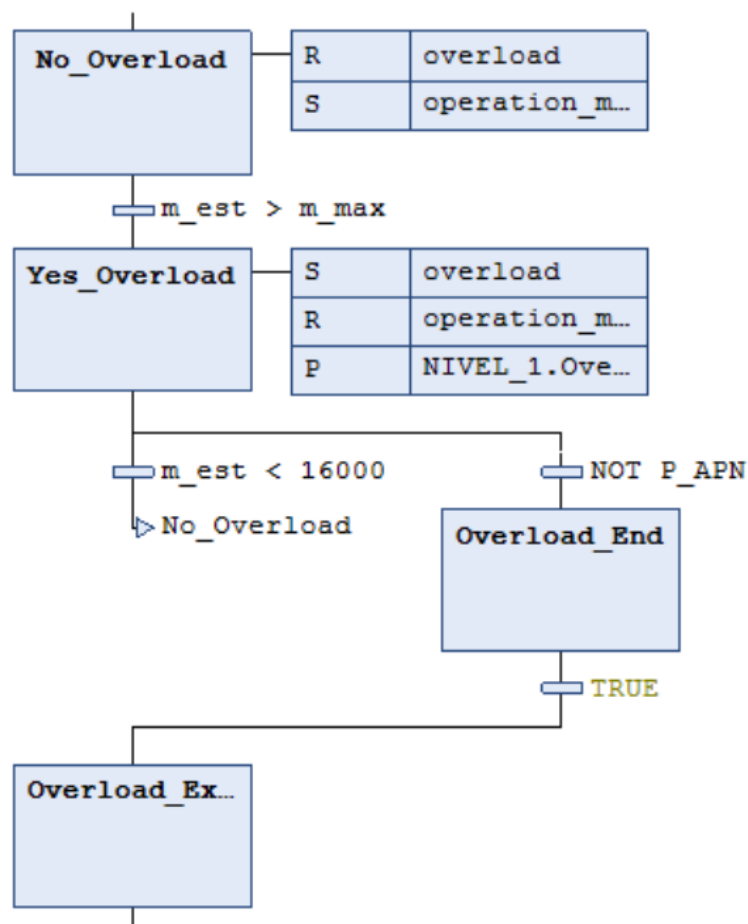
Figura 87: Macropaso Overload_Logic en CODESYS SFC.
