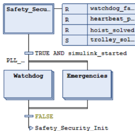
Figura 67: SFC del programa NIVEL_0 en CODESYS. El step inicial Safety_Security inicializa mediante acciones Reset/Set las variables de diagnóstico (watchdog_failed, heartbeat_present, hoist_solved, trolley_solved). La transición TRUE AND simulink_started habilita una rama AND que lanza en paralelo los pasos Watchdog y Emergencies, manteniendo ambas lógicas activas de forma concurrente durante toda la operación. Ante una condición FALSE, se ejecuta la acción Safety_Security_Init que reinicializa el nivel.
