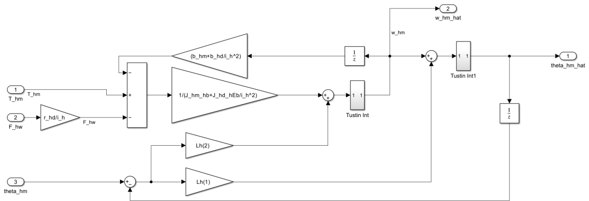
Figura 32: Diagrama de bloques del observador de estados del izaje discretizado (Simulink, T_{s2} = 1 ms).
