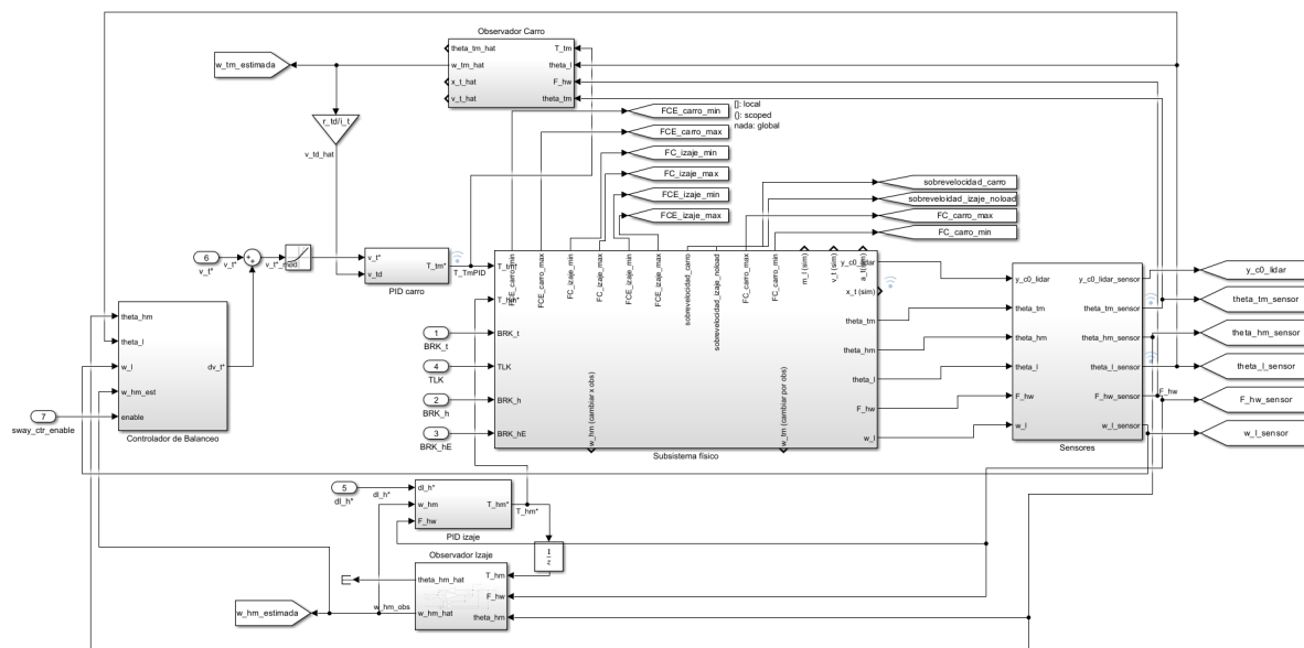
Figura 39: Diagrama de bloques del Nivel 2 completo: controladores de traslación, izaje y oscilación integrados en Simulink ( T_{s2} = 1 ms). Para mejorar la visibilidad del diagrama se han omitido las entradas a los generadores de trayectorias y otras consignas externas provenientes del Nivel 1.
