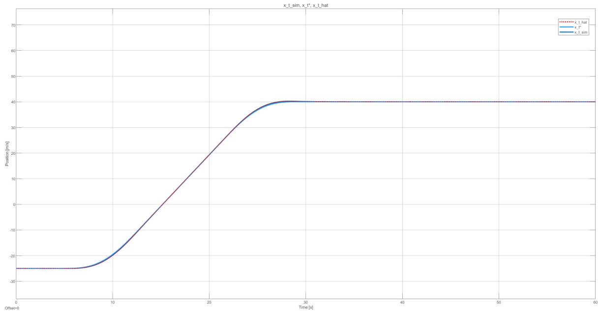
Figura 29: Traslación del carro — posición: consigna x_t^*(t) , estimada \hat{x}_t(t) y simulada x_t(t) (carga máxima, perfil trapezoidal).
