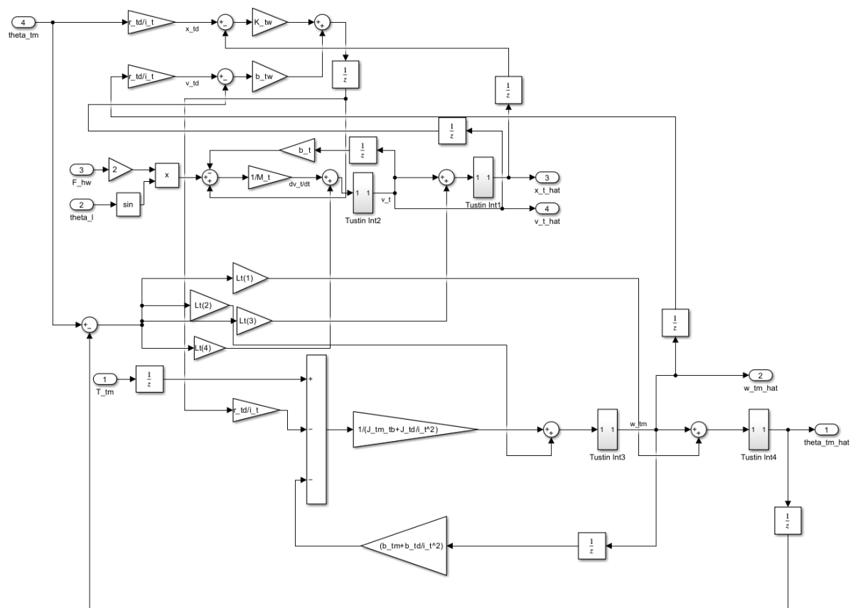
Figura 27: Diagrama de bloques del observador de estados del carro discretizado (Simulink, T_{s2} = 1 \text{ ms} ).
