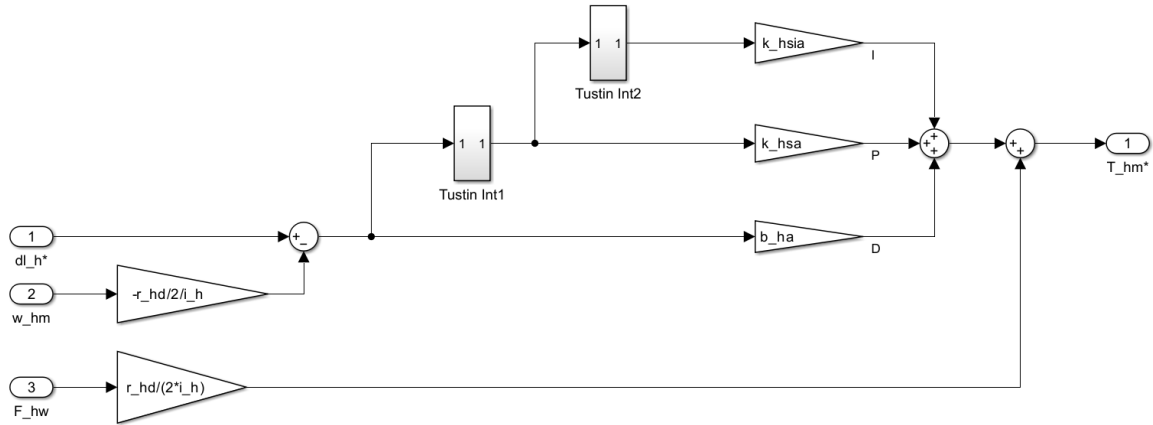
Figura 31: Diagrama de bloques del controlador de izaje de carga discretizado (Simulink, T_{s2} = 1 ms).
