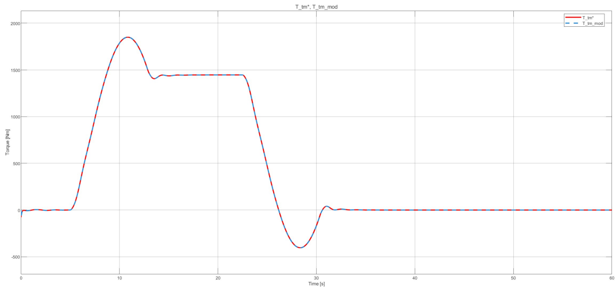
Figura 30: Traslación del carro — comparativa de torque: consigna T_{tm}^*(t) y salida del modulador T_{tm}(t) (spreader vacío, perfil trapezoidal).
