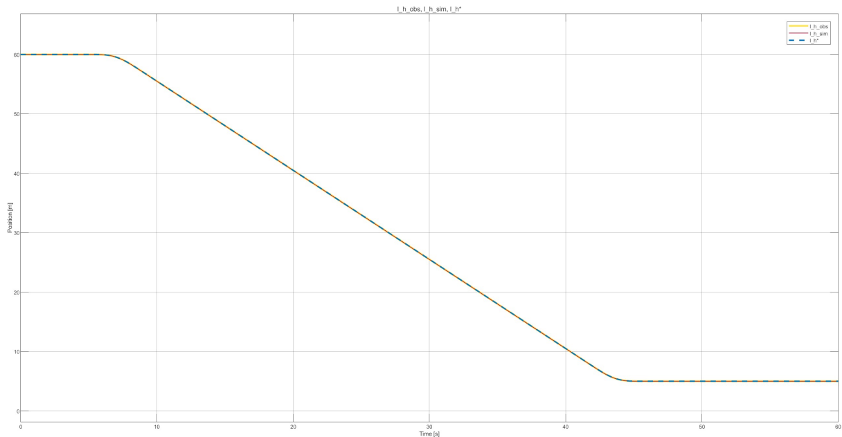
Figura 34: Izaje de carga — posición: consigna l_h^*(t) , estimada \hat{l}_h(t) y simulada l_h(t) (carga máxima, perfil trapezoidal).
