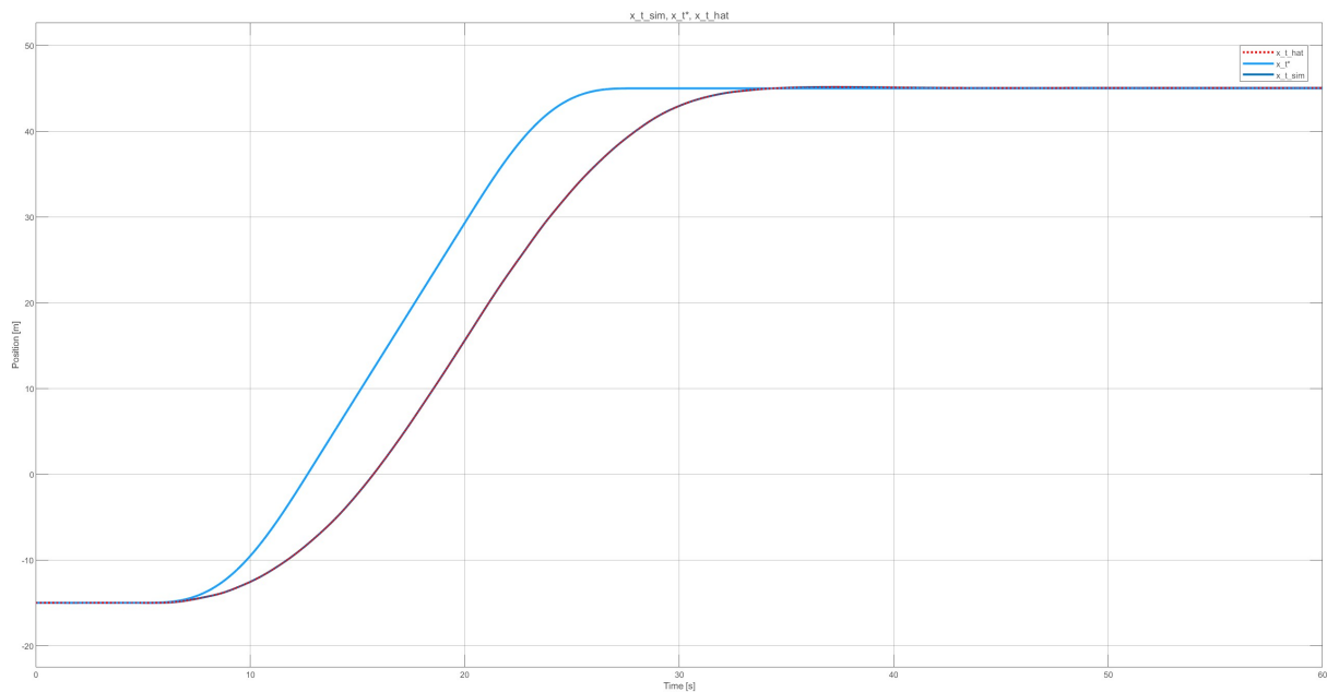
Figura 37: Controlador de balanceo — posición: consigna original x_t^*(t) , simulada x_t(t) y estimada \hat{x}_t(t) .
