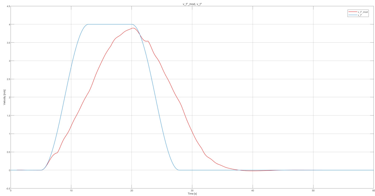
Figura 36: Controlador de balanceo — velocidad: consigna original v_t^*(t) y consigna modificada por el controlador de balanceo v_{t,mod}^*(t) .
