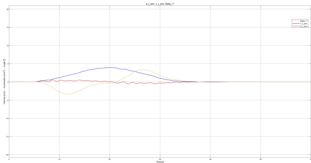
Figura 38: Controlador de balanceo — evolución conjunta de \theta_l(t) , v_t(t) y a_t(t) para analizar el comportamiento del ángulo de balanceo en cada región de aceleración y velocidad del carro.
