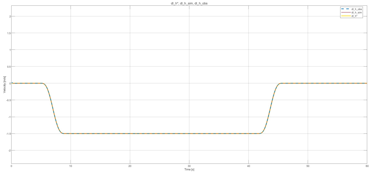
Figura 33: Izaje de carga — velocidad de cable: consigna \dot{l}_h^*(t) , estimada \hat{\dot{l}}_h(t) y simulada \dot{l}_h(t) (carga máxima, perfil trapezoidal).
