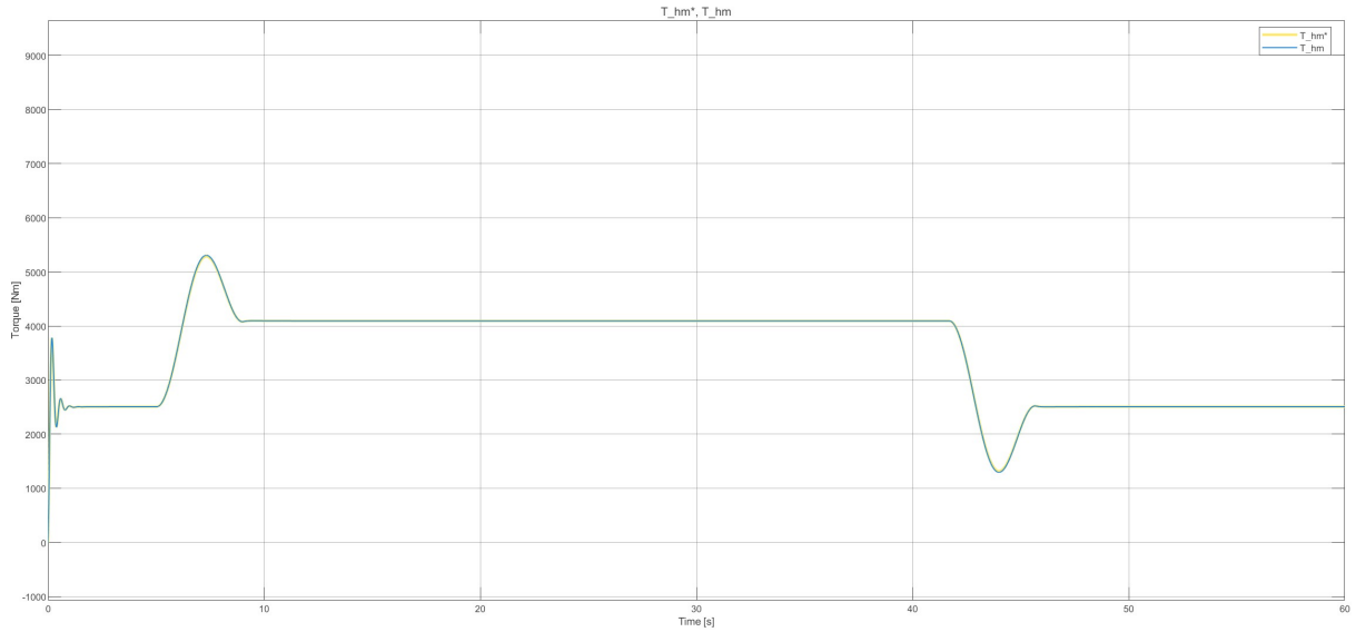
Figura 35: Izaje de carga — comparativa de torque: consigna T_{hm}^*(t) y torque a la salida del modulador T_{hm}(t) (carga máxima, perfil trapezoidal).
