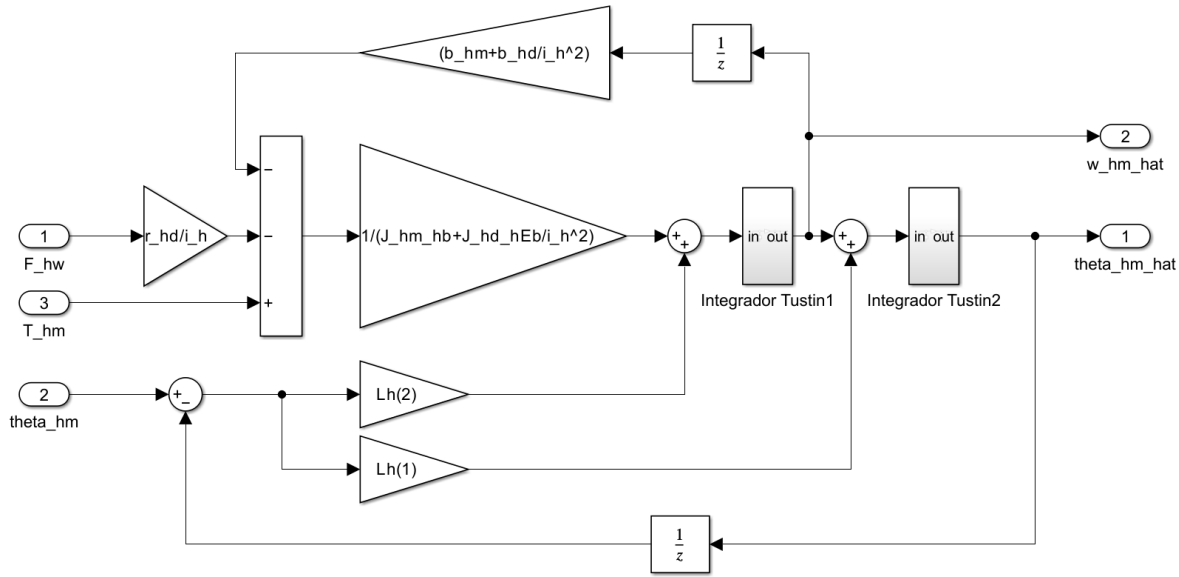
Figura 40: Observador de estados del izaje implementado por bloques en Simulink ( T_{s2} = 1 \text{ ms} ), con las ganancias de retroalimentación \mathbf{L}_h .
