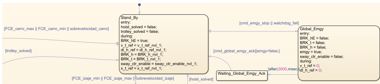
Figura 57: Estado Emergencies: estado de entrada Stand_By (Stateflow).
