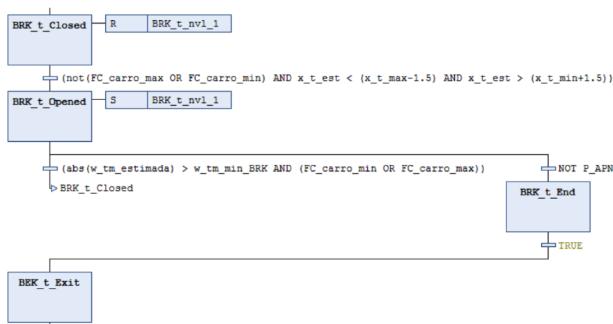
Figura 73: Interior del macropaso BRK_t_Logic. El step BRK_t_Closed mantiene el freno aplicado (R BRK_t_nv1_1) hasta que la posición estimada del carro se encuentra dentro de la zona segura y no hay fin de carrera activo, condición bajo la cual se habilita la apertura (BRK_t_Opened, S BRK_t_nv1_1). El freno se vuelve a aplicar si la velocidad supera el umbral w_{tm\_min\_BRK} con un fin de carrera activo, retornando a BRK_t_Closed. La rama OR con NOT P_APN provee el camino de salida del macropaso. El caso del izaje (BRK_h_Logic) es enteramente análogo.
