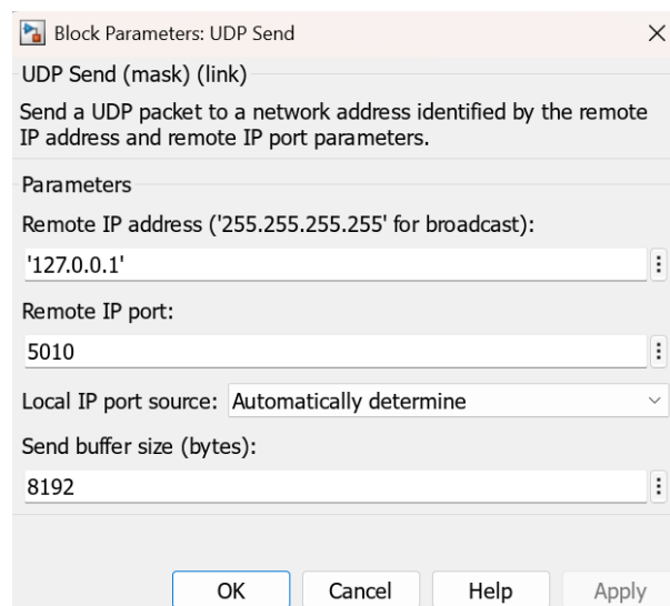
Figura 92: Configuración del bloque UDP Send en Simulink para el canal de datos de RT_VIEW (puerto 5010, loopback).
