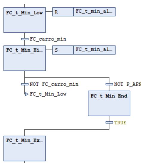
Figura 75: Interior del macropaso Trolley_Min_LS, representativo de los cuatro. Monitorea FC_carro_min para activar o limpiar la alarma FC_t_min_alarm (análogo a la lógica descrita en la sección 2.4). Los demás macropasos (Trolley_Max_LS, Hoist_Min_LS, Hoist_Max_LS) son enteramente análogos sobre sus respectivas señales.
