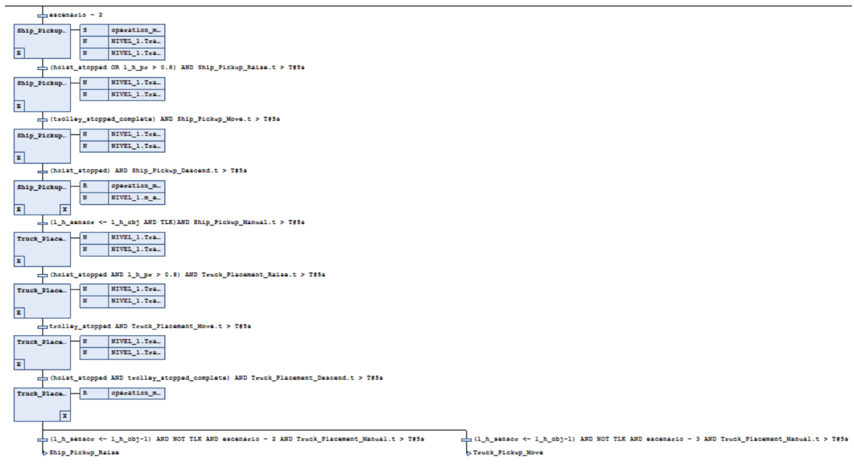
Figura 85: Recorrido de pasos para la operación de descarga (barco → camión) dentro del macropaso Pick_And_Place_Loop.
