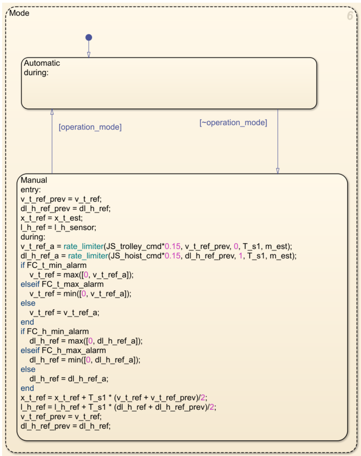
Figura 46: Subestado Mode: lógica de conmutación entre operación manual y automática.
