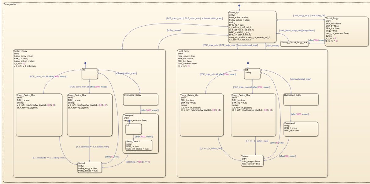
Figura 58: Estado Emergencias completo: Stand_By y transiciones hacia Trolley_Emg, Hoist_Emg y Global_Emg (Stateflow).
