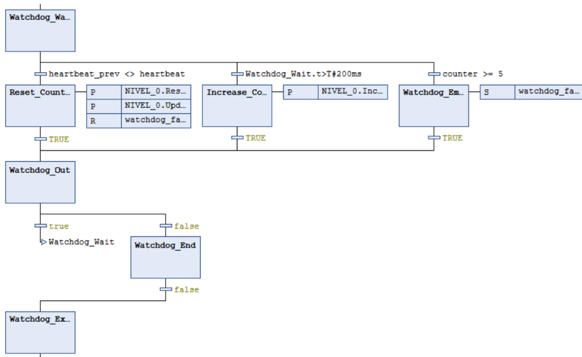
Figura 65: Macropaso Watchdog del programa NIVEL_0. Su funcionamiento es análogo al descrito para el estado homónimo en el Statechart de Stateflow (sección 3.4.1). Las acciones ResetCounter, UpdateHeartbeat e IncreaseCounter están implementadas en ST como acciones asociadas a los pasos de esta POU. Al final del macropaso se incorpora una rama OR con transición false hacia el step Watchdog_Exit, recurso requerido por IEC 61131-3 para que el compilador acepte el diagrama SFC como conforme a la norma.
