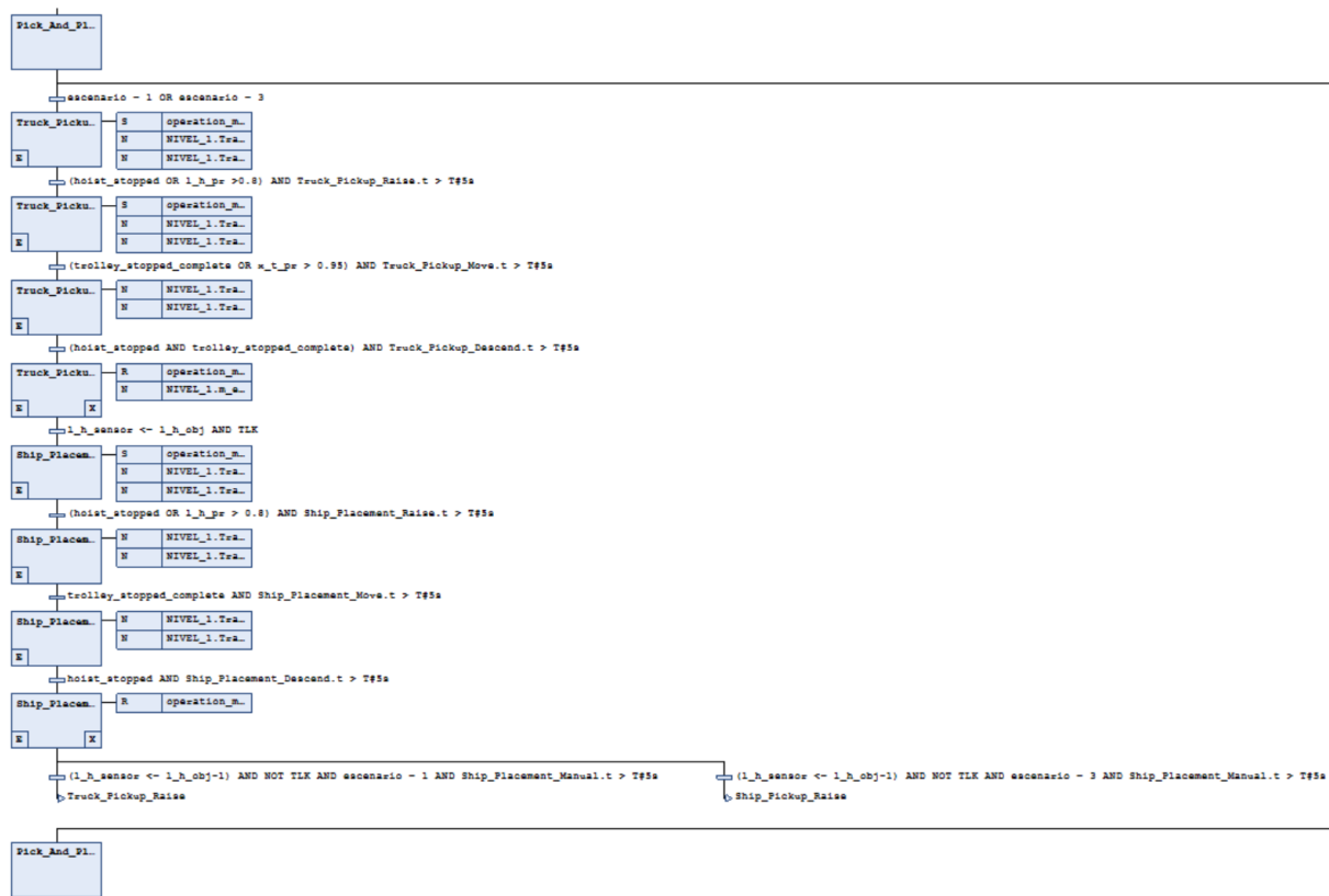
Figura 84: Recorrido de pasos para la operación de carga (camión → barco) dentro del macropaso Pick_And_Place_Loop.
