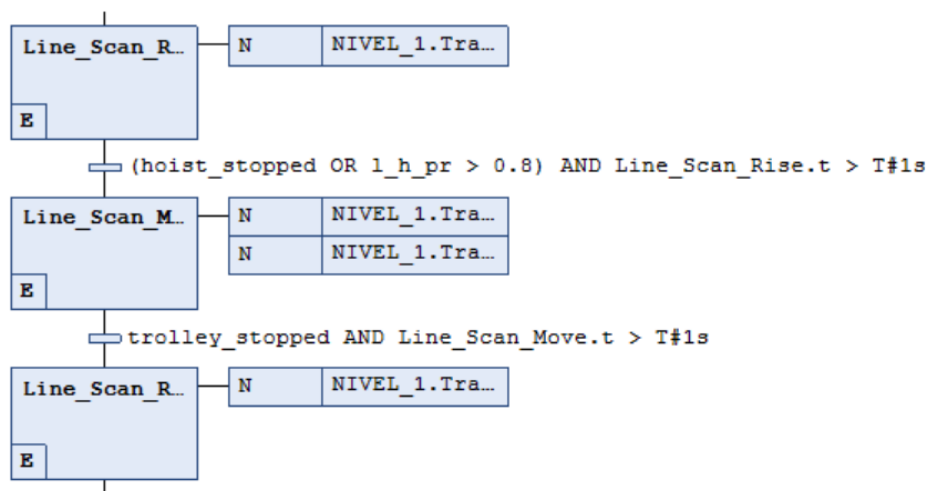
Figura 82: Pasos de inicialización del scan en el planificador de trayectorias de CODESYS: elevación, barrido derecha y barrido izquierda.
