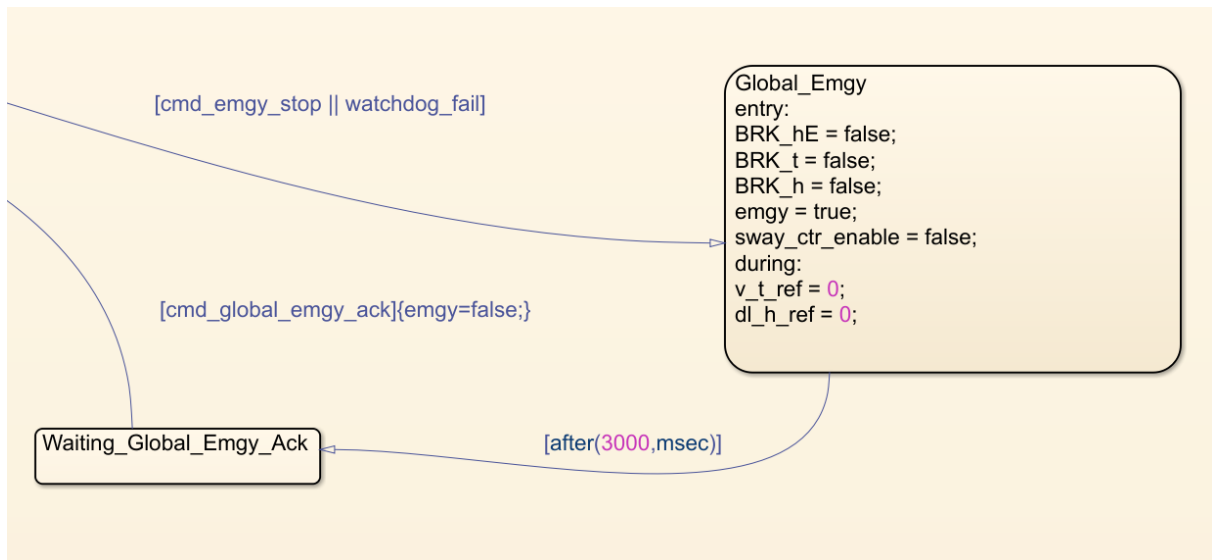
Figura 61: Subestado Global_Emg completo: acciones de entrada, espera de 3 s y reconocimiento del operador en Waiting_Global_Emg_Ack (Stateflow).
