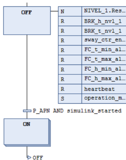
Figura 69: Macropaso Supervisory_Control del programa NIVEL_1. El step OFF inicializa las variables de control y alarma mediante acciones Reset/Set, y permanece activo hasta que se cumple P_APN AND simulink_started. El macropaso ON encapsula la lógica de operación normal y retorna incondicionalmente a OFF al finalizar.
