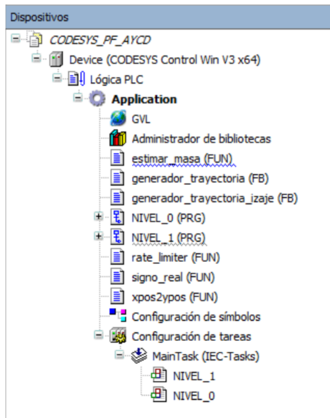
Figura 63: Árbol de proyecto CODESYS_PF_AYCD. Bajo Application se agrupan las variables globales (GVL), las funciones auxiliares ( estimar_masa , rate_limiter , signo_real , xpos2ypos ), los bloques de función de generación de trayectorias ( generador_trayectoria , generador_trayectoria_izaje ), y las POU tipo Programa NIVEL_0 y NIVEL_1 (cada una con acciones internas). La Configuración de símbolos habilita la interfaz OPC UA. En Configuración de tareas , MainTask ejecuta cíclicamente ambos programas.
