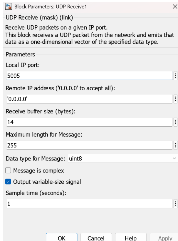
Figura 90: Configuración del bloque UDP Receive en Simulink: puerto 5005, buffer de 14 bytes, salida uint8 (Instrument Control Toolbox).
