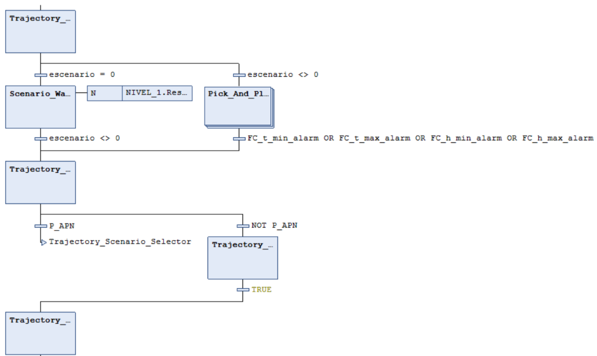
Figura 83: Lógica de selección de escenario y vía de escape del planificador de trayectorias en CODESYS (comportamiento descrito en la sección 3.3.9).
