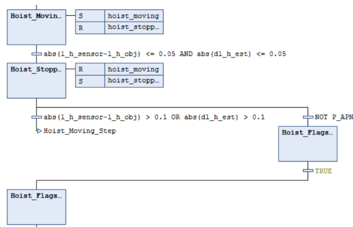
Figura 79: Macropaso Hoist_Movement_Flags en CODESYS (comportamiento descrito en la sección 3.3.8).
