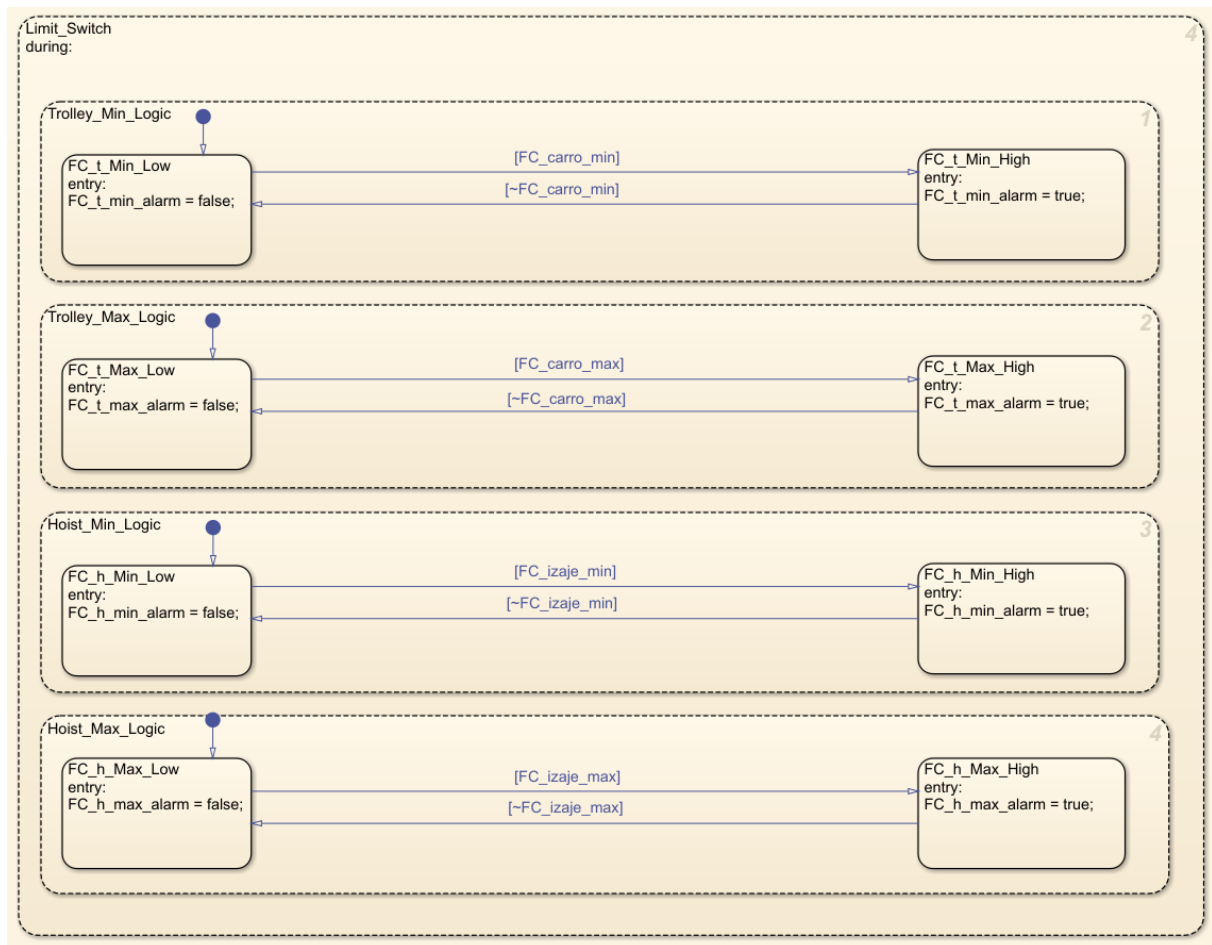
Figura 45: Subestado Limit_Switch: cuatro ramas paralelas de detección de fines de carrera.
