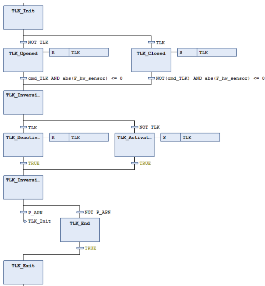
Figura 81: Macropaso TLK_Logic en CODESYS.
