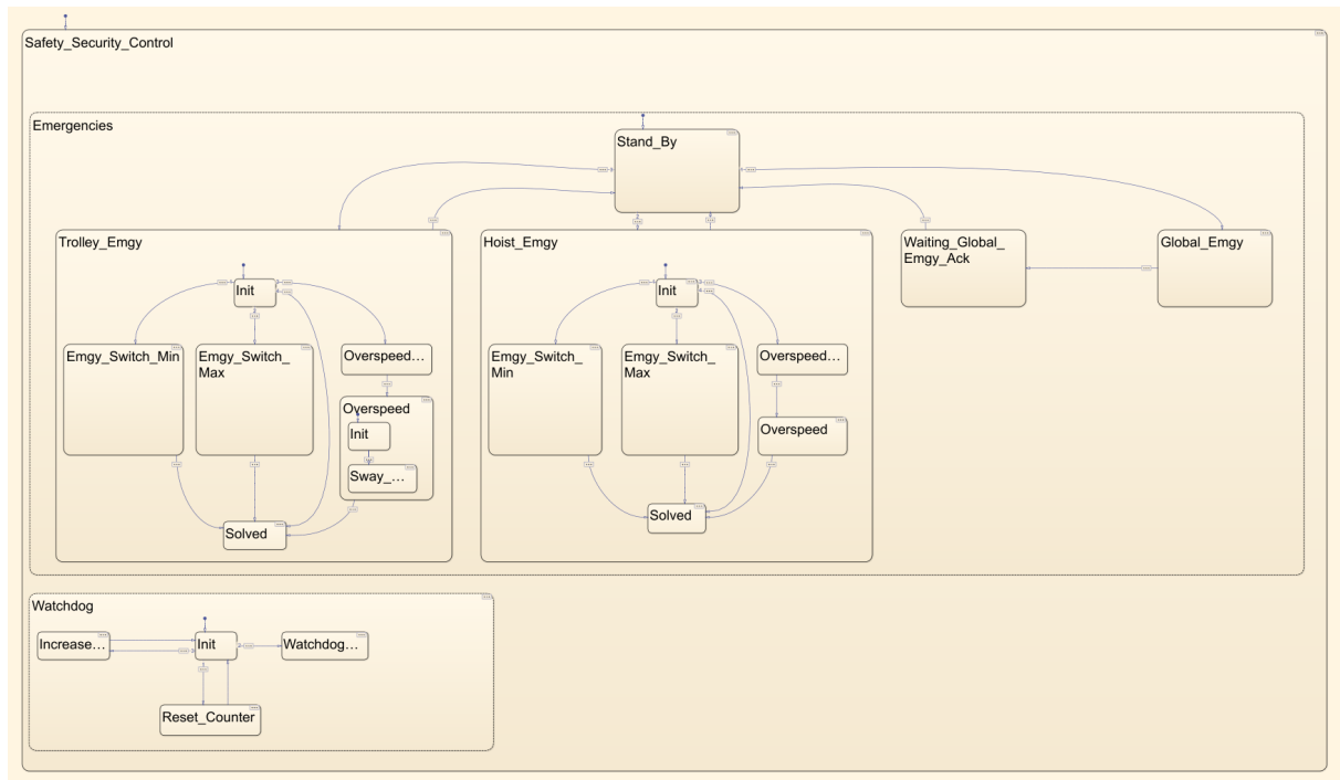
Figura 56: Diagrama de bloques del Nivel 0 completo: estados paralelos Emergencies y Watchdog (Stateflow, T_{s0} = 20 ms).
