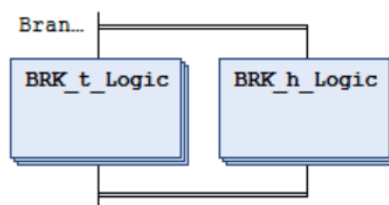
Figura 72: Macropaso BRK_Logic: rama AND que ejecuta en paralelo los macropasos BRK_t_Logic y BRK_h_Logic, uno por cada accionamiento.
