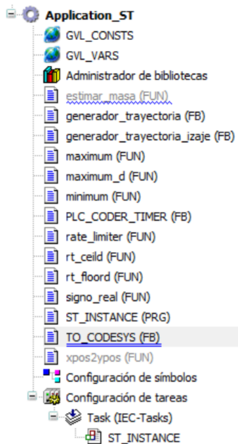
Figura 87: Estructura del proyecto CODESYS generado automáticamente mediante PLC Coder: Function Blocks , Programs , variables globales y bibliotecas auxiliares.
