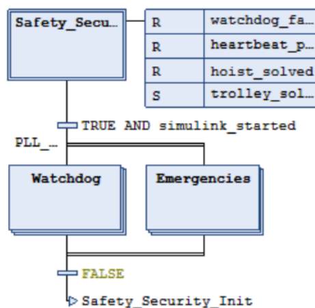
Figura 64: SFC del programa NIVEL_0 en CODESYS. El step inicial Safety_Security inicializa mediante acciones Reset/Set las variables de diagnóstico ( watchdog_failed , heartbeat_present , hoist_solved , trolley_solved ). La transición TRUE AND simulink_started habilita una rama AND que lanza en paralelo los pasos Watchdog y Emergencies , manteniendo ambas lógicas activas de forma concurrente durante toda la operación. Ante una condición FALSE , se ejecuta la acción Safety_Security_Init que reinicializa el nivel.
