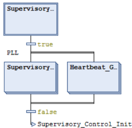
Figura 67: SFC del programa NIVEL_1 en CODESYS. El step inicial Supervisory_Control habilita, mediante transición true , una rama AND que activa en paralelo los macropasos Heartbeat_Generator y Supervisory_Control , los cuales permanecen activos de forma concurrente durante toda la operación. La rama OR con transición false y acción Supervisory_Control_Init provee el camino de salida requerido por IEC 61131-3 para conformidad del compilador.
