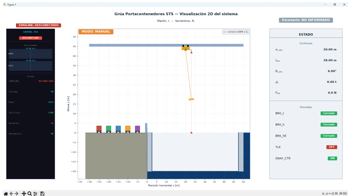
Figura 94: Visualización 2D en tiempo real de la grúa STS ( visualizacion_grua.py ): vista central con geometría animada, panel izquierdo de control PS4 y panel derecho de variables de estado (Python/matplotlib).
