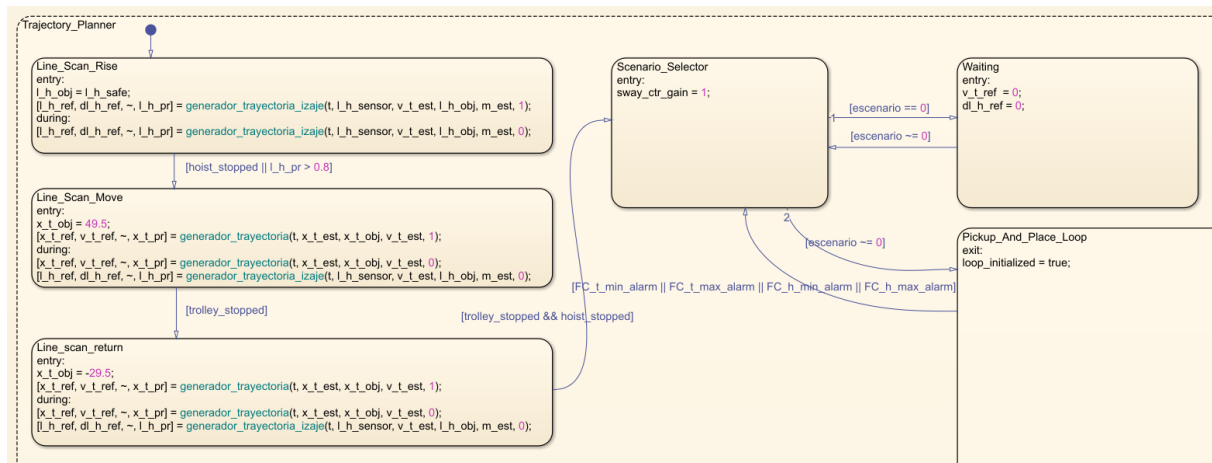
Figura 52: Estructura general del Trajectory_Planner: selección de escenario, escaneo LIDAR y retorno a homing .
