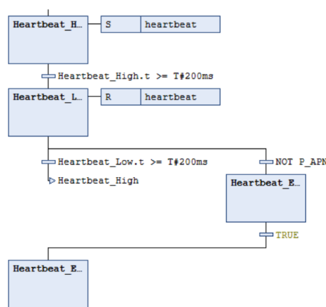
Figura 68: Macropaso Heartbeat_Generator del programa NIVEL_1, análogo al diseño de Stateflow de la sección 3.3.1. Al final se provee el camino de escape mencionado anteriormente, requerido por IEC 61131-3 para conformidad del compilador.
