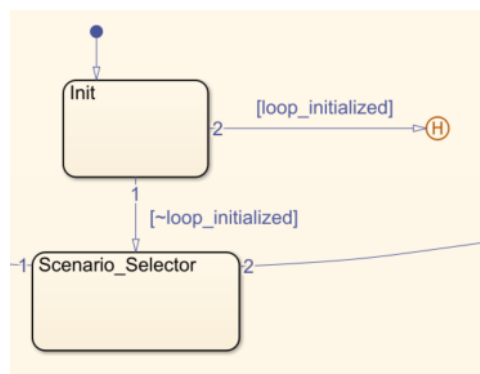
Figura 53: Lógica de Init dentro de Pickup_And_Place_Loop: reanudación por historia o inicialización según loop_initialized .
