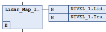
Figura 71: Macropaso Lidar_Map del programa NIVEL_1. Ejecuta las acciones LidarMapEntry (calificador N en el step de entrada E) y LidarMapDuring (calificador N en el step principal), análogas a las acciones entry y during del estado homónimo en Stateflow (sección 3.3.7), ambas implementadas en ST dentro de esta POU.
