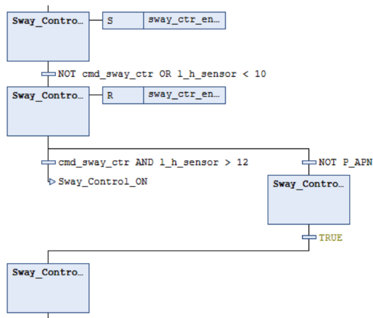
Figura 76: Macropaso Sway_Control_Mode en CODESYS.
