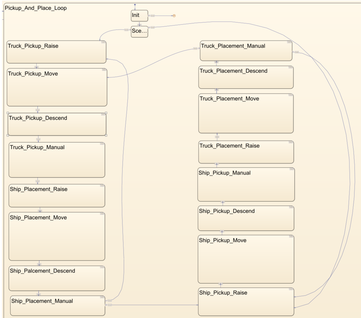
Figura 54: Estados del ciclo Pickup_And_Place_Loop.
