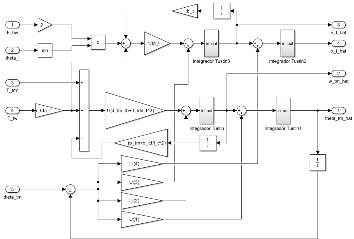
Figura 39: Observador de estados del carro implementado por bloques en Simulink ( T_{s2} = 1 \text{ ms} ), con las ganancias de retroalimentación \mathbf{L}_t .
