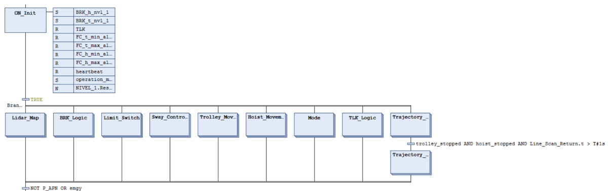
Figura 70: Interior del macropaso ON. Tras el step de inicialización ON_Init, una rama AND lanza en paralelo los macropasos Lidar_Map, BRK_Logic, Limit_Switch, Sway_Control, Trolley_Movement, Hoist_Movement, Mode, TLK_Logic y Trajectory, ejecutándose todos de forma concurrente. La rama AND finaliza con la transición NOT P_APN OR emgy, que retorna el control al step OFF.
