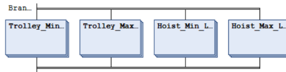
Figura 74: Macropaso Limit_Switch: rama AND con los macropasos Trolley_Min_LS, Trolley_Max_LS, Hoist_Min_LS y Hoist_Max_LS, uno por cada fin de carrera supervisado.
