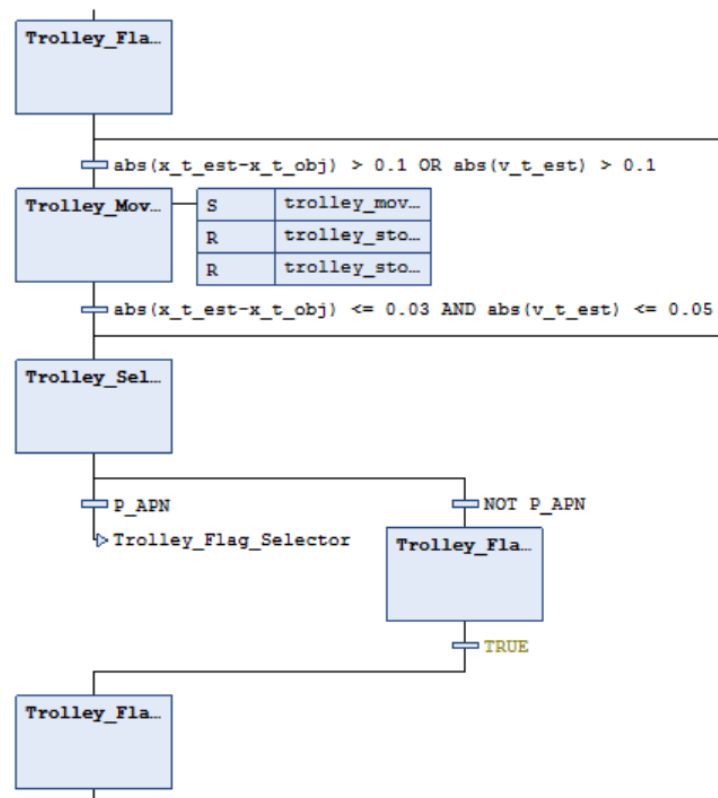
Figura 77: Macropaso Trolley_Movement_Flags en CODESYS: primer elemento de la rama OR (comportamiento descrito en la sección 3.3.8).
