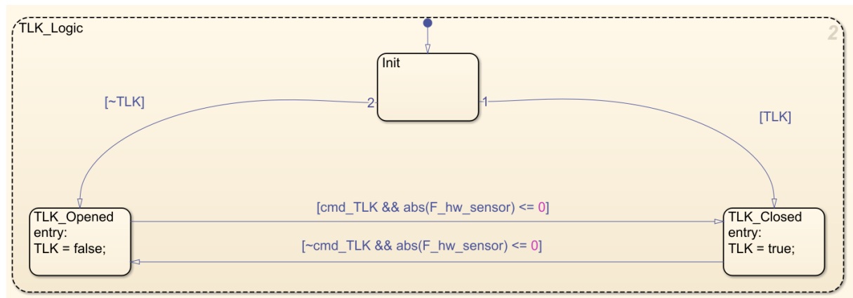
Figura 47: Subestado TLK_Logic: lógica de apertura y cierre de twistlocks con condición de seguridad sobre la fuerza en cable.
