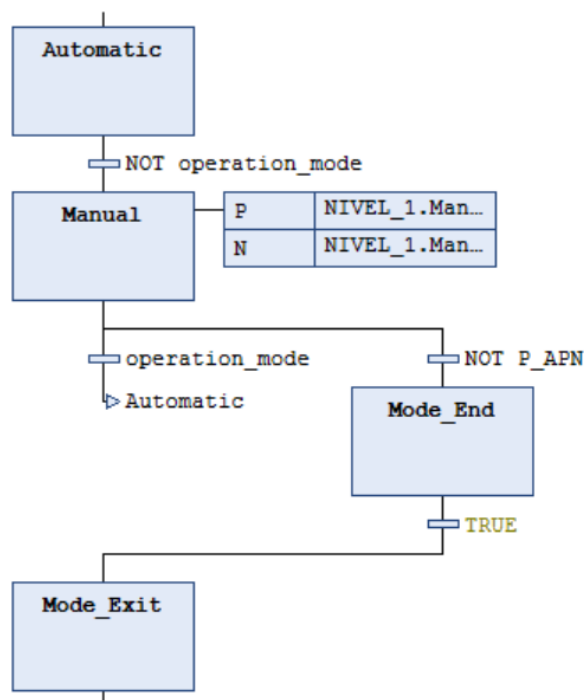
Figura 80: Macropaso Mode en CODESYS.
