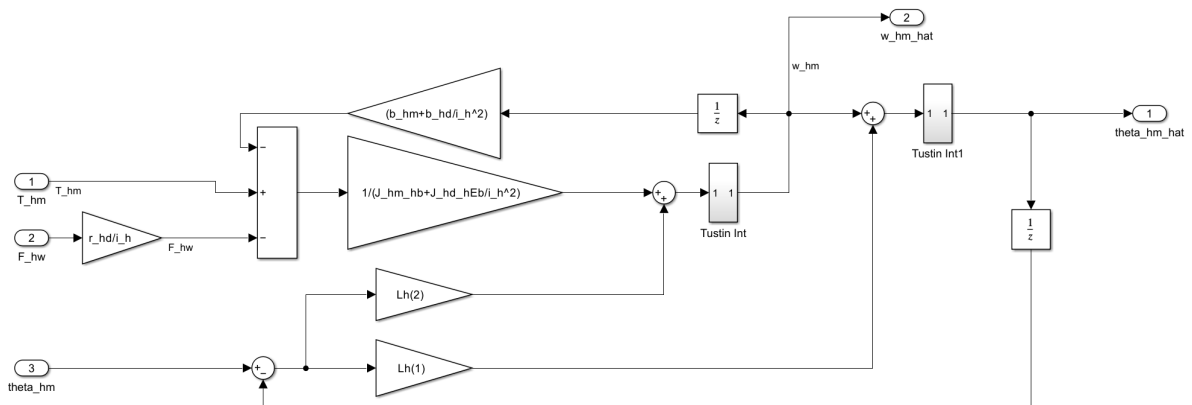
Figura 32: Diagrama de bloques del observador de estados del izaje discretizado (Simulink, T_{s2} = 1 ms).
