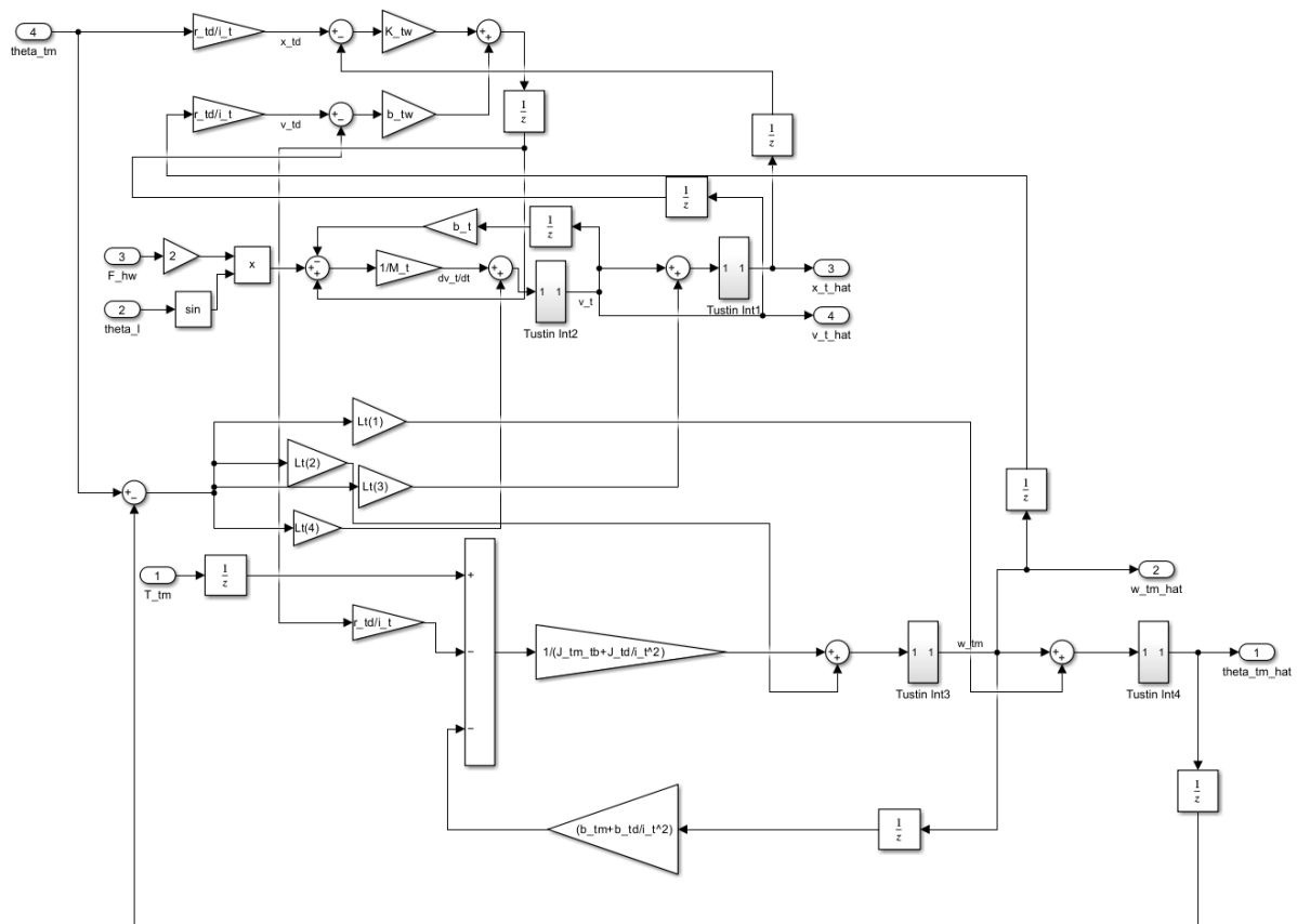
Figura 27: Diagrama de bloques del observador de estados del carro discretizado (Simulink, T_{s2} = 1 ms).
