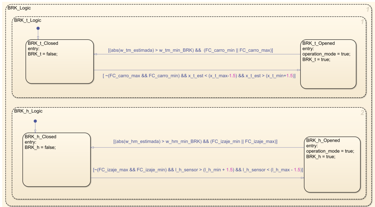
Figura 42: Lógica de frenos: subestados paralelos BRK_t_Logic y BRK_h_Logic.
