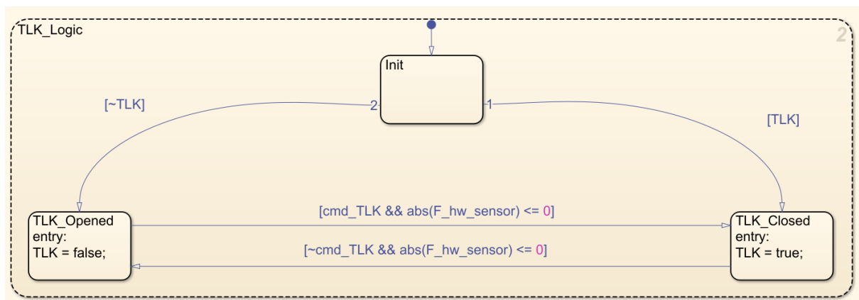
Figura 45: Subestado TLK_Logic: lógica de apertura y cierre de twistlocks con condición de seguridad sobre la fuerza en cable.
