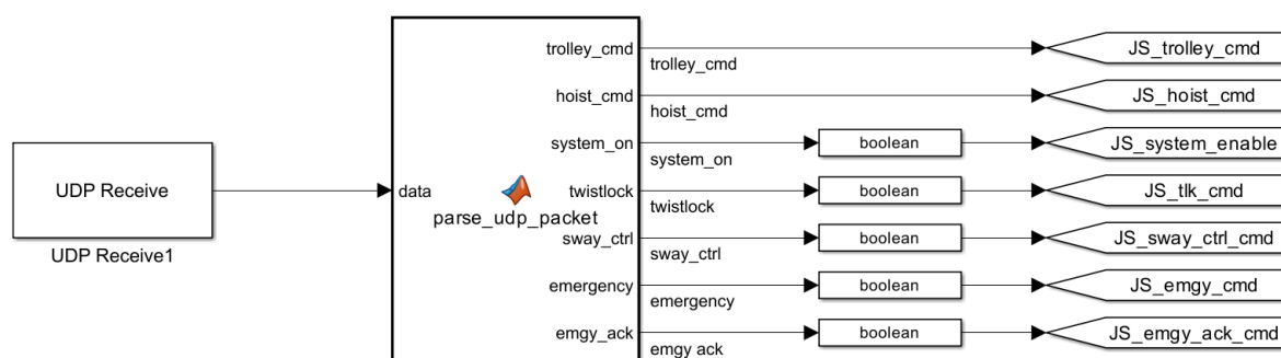
Figura 64: Bloque de lectura UDP completo en Simulink: UDP Receive y MATLAB Function parse_udp_packet con sus siete salidas hacia el sistema de control.
