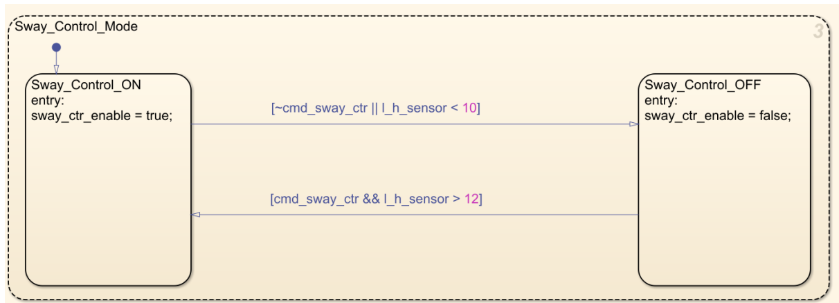
Figura 46: Subestado Sway_Control_Mode : habilitación del controlador de balanceo con condición de longitud mínima de cable.
