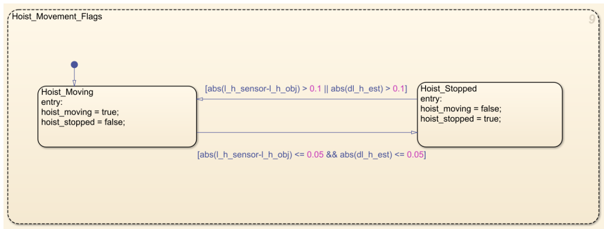
Figura 49: Subestado Hoist_Movement_Flags : detección de izaje detenido.
