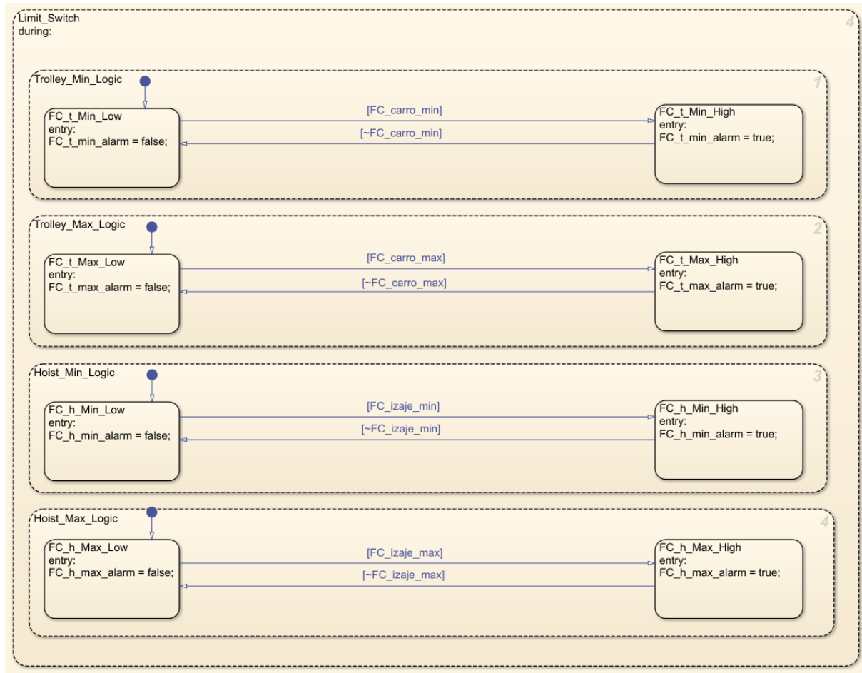
Figura 43: Subestado Limit_Switch : cuatro ramas paralelas de detección de fines de carrera.
