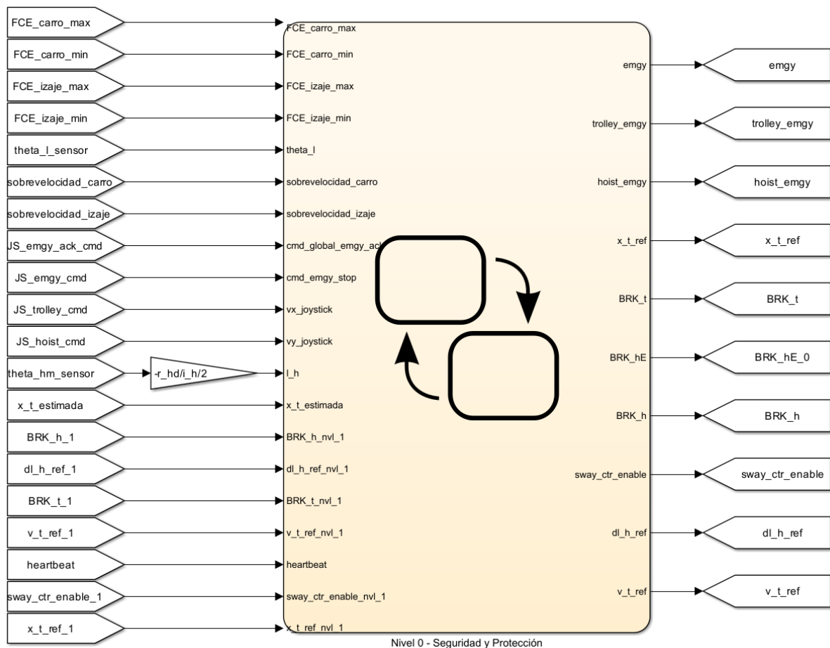
Figura 53: Nivel 0 visto desde el exterior: entradas y salidas del autómata de seguridad y protección (Stateflow).
