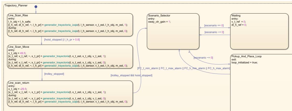
Figura 50: Estructura general del Trajectory_Planner: selección de escenario, escaneo LIDAR y retorno a homing .
