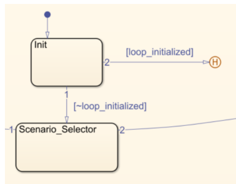
Figura 51: Lógica de Init dentro de Pickup_And_Place_Loop: reanudación por historia o inicialización según loop_initialized .
