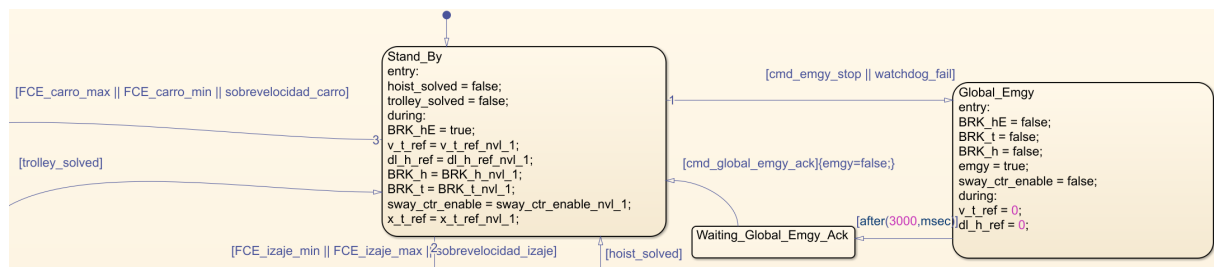
Figura 55: Estado Emergencies: estado de entrada Stand_By (Stateflow).
