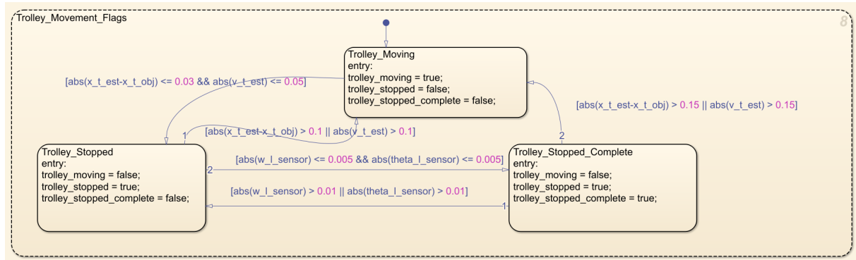
Figura 48: Subestado Trolley_Movement_Flags : detección de carro detenido con condición de balanceo amortiguado.
