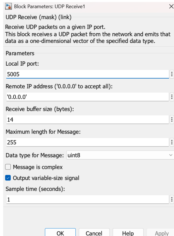
Figura 63: Configuración del bloque UDP Receive en Simulink: puerto 5005, buffer de 14 bytes, salida uint8 (Instrument Control Toolbox).
