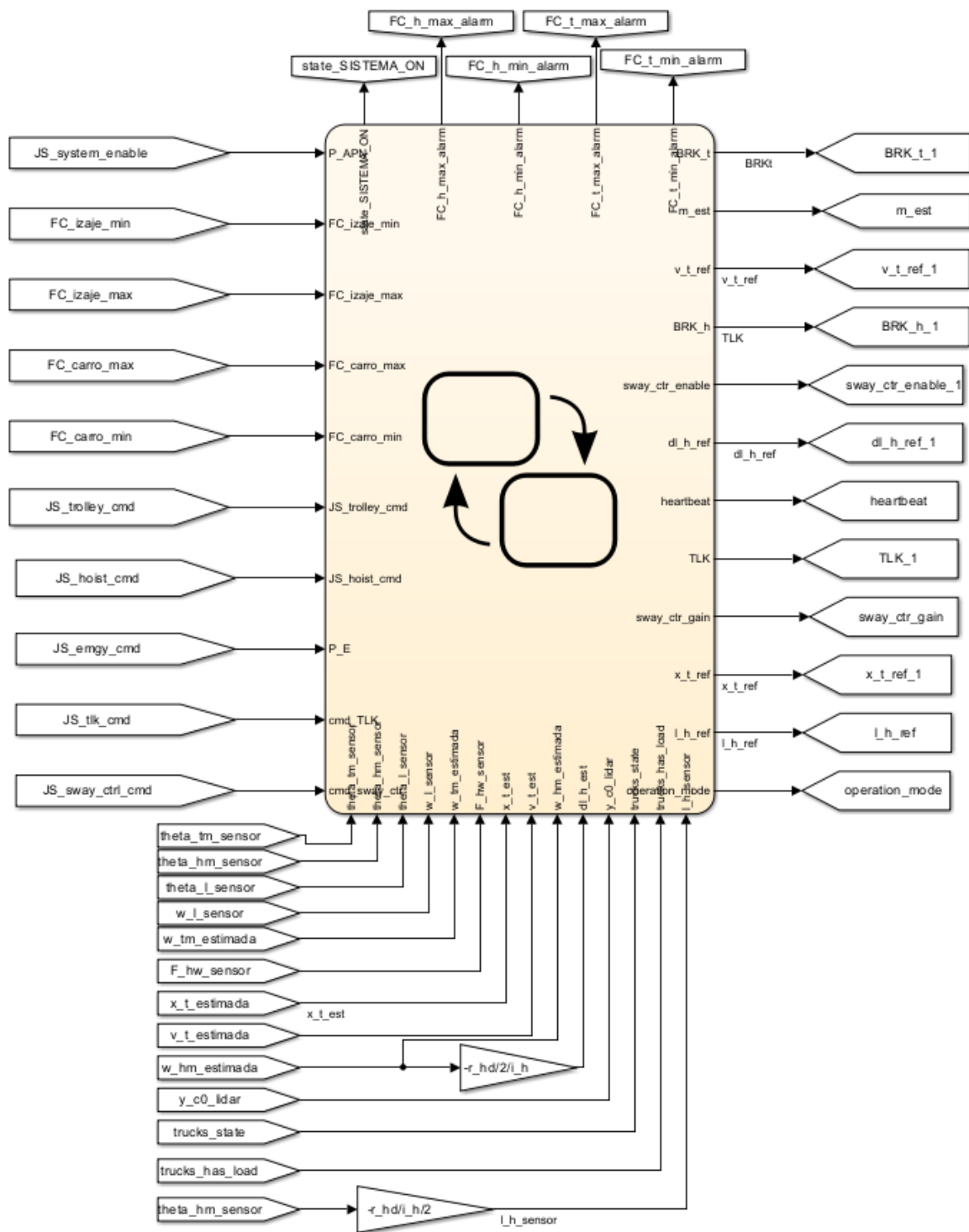
Figura 40: Esquema de entradas y salidas del Nivel 1.
