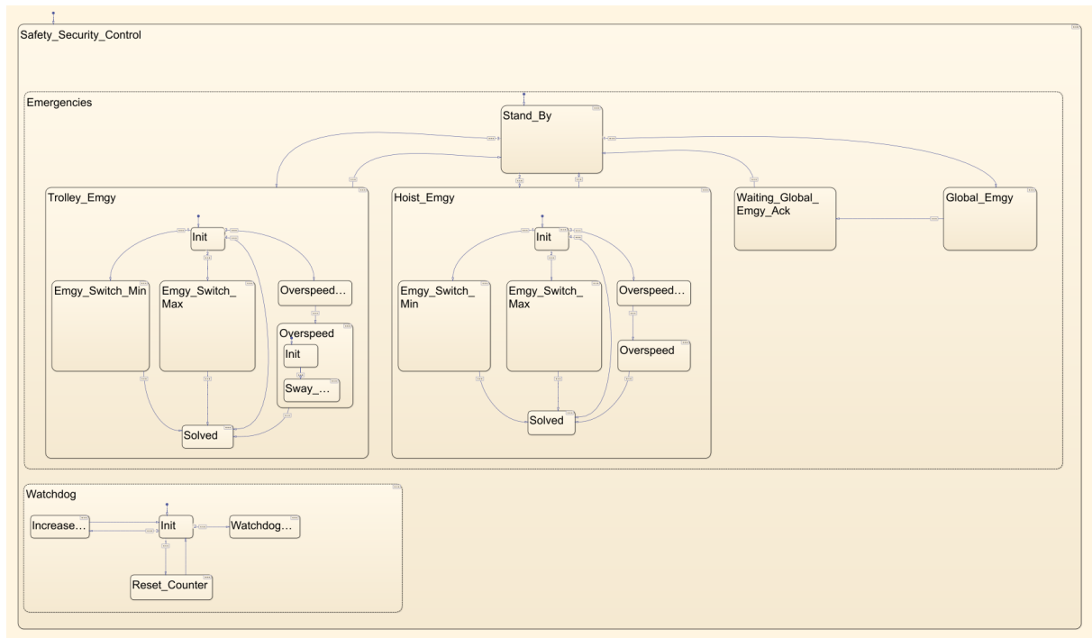
Figura 54: Diagrama de bloques del Nivel 0 completo: estados paralelos Emergencies y Watchdog (Stateflow, T_{s0} = 20 ms).
