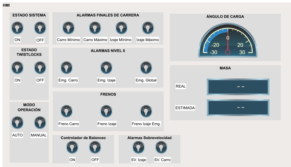
Figura 68: Panel de monitoreo del sistema desarrollado con la librería Dashboard de Simulink.
