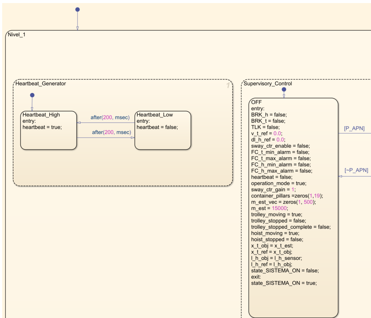
Figura 41: Estructura paralela del Nivel 1: Heartbeat_Generator y estado OFF de Supervisory_Control .
