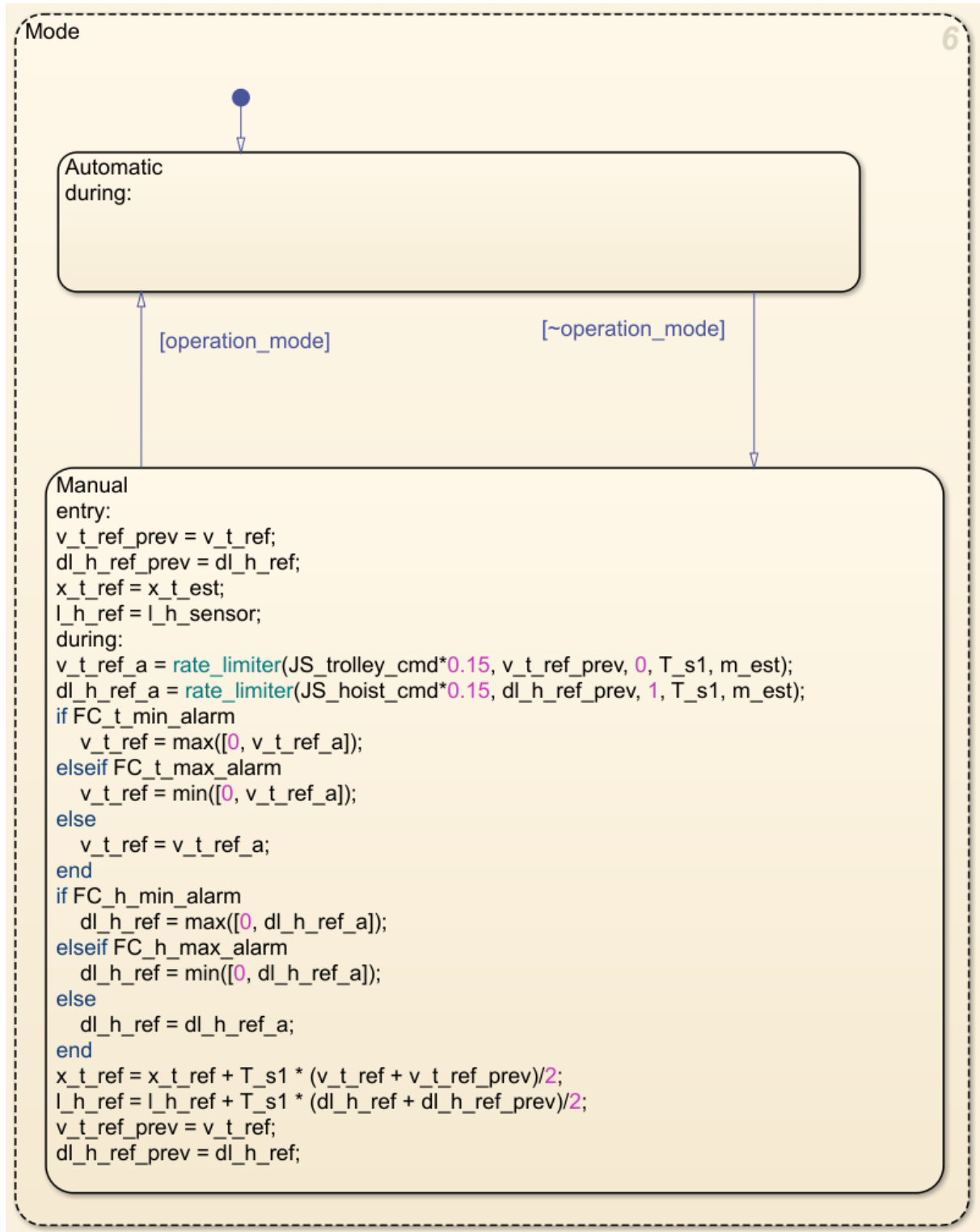
Figura 44: Subestado Mode: lógica de conmutación entre operación manual y automática.
