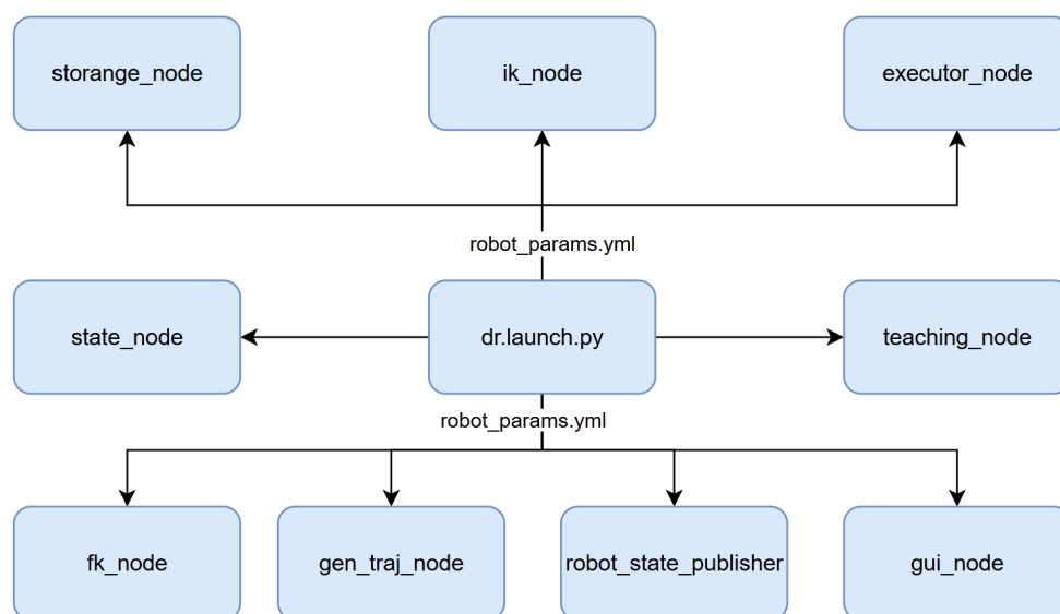
Figura 33: Esquema de levantamiento de nodos desde nodo launcher.
