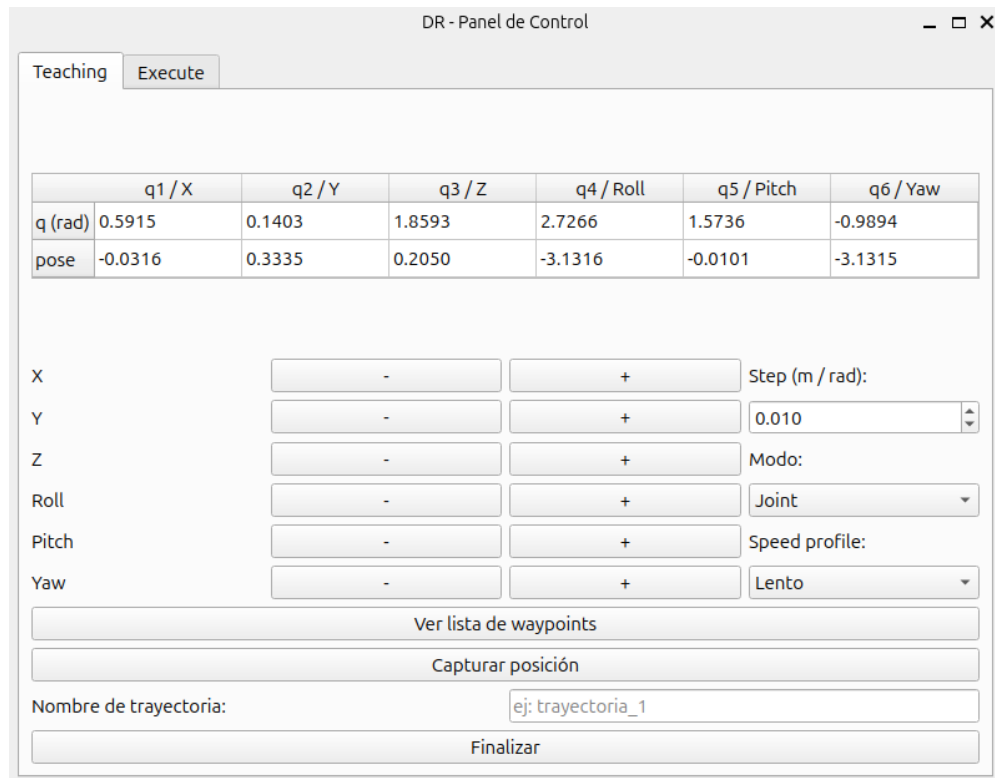
Figura 35: Interfaz gráfica de usuario en ROS 2 - Pestaña de teaching.
