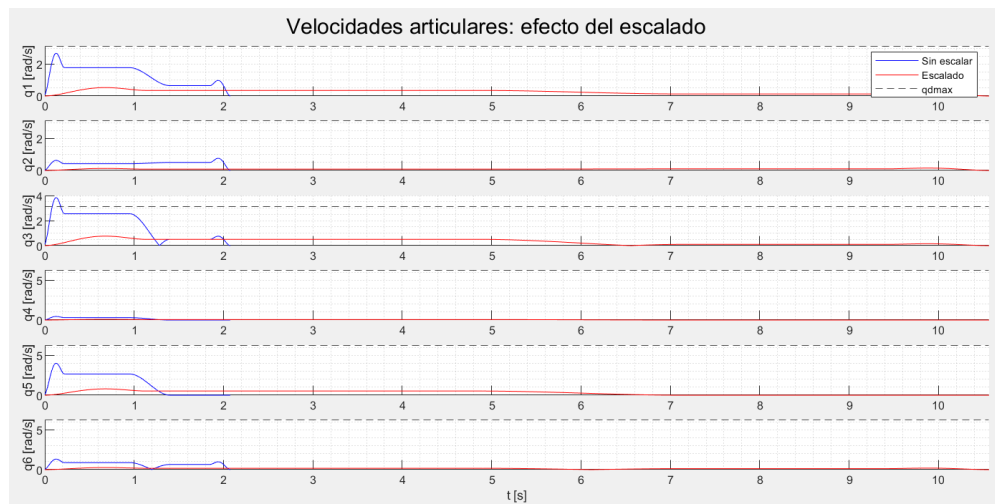
Figura 40: Comparativa entre perfiles de velocidad articular antes y después del escalado para cumplimiento de límites.
