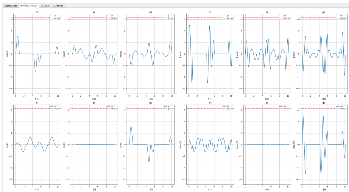
Figura 37: Evolución de velocidades y aceleraciones articulares durante el ciclo.
