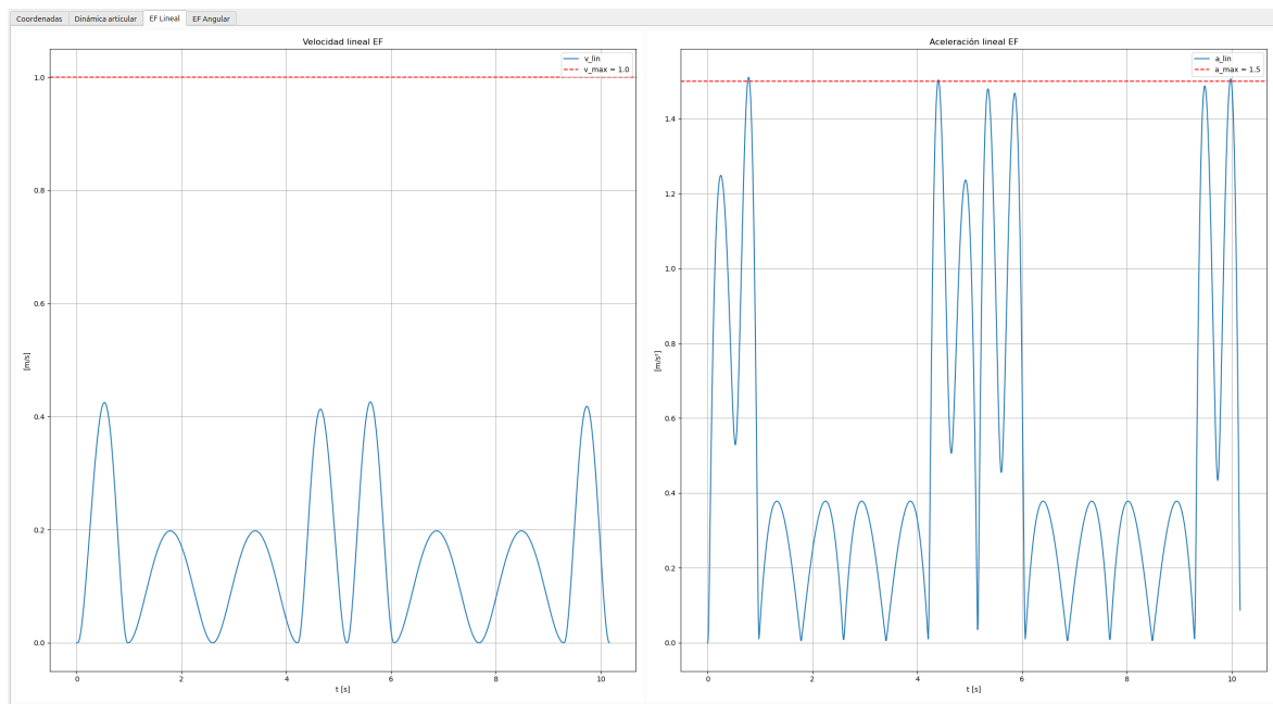
Figura 38: Evolución de velocidad y aceleración lineales del efector final durante el ciclo.
