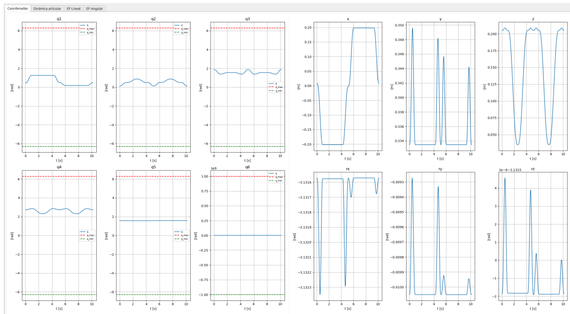
Figura 36: Evolución de posiciones articulares y coordenadas cartesianas del efector final durante el ciclo.
