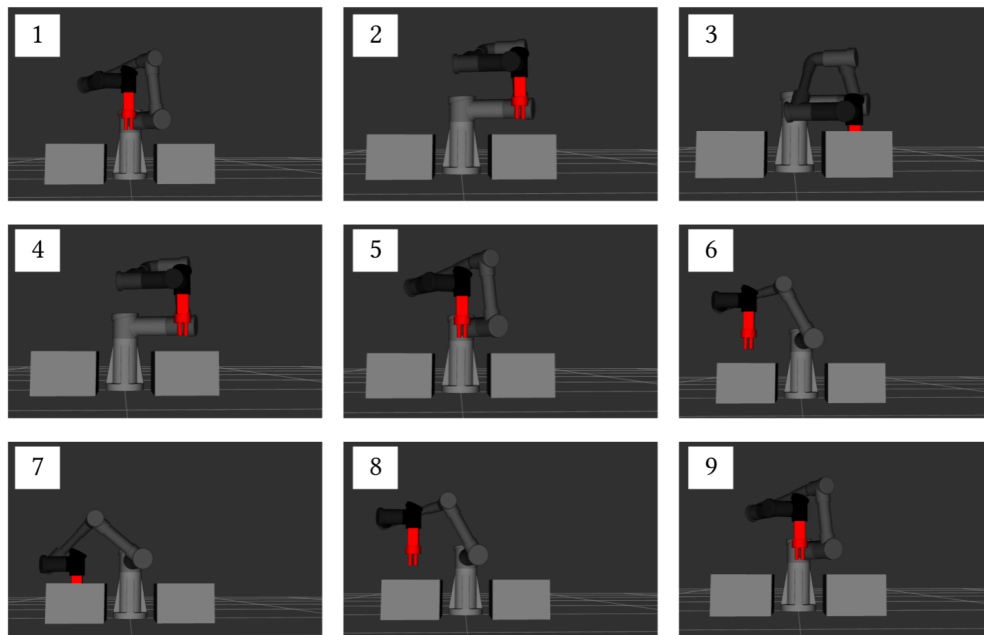
Figura 34: Nueve posturas del robot correspondientes a un ciclo completo de la tarea.
