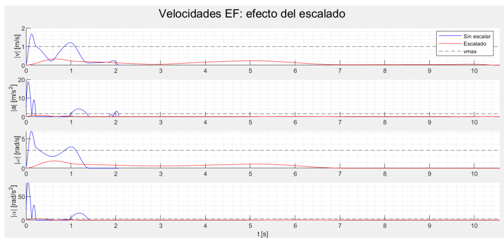
Figura 41: Comparativa entre perfiles de velocidad cartesiana del efector final antes y después del escalado para cumplimiento de límites.
