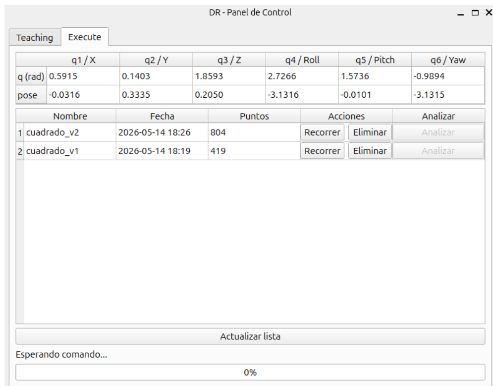
Figura 29: Interfáz gráfica de usuario en ROS 2 - Pestaña de ejecución.
