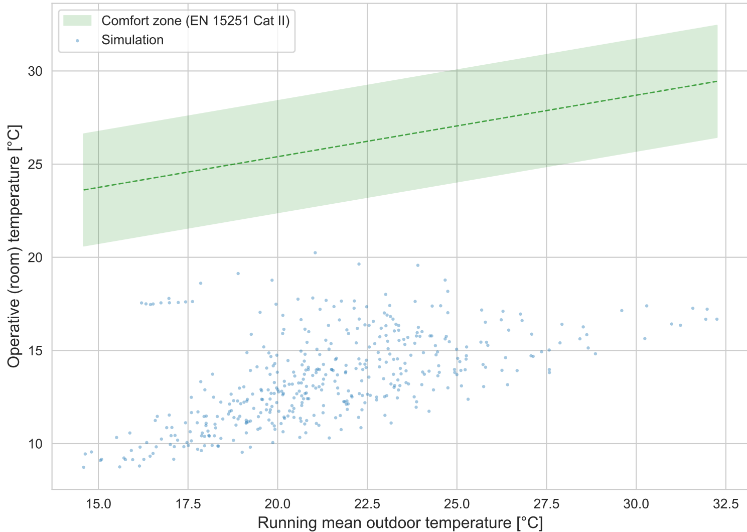
Adaptive Comfort Map — EN 15251
