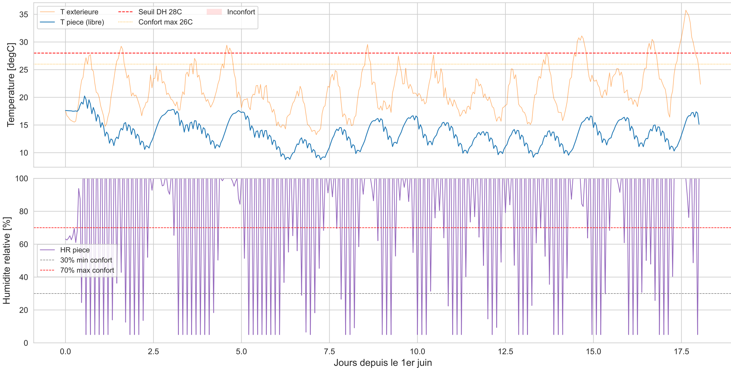
Beton de chanvre 30 cm — Simulation libre juin-juillet (Macon +2C) T max ext=36.6C T max piece=nanC Attenuation=nanC DH=nan degC.h
