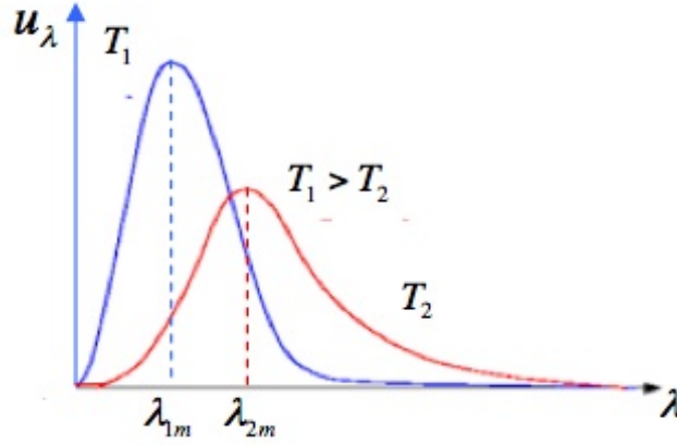
Figura 4: Radiación espectral u_\lambda de un cuerpo negro
