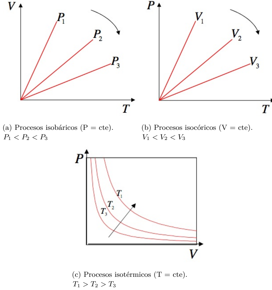
Figura 1: Procesos reversibles de un gas ideal.
