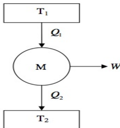
Figura 3: El sistema que realiza el ciclo reversible o irreversible (círculo) absorbe calor Q_1 de la fuente a T_1 , cede calor Q_2 a la fuente más fría a T_2 y entrega trabajo W .
