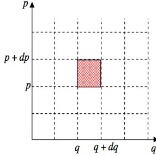
Figura 4: Espacio de fases de una partícula.
