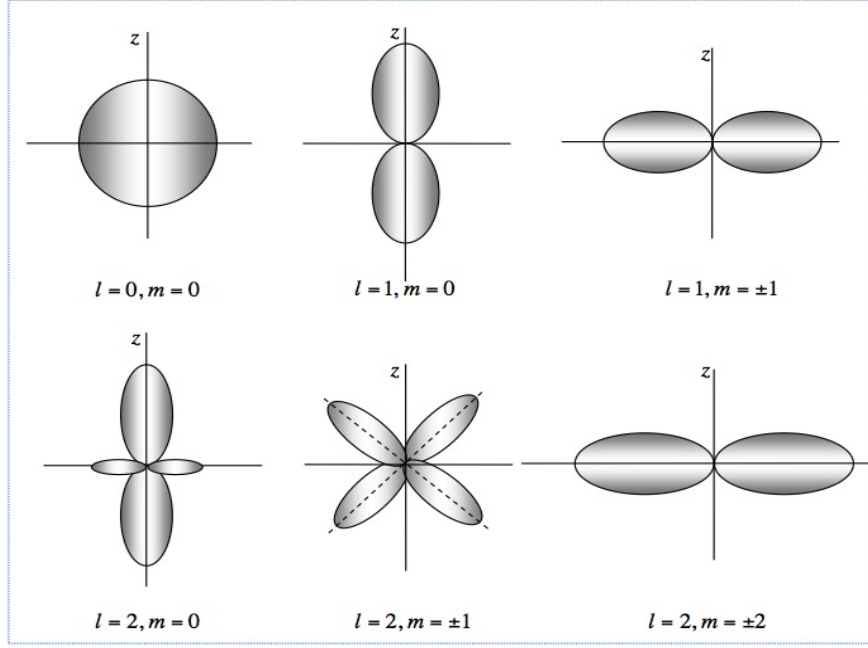
Figura 8: Armónicos esféricos Y_{lm}(\theta, \phi) para l = 0, 1, 2 y m = 0, \pm 1, \pm 2 .
