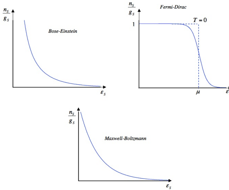
Figura 9: Forma funcional de las estadísticas MB, FD y BE.
