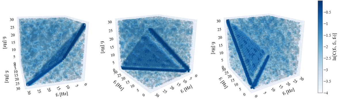
Figura 4.15: Distintas vistas de la correlación C(f_1, f_2, f_3) en escala logarítmica para la señal de 0-6 Hz y amplitud del 100%.
