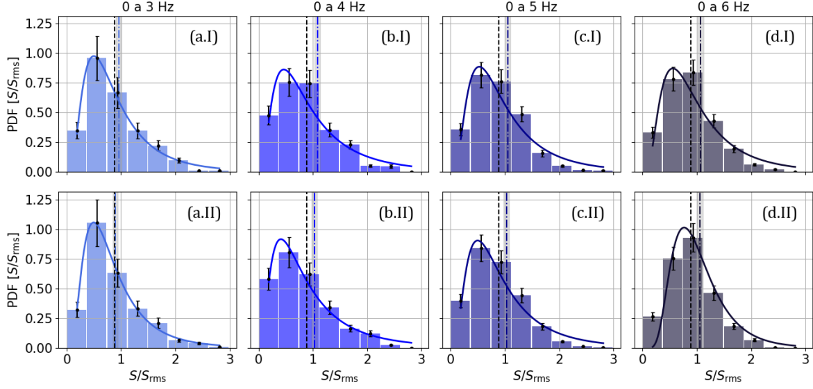
Figura 4.8: PDFs para la pendiente de las ondas normalizada ( S/S_{rms} ) de varias mediciones. Cada columna se corresponde a un rango de frecuencias, siendo (a) 0-3 Hz (b) 0-4 Hz (c) 0-5 Hz y (d) 0-6 Hz. La fila superior (n.I) se corresponde a la amplitud de 80 % y la inferior (n.II) a 120 %. Para cada una se muestra el ajuste por el modelo log-normal (—), el valor medio obtenido (---) con su incerteza y el valor teórico esperado de \sqrt{\pi}/2 (---).
