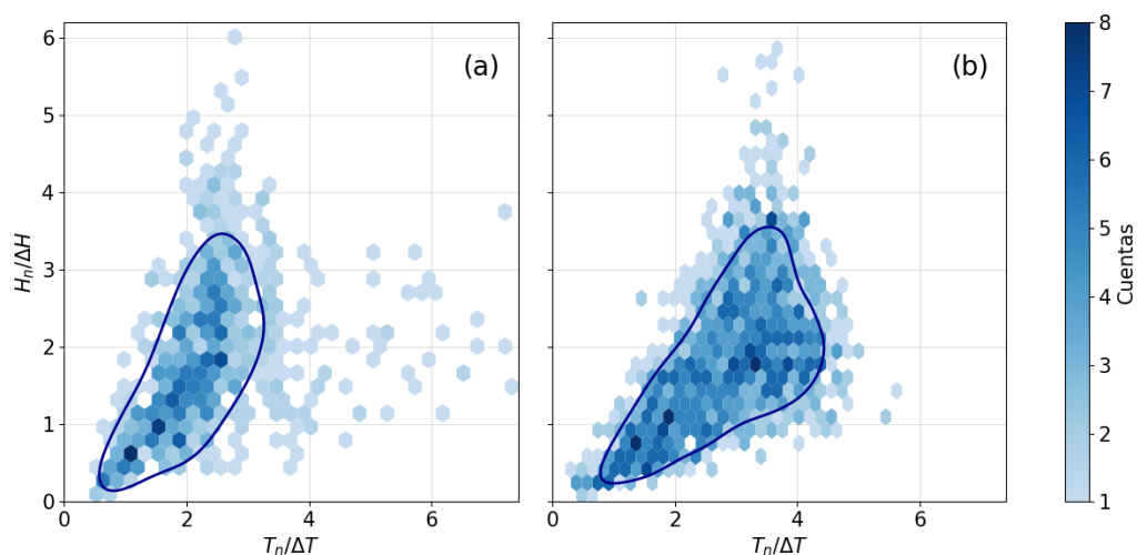
Figura 4.6: Histograma 2D de bins hexagonales para el conjunto de puntos (T_n, H_n) normalizados por la desviación estándar en los casos de (a) la medición correspondiente al forzado de 0-6 Hz y 150 % de amplitud, y (b) las mediciones en el océano reportadas por Tayfun (2006) [36]. La línea sólida superpuesta (—) representa en ambos casos el contorno que contiene al 67% de los puntos.
