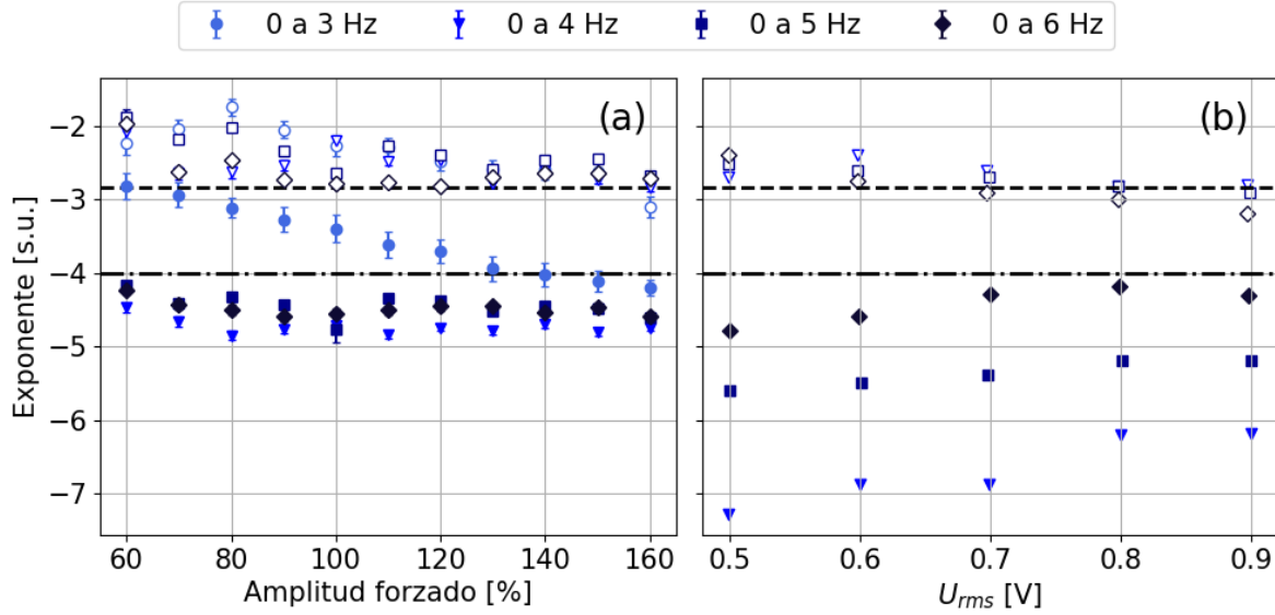
Figura 4.13: (a) Exponentes de la PSD obtenidos para ambos regímenes de la cascada de energía. En símbolos llenos (●) para el gravitatorio y en símbolos vacíos (○) para el capilar. Las líneas horizontales muestran la predicción teórica para los espectros de ZE, de -4 en gravedad (— · — · —) y -17/6 en capilar (— — —). (b) Resultados de la literatura para un experimento análogo en mercurio [38].
