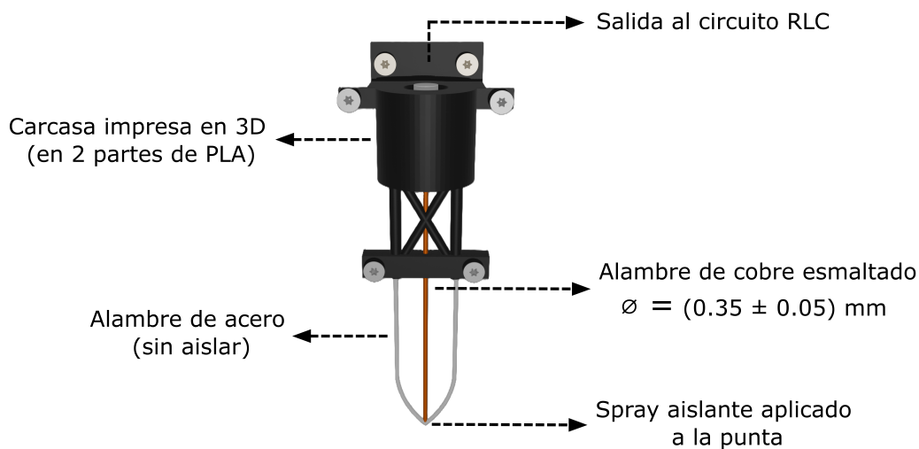
Figura 3.9: Modelo 3D de la sonda construida. El componente principal es el alambre de cobre esmaltado de (0.35 \pm 0.05) mm de diámetro. El soporte estructural consta de una carcasa impresa en PLA y un alambre de acero sin esmaltar que cumple la función adicional de conectar el agua a Tierra.
