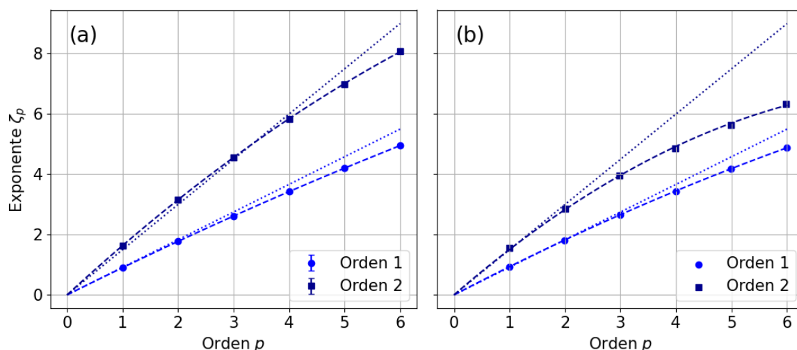
Figura 4.22: Exponentes \zeta_p obtenidos para las funciones de estructura S_p en el rango capilar (●) calculadas con las diferencias de orden uno y dos. (a) Este trabajo. (b) Falcon (2007) [37]. Se muestran además los ajustes realizados (---) por una función cuadrática \zeta_p = c_1 p - c_2 p^2/2 , cuyos resultados se encuentran en la Tabla 4.2, y el escalado esperado por análisis dimensional (.....).
