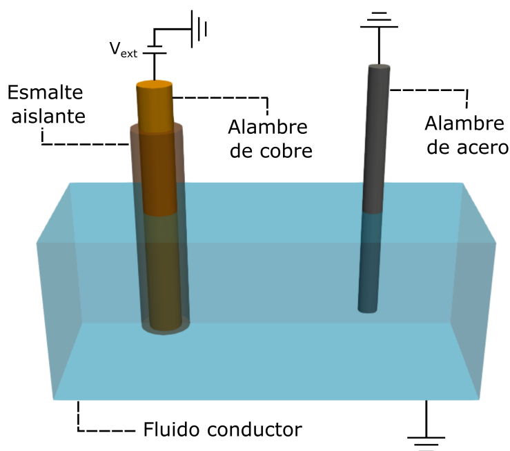
Figura 3.2: Esquema de un alambre esmaltado sumergido en un fluido conductor, puesto a Tierra mediante otro alambre sin aislar. El alambre de cobre se encuentra a conectado a un potencial externo V_{ext} . El recubrimiento aislante actuará como medio dieléctrico, comportándose el sistema efectivamente como un capacitor, cuya capacitancia depende de la altura sumergida.
